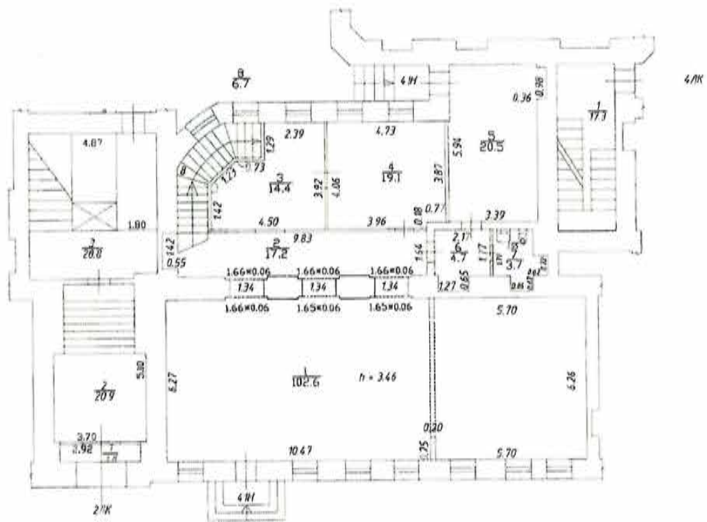
План части 1 этажа
