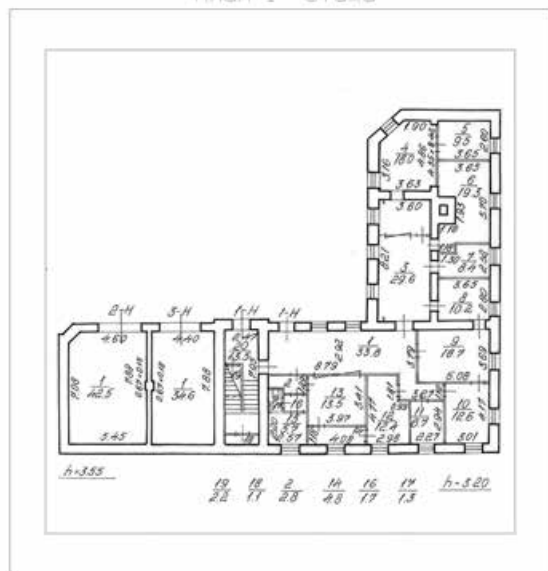
План 1 этажа
