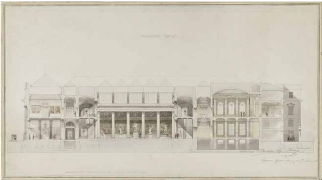
30. Проект выставочного корпуса Императорской Академии художеств. Продольный разрез. Архитектор Л. Бенуа. 1914 г. Государственной Русский музей (инв. № Аф ВХ 483).
