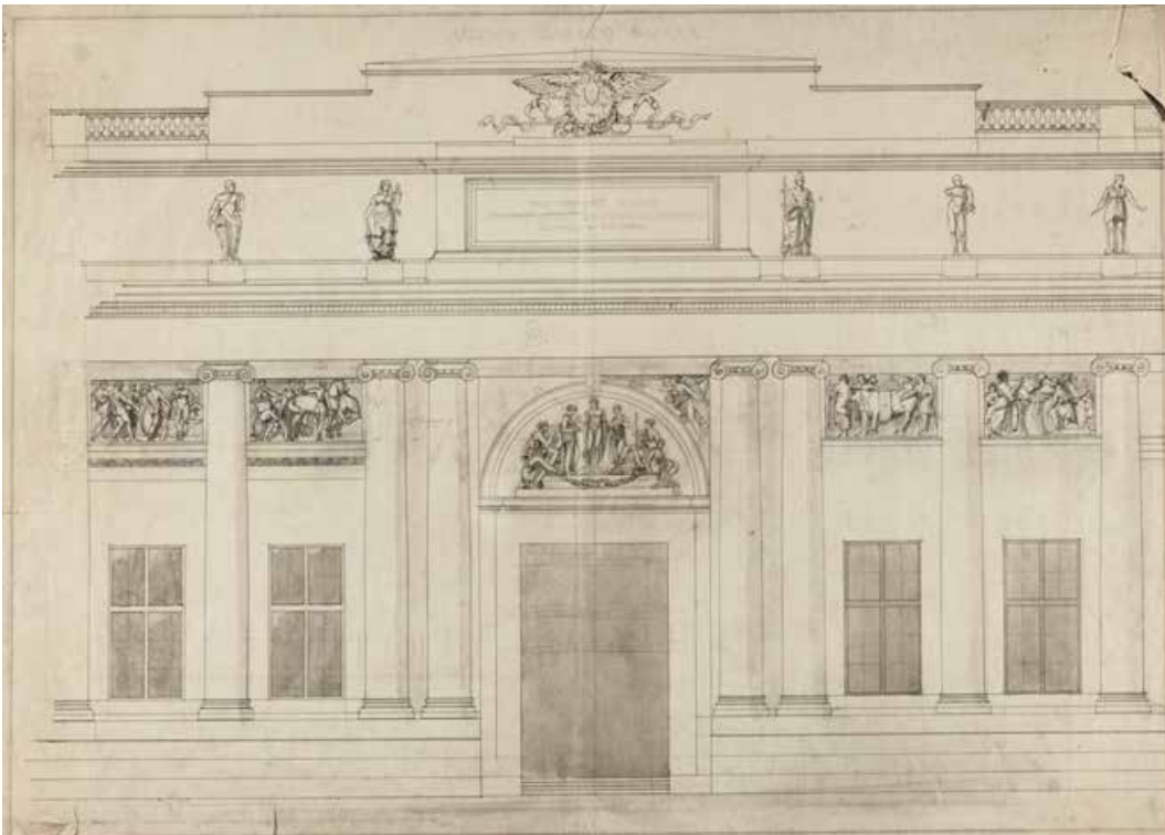
27. Проект выставочного корпуса Императорской Академии художеств. Фасад со стороны Екатерининского канала. Архитектор Л. Бенуа. 1914 г. Деталь главного входа. Государственной Русский музей (инв. № Аф ВХ 484).
