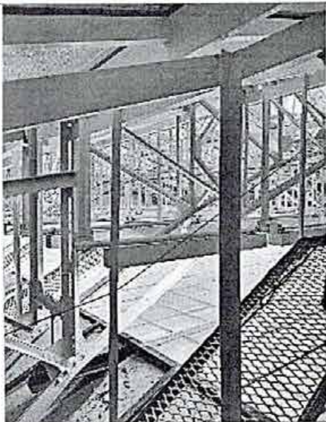
Фото 14. Фрагмент конструкций светового фонаря
