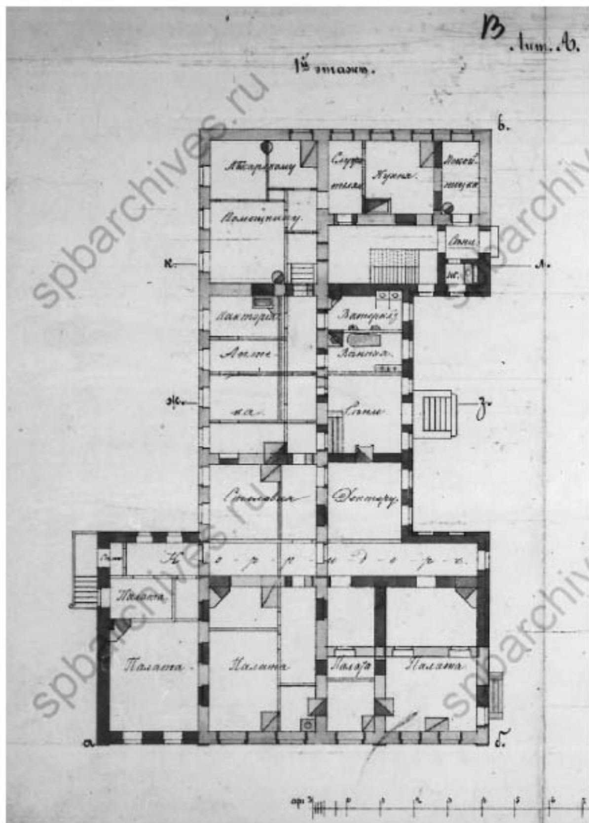
18. Духовная Академия лит. А, план 1-го этажа, 1879 г. (ЦГИА СПб Ф.513. Оп. 102. Д. 760)
