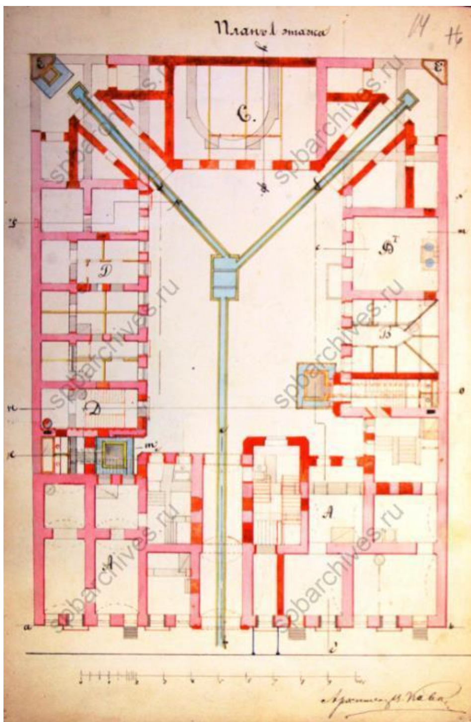
8. Проектный чертеж 1-го этажа. 1871 г. ЦГИА СПб. Ф.513. Оп.102. Д.3459. Л.14.
