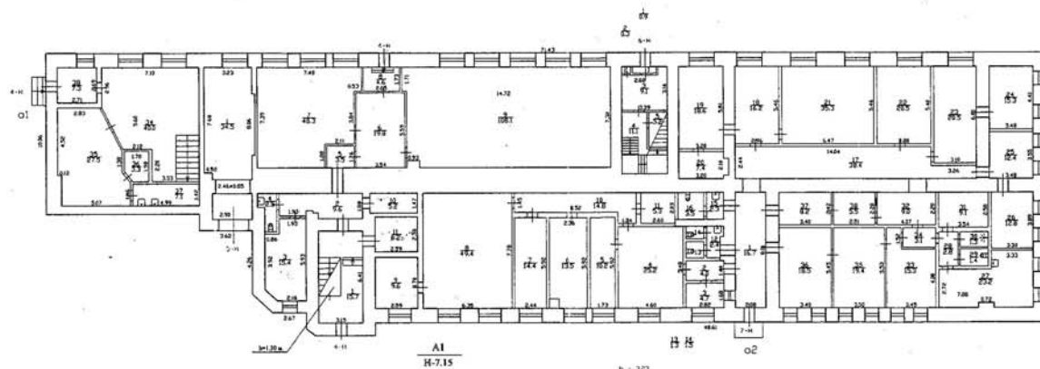
Литера А План 1 этажа
