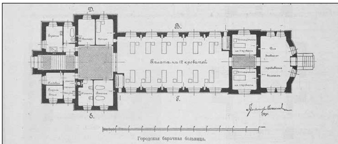
5. Александровская городская барачная больница им. С.П. Боткина. Каменный лечебный павильон 14 кроватей. Арх. А.Д. Шиллинг, под руководством И.С. Китнера и главного врача С.В. Посадского. План 1-го этажа. 1910 г.
