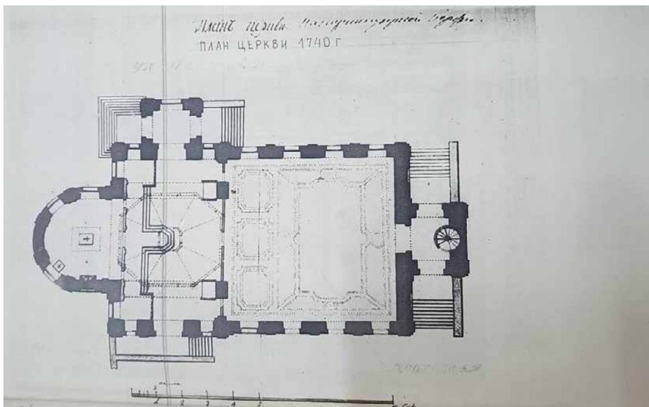
10. План церкви Св. Пантелеймона, 1740 г. ЦГАНТД СПб Ф.488. Оп.3-24. Д.713
