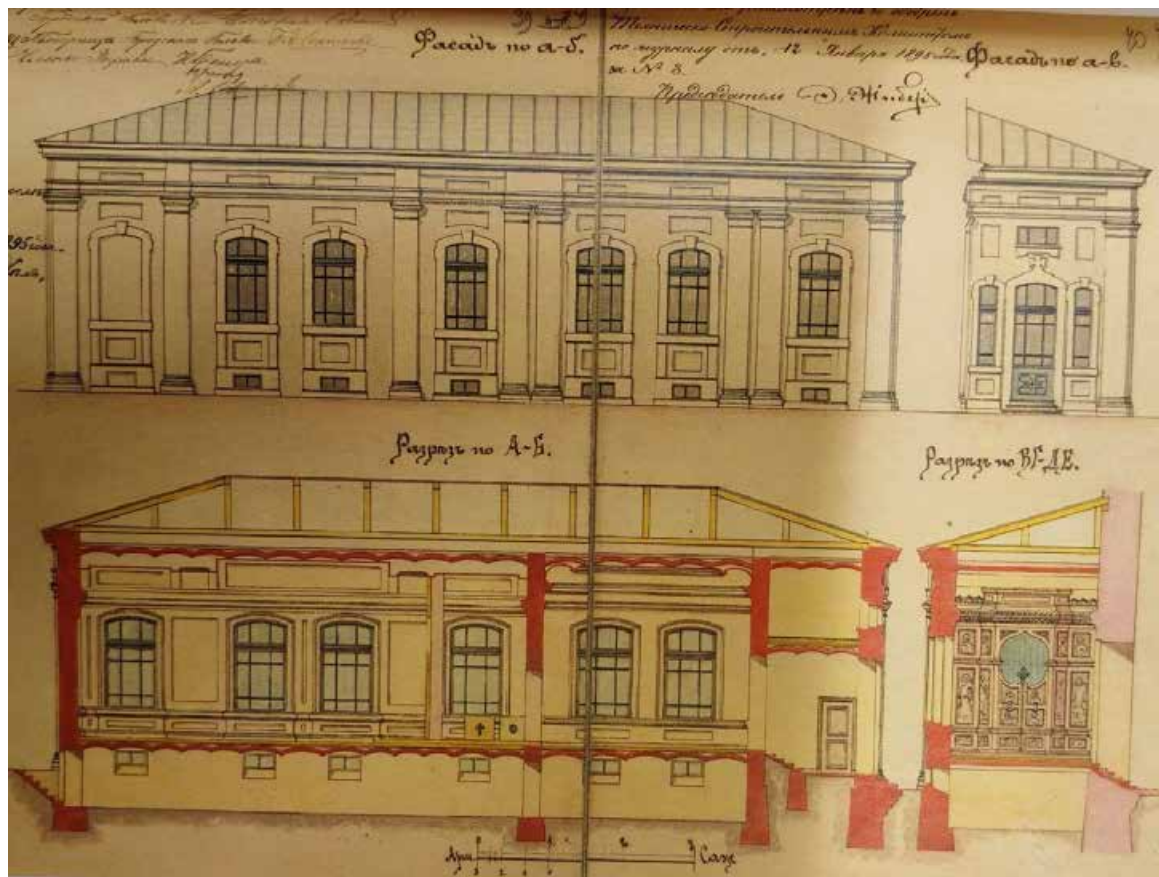
18. Церковь Св. Пантелеимона. Проект северной пристройки. Фасады. Арх. И.В. Гольмдорф. 1895 г. ЦГИА СПб. Ф.513, оп. 102, д.4338
