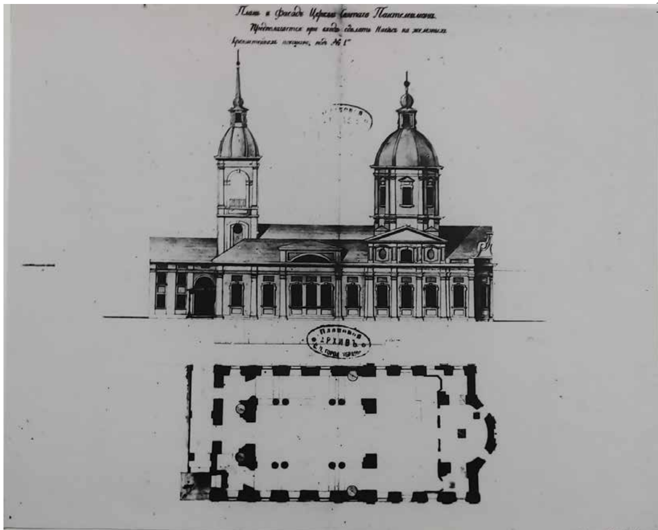
15. План и фасад церкви св. Пантелеймона. Предполагается на входе сделать навес на железных кронштейнах. 1853 г. ЦГАНТД СПб Ф.488. Оп.3-24. Д.713
