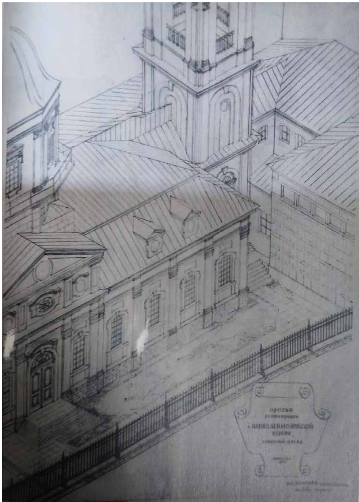
53. Проект реставрации церкви св. Пантелеимона 1984 года. Историческая реконструкция северного фасада. Архив КГИОП, П.192 Пр.2
