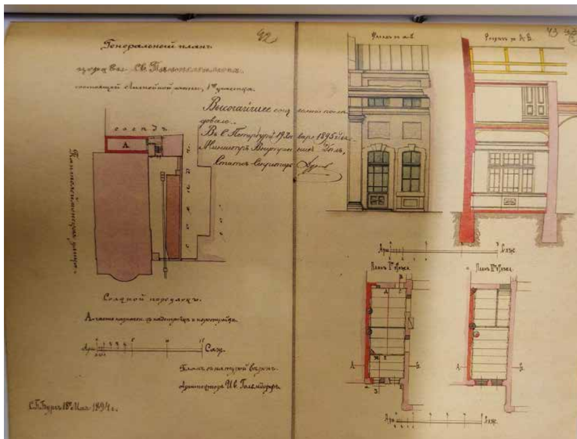
19. Церковь Св. Пантелеимона. Проект перестраиваемых западных помещений. Арх. И.В. Гольмдорф. 1894 г. ЦГИА СПб. Ф.513, оп. 102, д.4338
