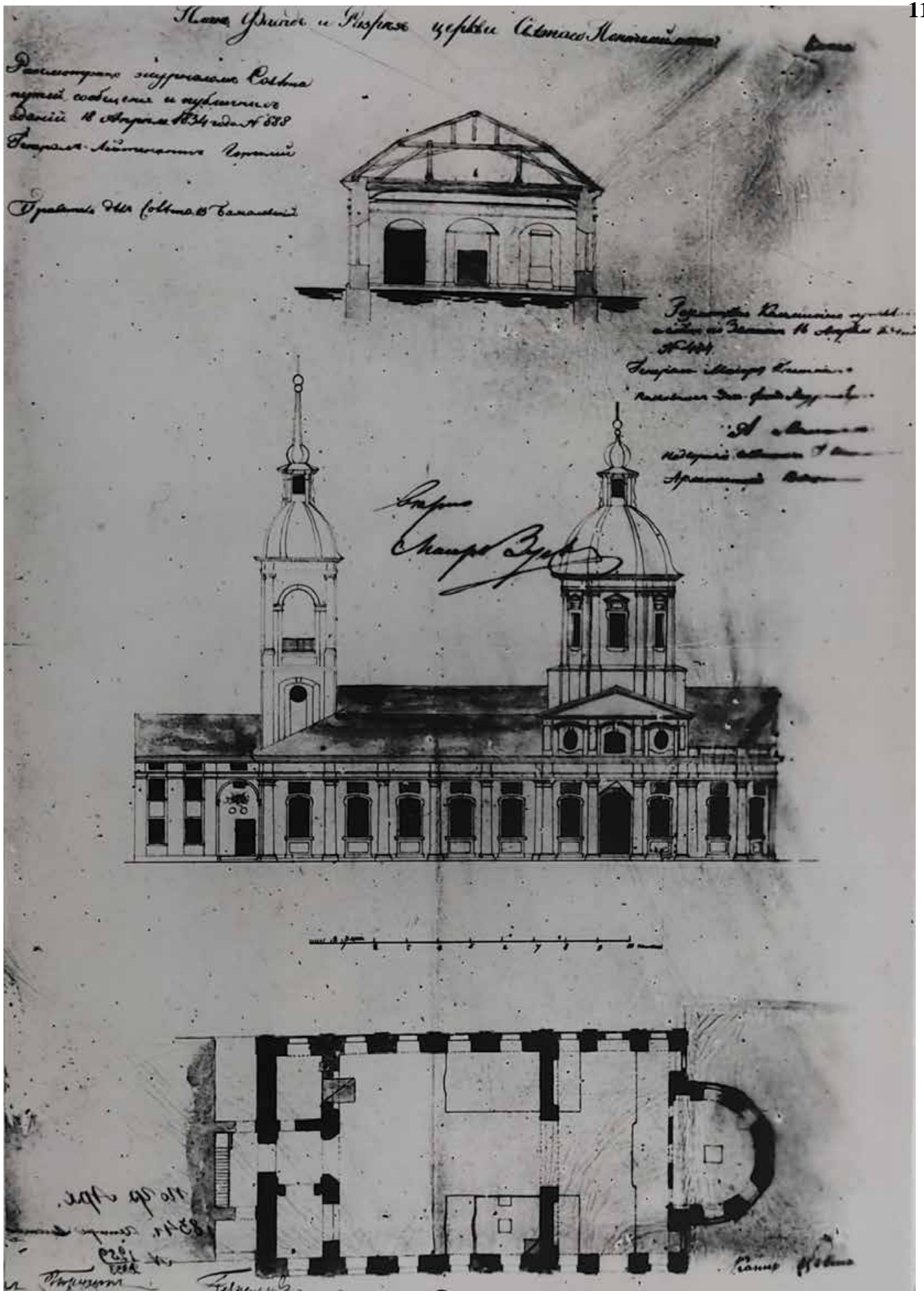
12. План, фасад и разрез церкви св. Пантелеймона. Копия 1779 г. ЦГАНТД СПб Ф.488. Оп.3-24. Д.713
