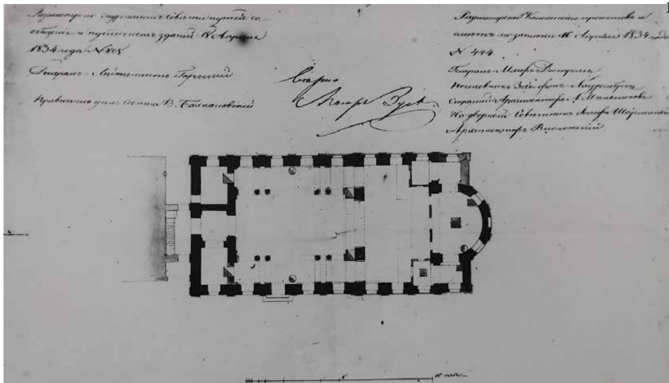
13. План церкви св. Пантелеймона с предполагаемыми переделками. 1834 г. ЦГАНТД СПб Ф.488. Оп.3-24. Д.713
