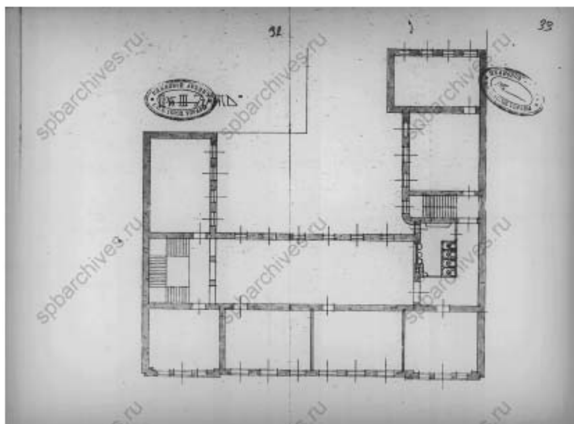
34. Планы 2-го и 3-го этажей. 1909 г. // Источник: ЦГИА СПб Ф.513 Оп.102 Д.1870 Лл.32, 33.
