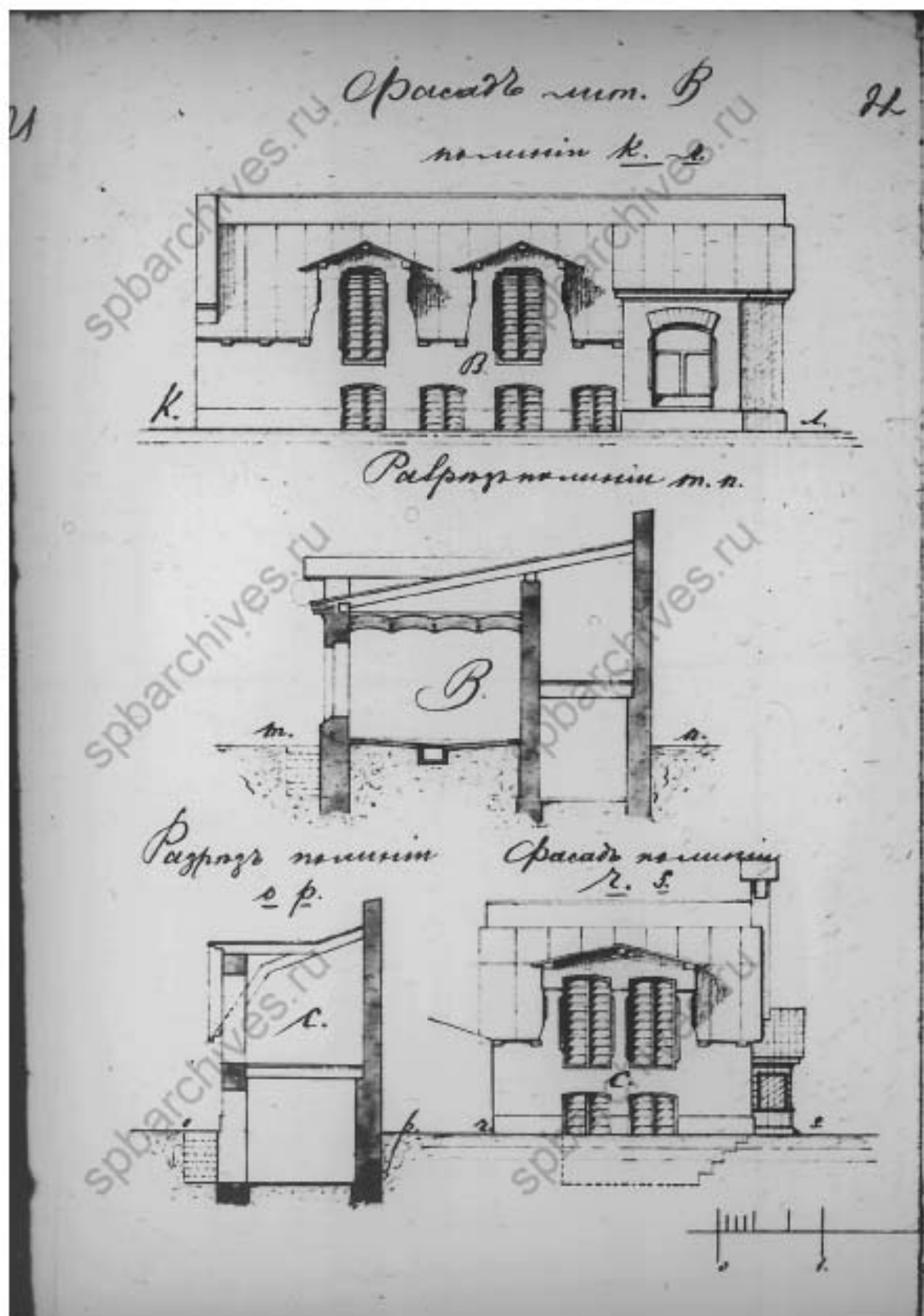
17. Фасад лит. В по линии кл. Разрез по линии тп. Разрез по линии ор. Фасад по линии гс. 1876 г. // Источник: ЦГИА СПб Ф.513 Оп.102 Д.1870 Л.22.
