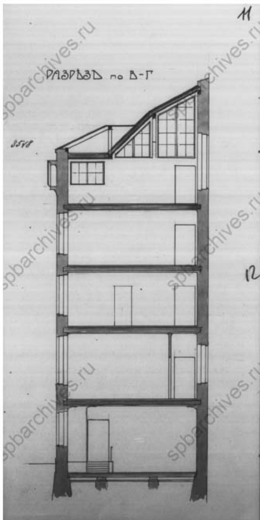
59. Разрез по ВГ. 1912 г. // Источник: ЦГИА СПб Ф.515 Оп.4 Д.2911 Лл.11-12.
