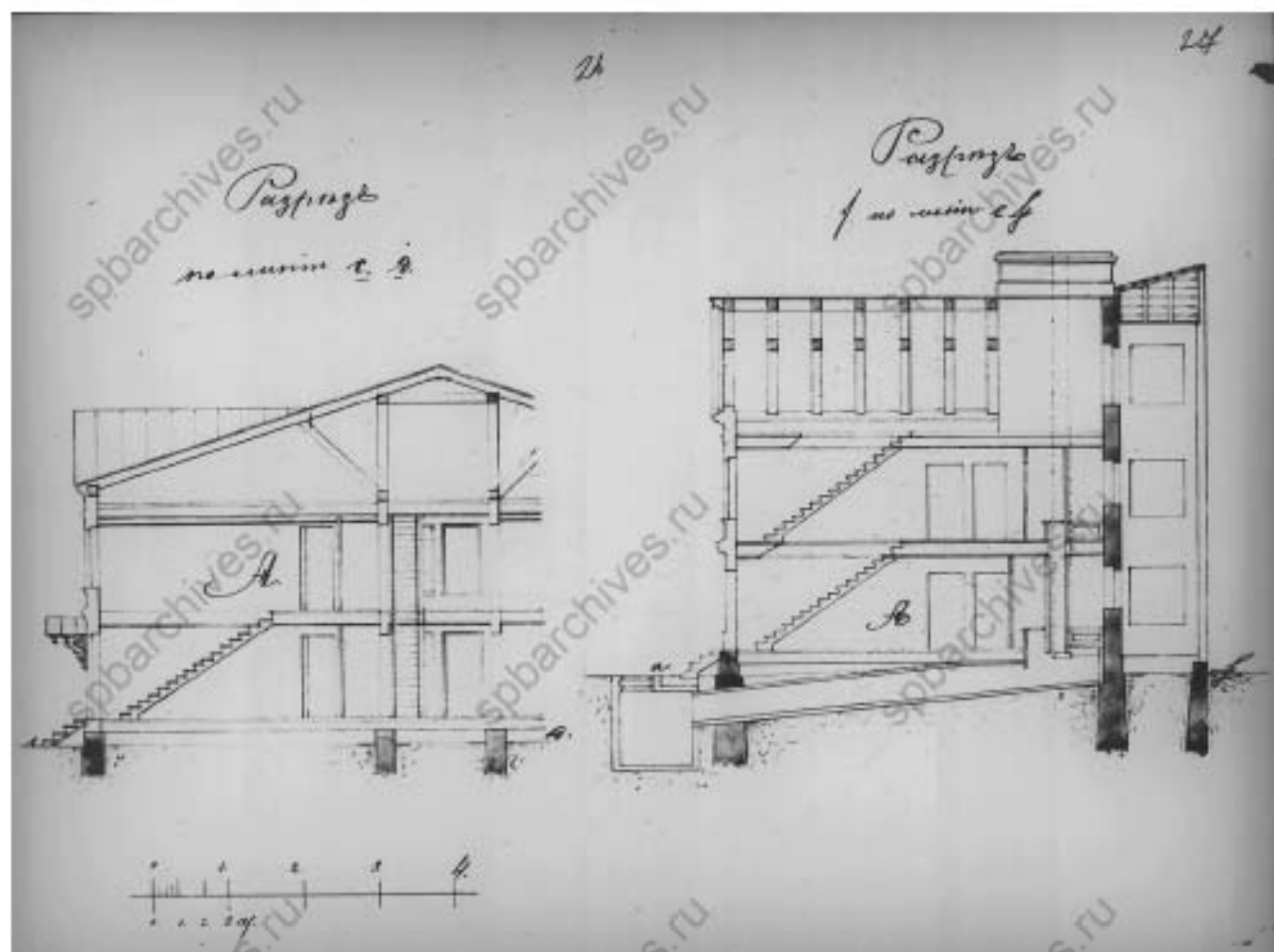
21. Разрез по линии cd. Разрез по линии ef. 1876 г. // Источник: ЦГИА СПб Ф.513 Оп.102 Д.1870 Лл.26, 27.
