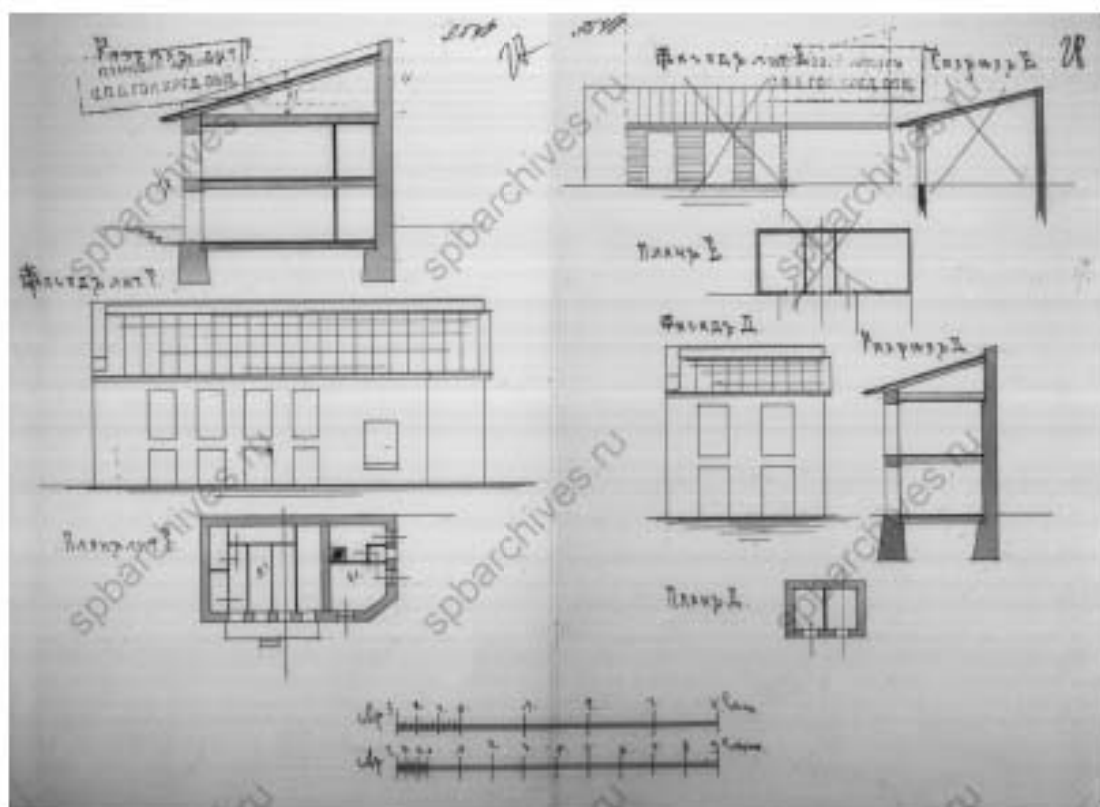
31. Разрезы, планы и фасады лит. Г и лит. Д. 1904 г. // Источник: ЦГИА СПб Ф.515 Оп.4 Д.2911 Лл.27, 28.
