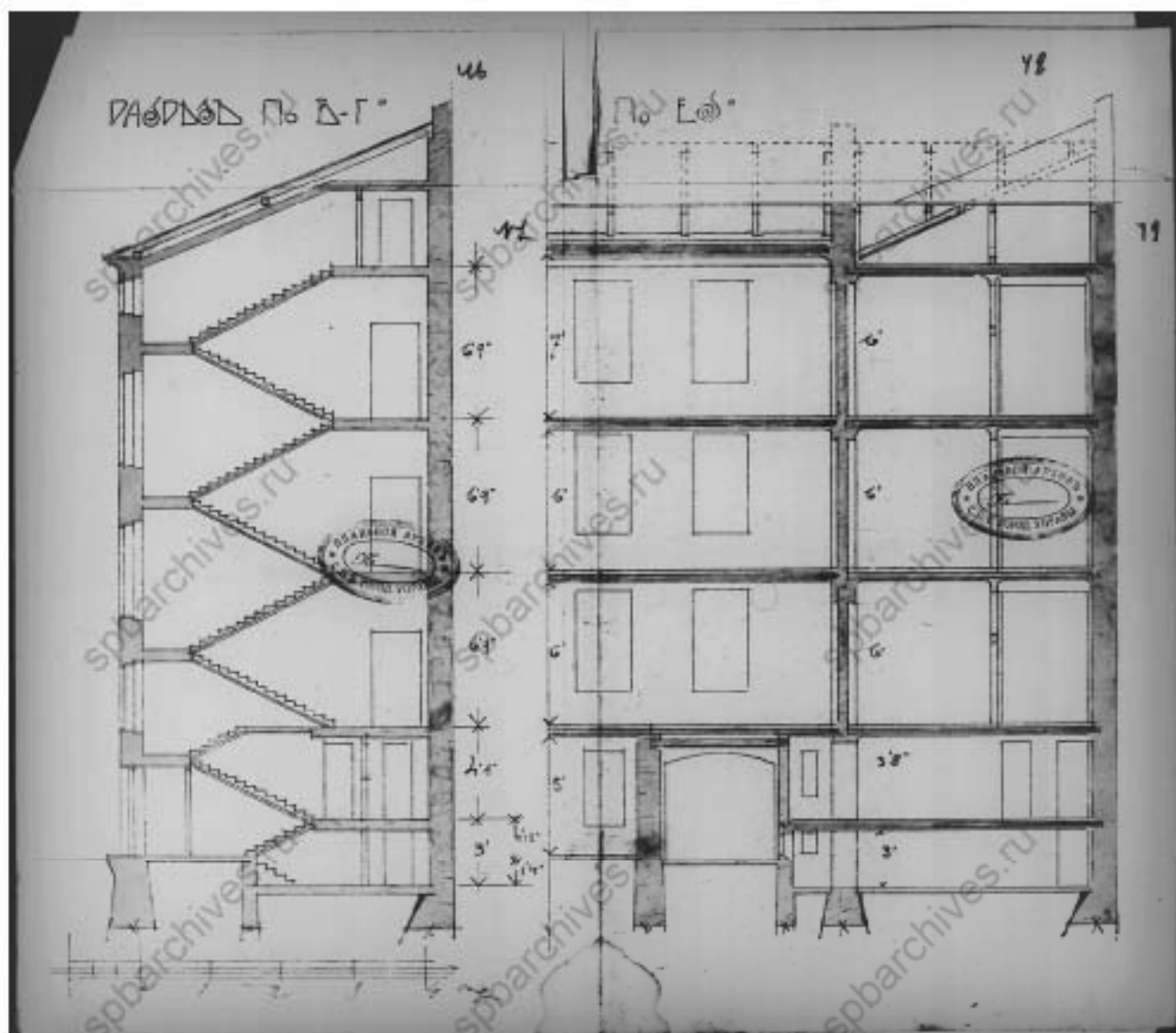
39. Разрез по ВГ. 1909 г. // Источник: ЦГИА СПб Ф.513 Оп.102 Д.1870 Лл.46-49.
