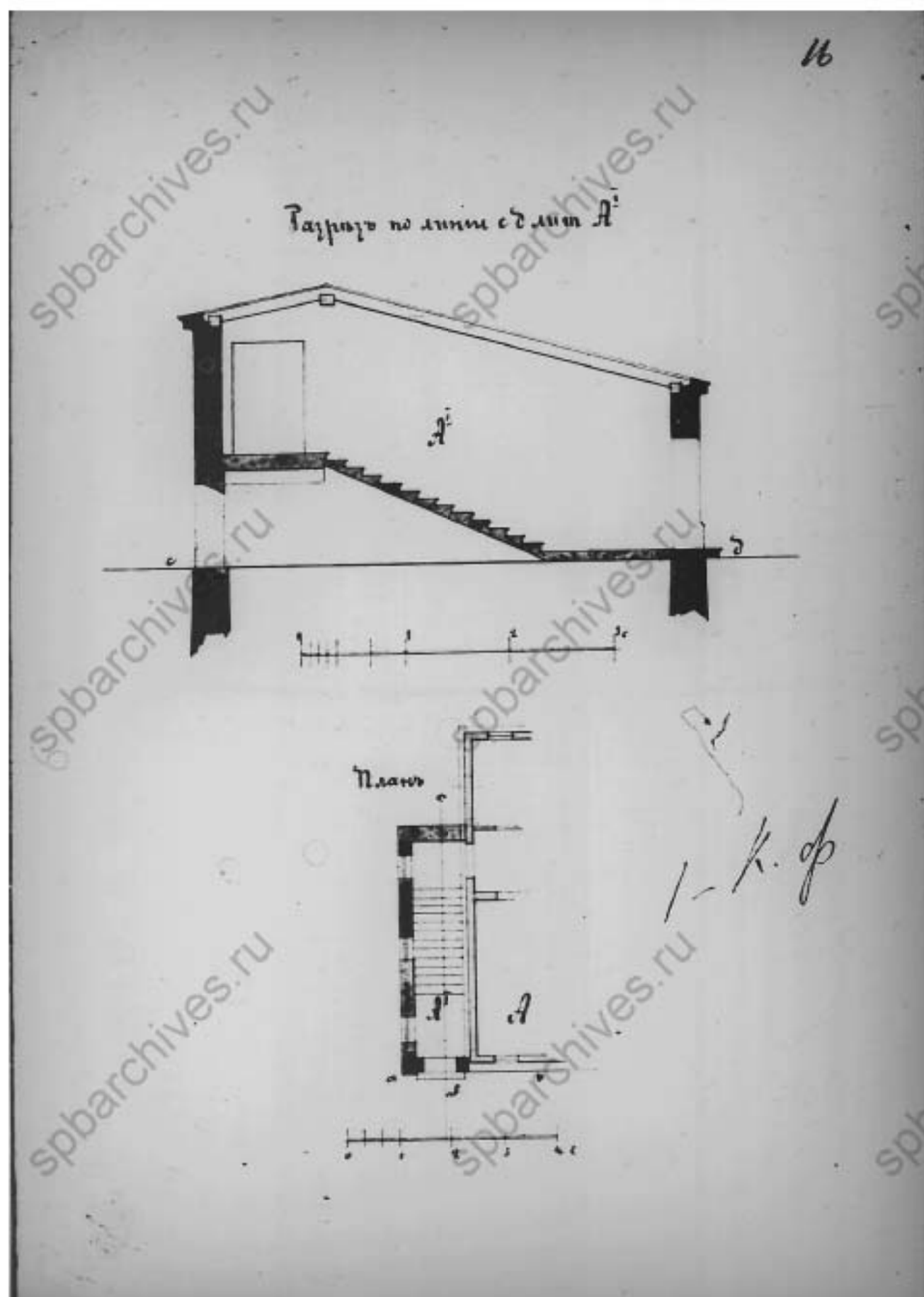
12. Разрезъ по лини сд лит. А'. План. 1873 г. // Источник: ЦГИА СПб Ф.513 Оп.102 Д.1870 Л.16.
