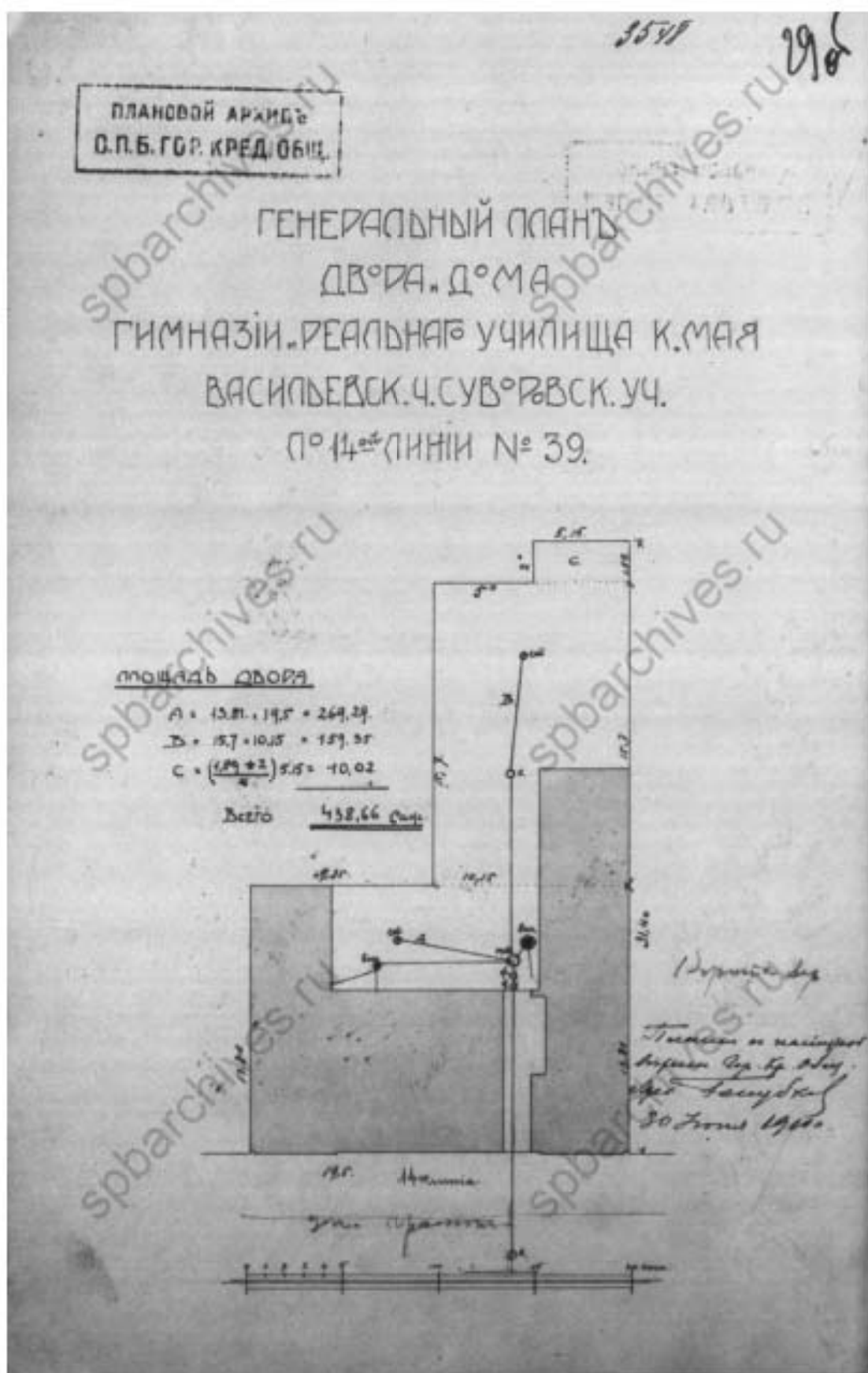
40. Генеральный план двора дома гимназии реального училища К. Мая Васильевск. Ч. Суворовск. Уч. по 14-ой линии №39. 30 июня 1910 г. // Источник: ЦГИА СПб Ф.515 Оп.4 Д.2911 Л.29об.
