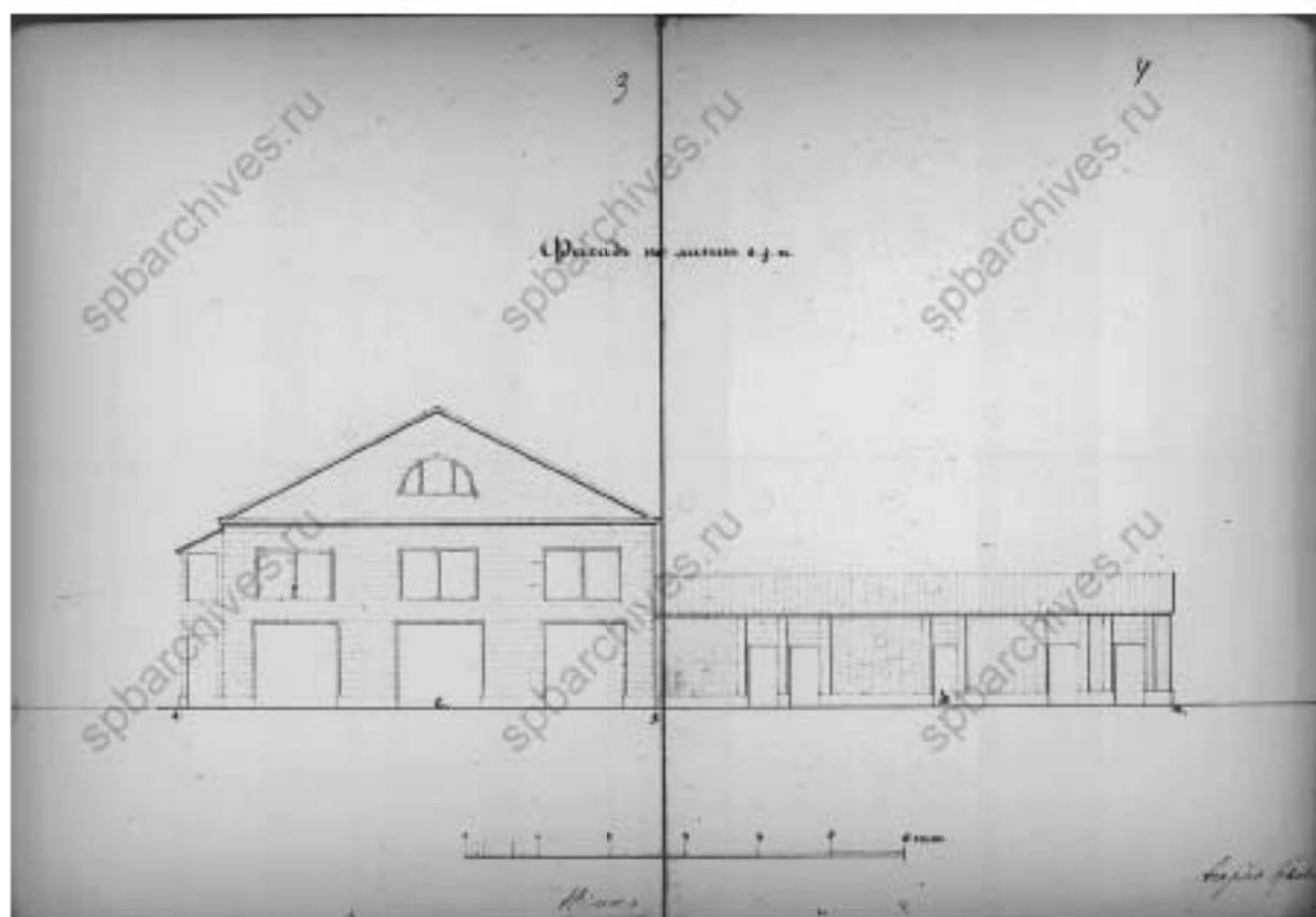
5. Фасад по линии еfn. Строения С и D. 1862 г. // Источник: ЦГИА СПб Ф.513 Оп.102 Д.1870 Лл.3, 4.
