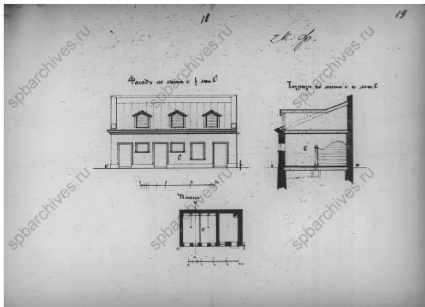
14. Фасад по линии е-ф лит. С. Разрез по линии и-п лит. С. План. 1873 г. // Источник: ЦГИА СПб Ф.513 Оп.102 Д.1870 Лл.18, 19.
