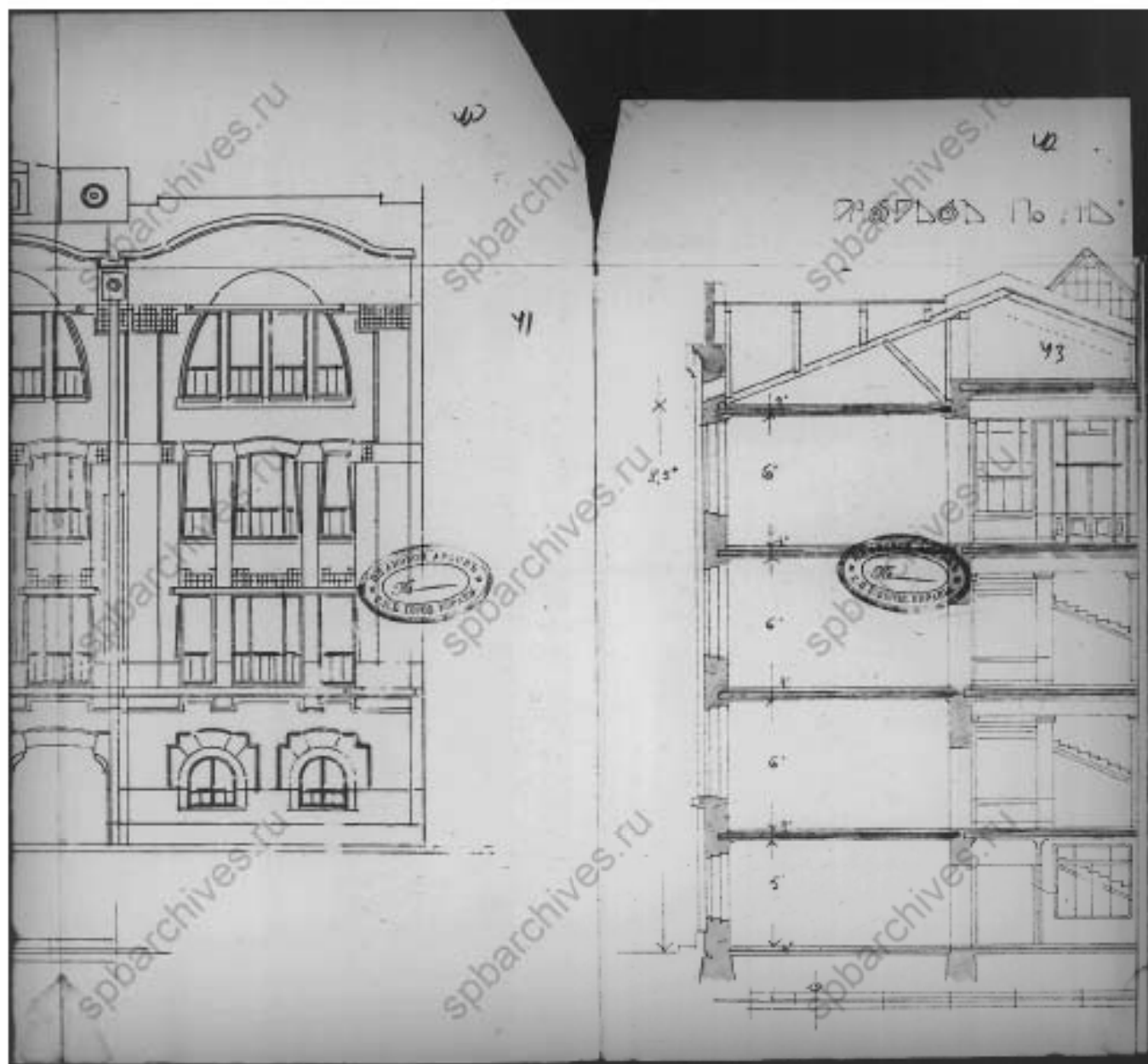
37. Фасад по 14 линии. Фрагмент. Разрез по АБ. Фрагмент. 1909 г. //
