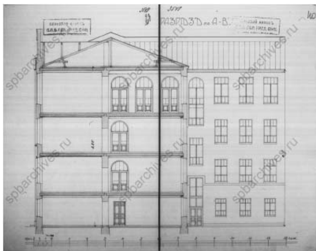
46. Разрез по АВ. // Источник: ЦГИА СПб Ф.515 Оп.4 Д.2911 Лл.39, 40.
