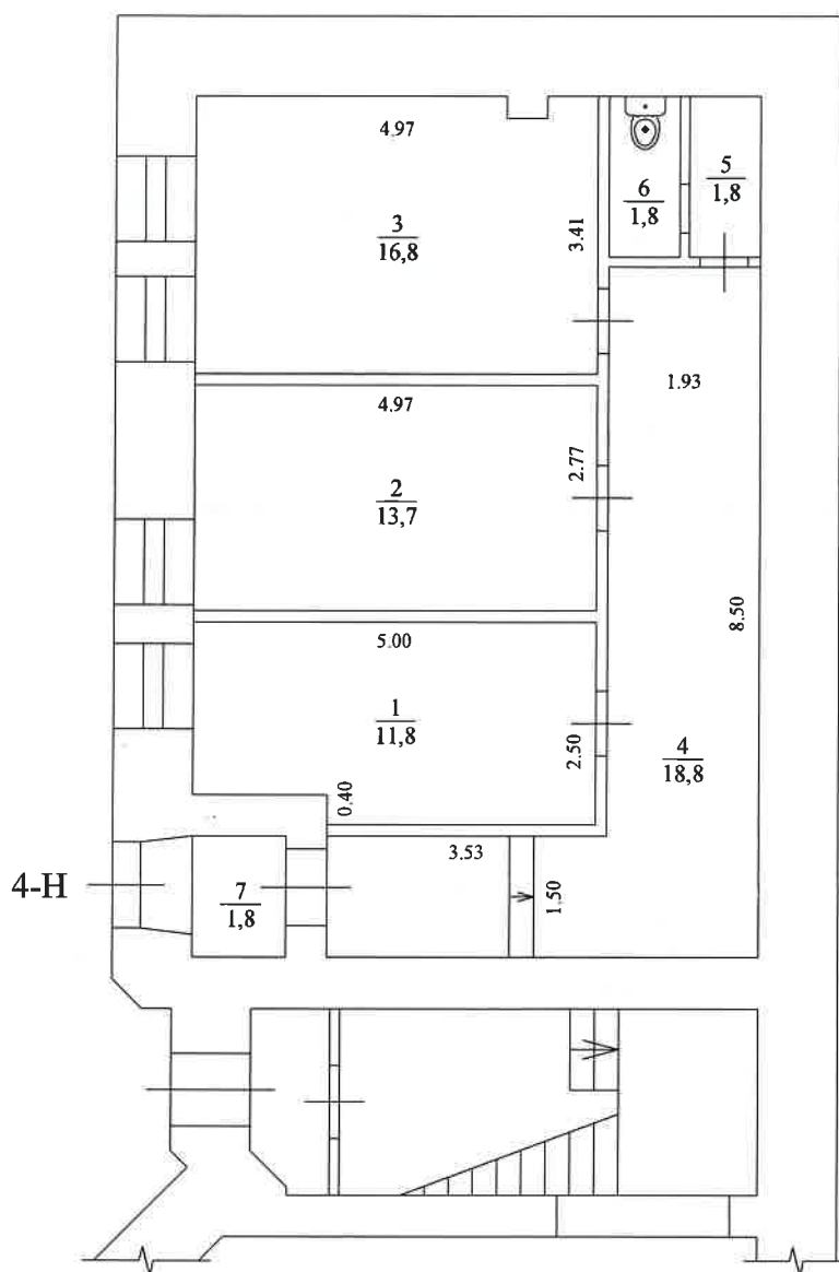
План 1 этажа
