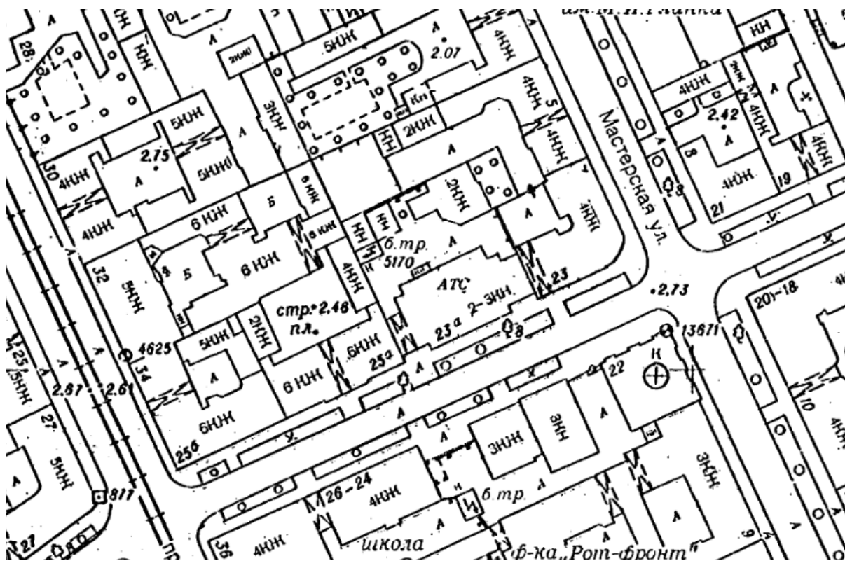
Рис. 11. Токосъёмка 1991 г. М 1:2000. Планшет № 2429-13.
