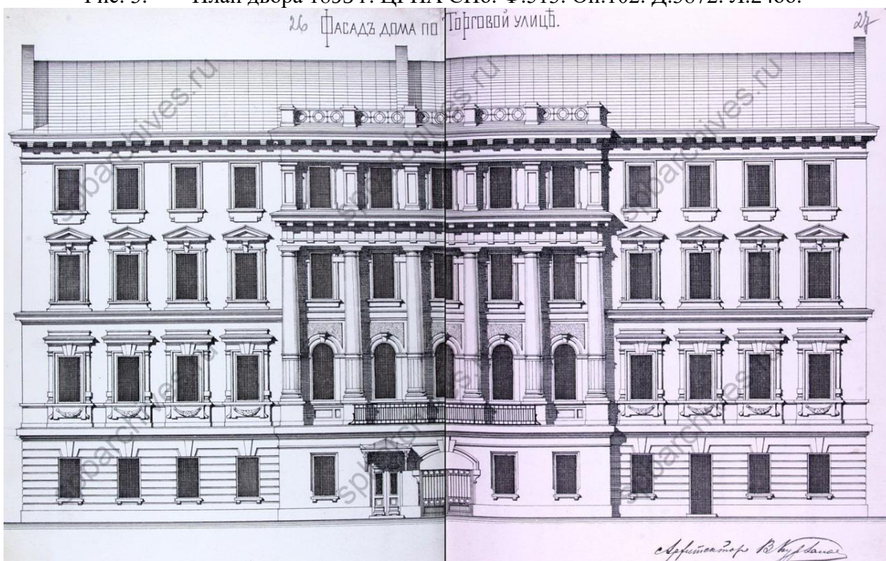
Рис. 4. Фасад дома по Торговой улице. 1895 г. ЦГИА СПб. Ф.513. Оп.102. Д.3872. Л.26-27.
