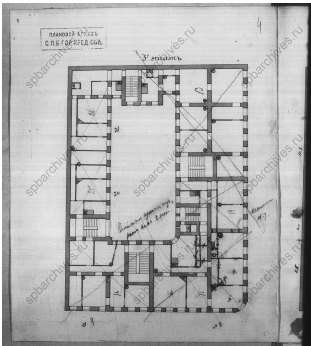
48. ЦГИА СПб. Фонд 515. Опись 4. Дело 4170. 07.12.1873 г. Чертежи дома Е.В. Артемьевой по Б. Мещанской ул., 36 и Демидову пер., 7 (Казанской ул., 34 и Демидову пер., 7). Петроградское городское кредитное общество. Петроград. 1861-1919 гг. План 3-го этажа.
