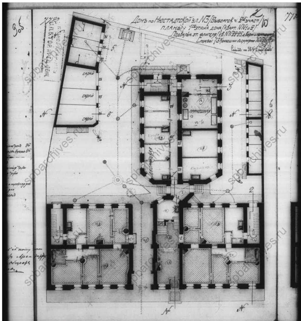
9. Дом по Нюстадской ул., №3. План 1-го этажа дома, подвалн. эт. флигеля. 1904 г. // ЦГИА СПб. ф.515 оп.4 д.2413. Л.10.
