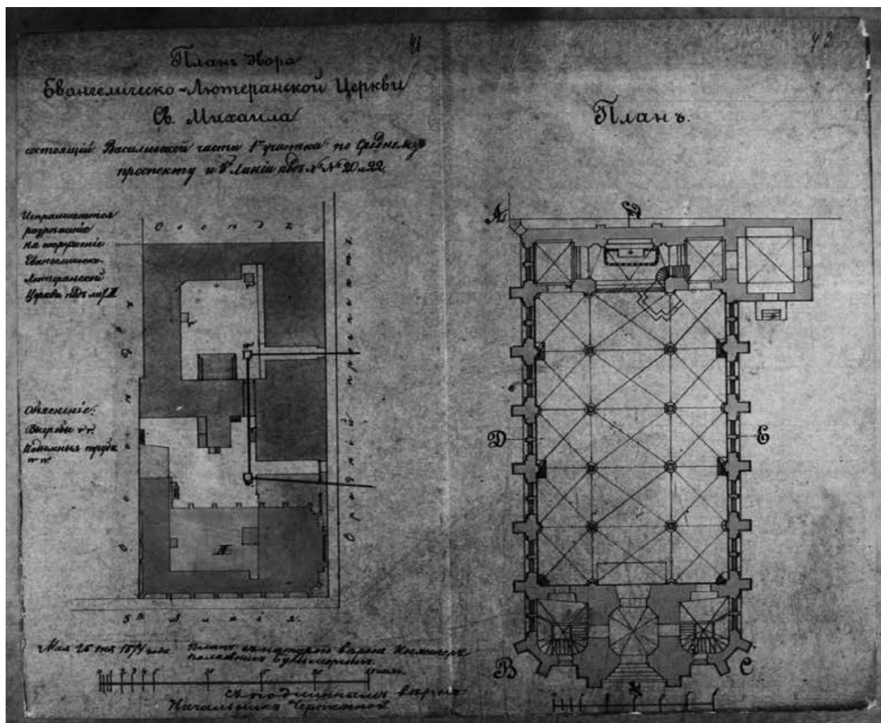
Илл. 27. План двора Евангелическо-Лютеранской Церкви Св. Михаила, состоящий Васильевской части 1-го участка по Среднему проспекту и 3-й линии под №№ 20 и 22. 1874 г. (источник: ЦГИА СПб: Фонд 513. Опись 102. Дело 2369).
