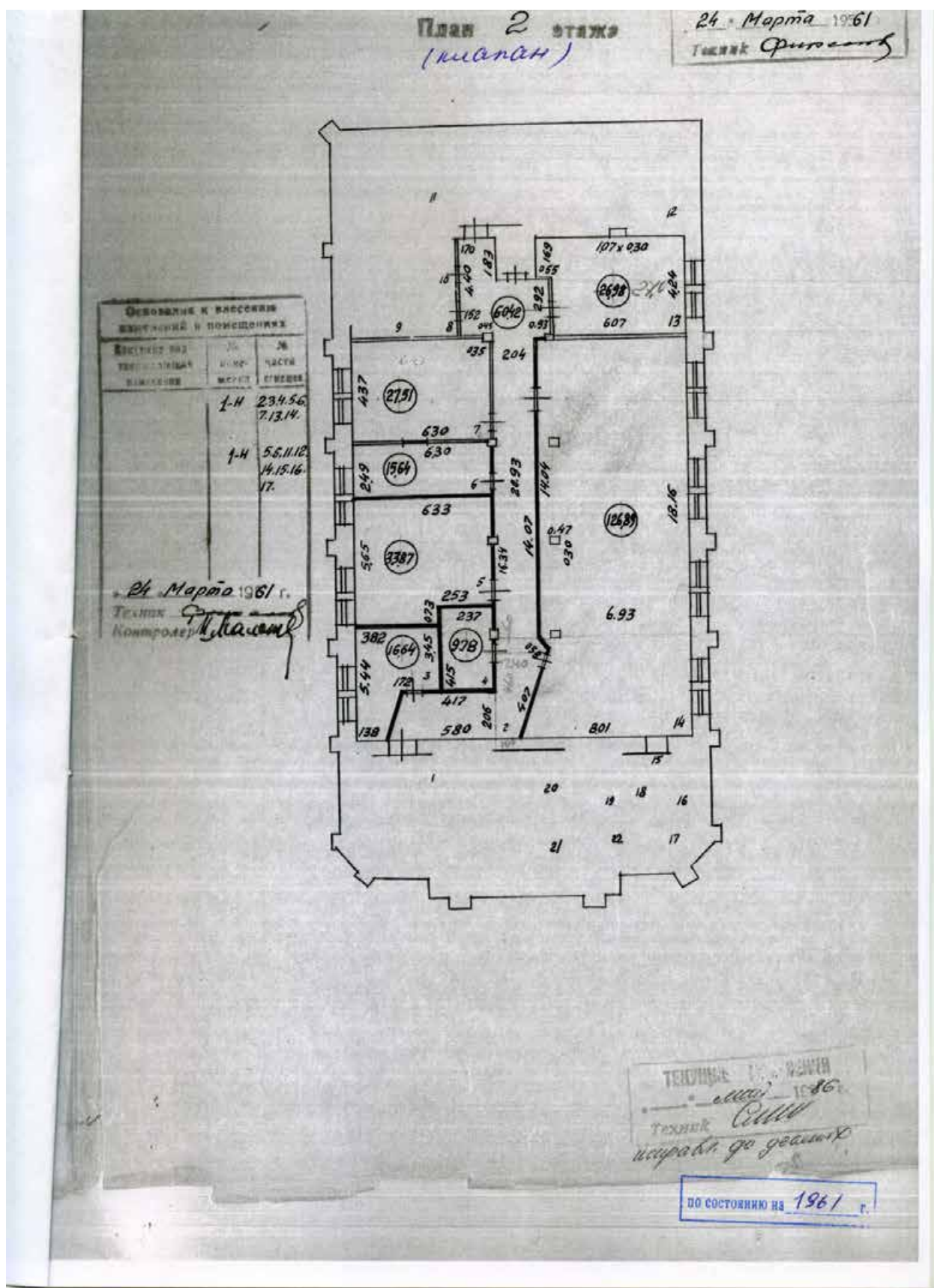
Илл. 64. План 2-го этажа. Архивные чертежи ПИБ здания по адресу: Санкт-Петербург, Средний пр. В.О., 18. 1961 г. (источник: СПб ГБУ «ГУИОН»).
