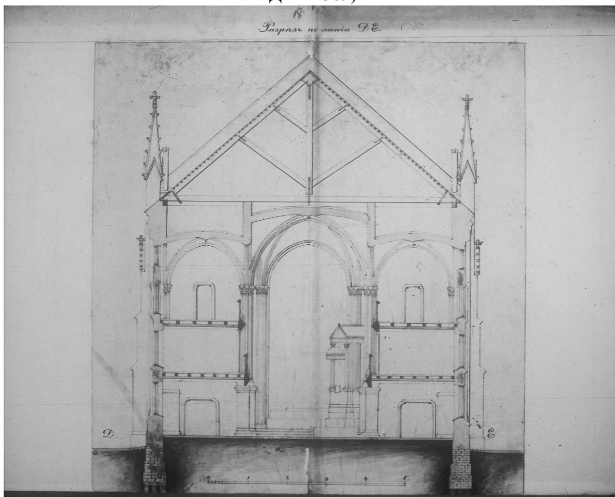
Илл. 20. Разрез по линии Д-Е. 1872 г. (источник: ЦГИА СПб: Фонд 513. Описание 102. Дело 2369).
