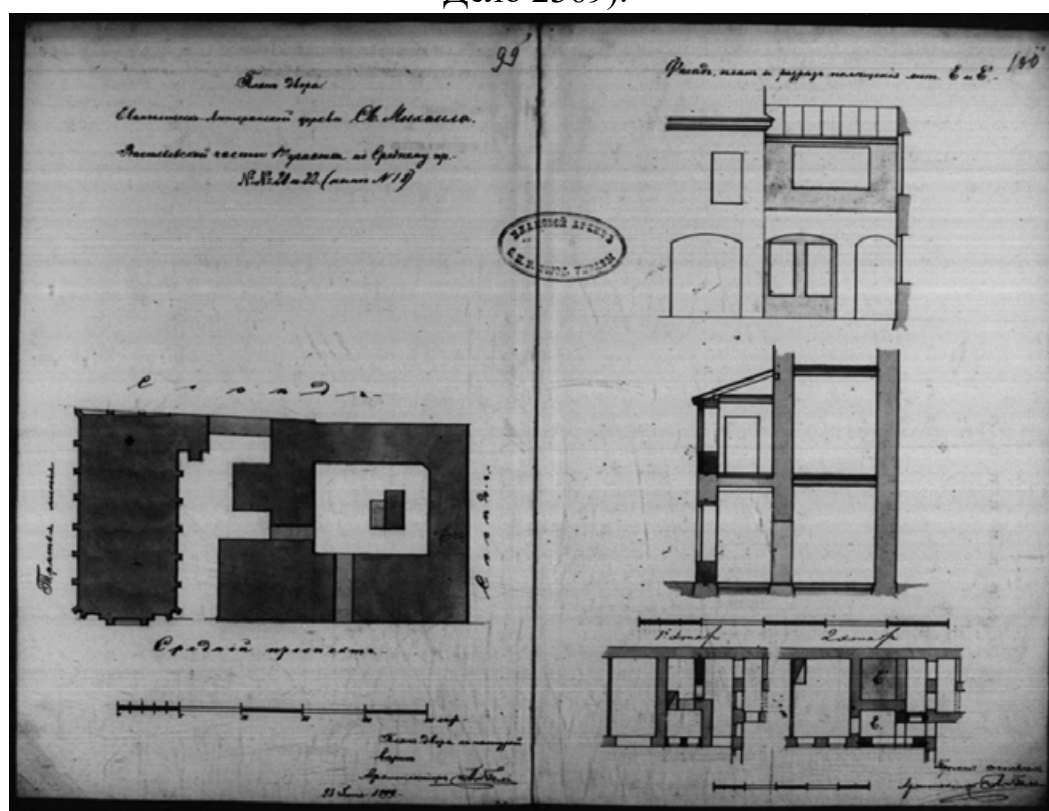
Илл. 48. План двора Евангелическо-Лютеранской Церкви Св. Михаила Васильевской части 1-го участка по Среднему проспекту № 20 и 22 (под № 18). Фасад, план и разрез помещения лит. Е и Е'. 1899 г. (источник: ЦГИА СПб: Фонд 513. Опись 102. Дело 2369).
