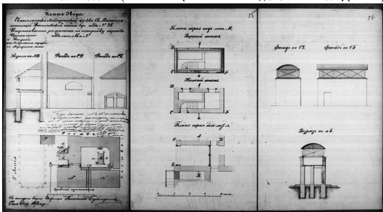
Илл. 33. План двора Евангелическо-Лютеранской Церкви Св. Михаила, состоящий Васильевской части 1-го участка под № 21. Планы сарая под лит. М. Планы сарая под лит. Л. Фасад по С-Д. Фасад по С-В. Разрез по а-б. 1874 г. (источник: ЦГИА СПб: Фонд 513. Описание 102. Дело 2369).
