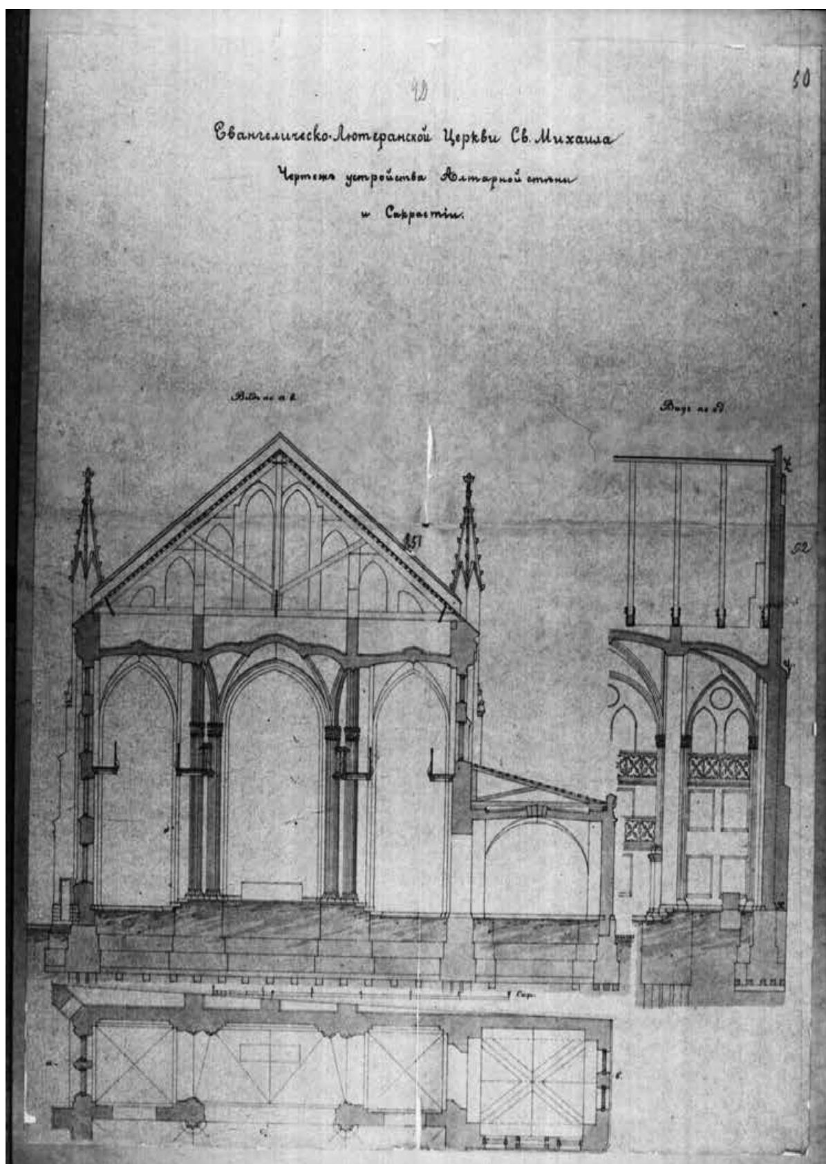
Илл. 31. Чертеж устройства Алтарной стены и Сакристия Евангелическо-Лютеранской Церкви Св. Михаила. Вид по а-в. Вид по с-д. Фрагмент плана. 1874 г. (источник: ЦГИА СПб: Фонд 513. Опись 102. Дело 2369).
