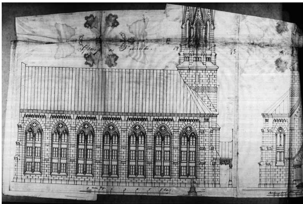
Илл. 44. Фасад по 3-й линии Евангелическо-Лютеранской Церкви Св. Михаила. 1886 г. (источник: ЦГИА СПб: Фонд 513. Опись 102. Дело 2369).
