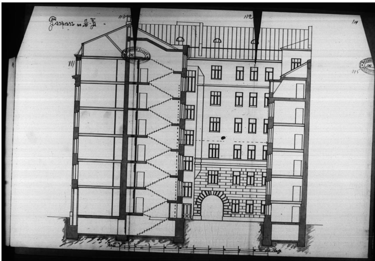
Илл. 50. Разрез по А-Б. 1913 г. (источник: ЦГИА СПб: Фонд 513. Опись 102. Дело 2369).
