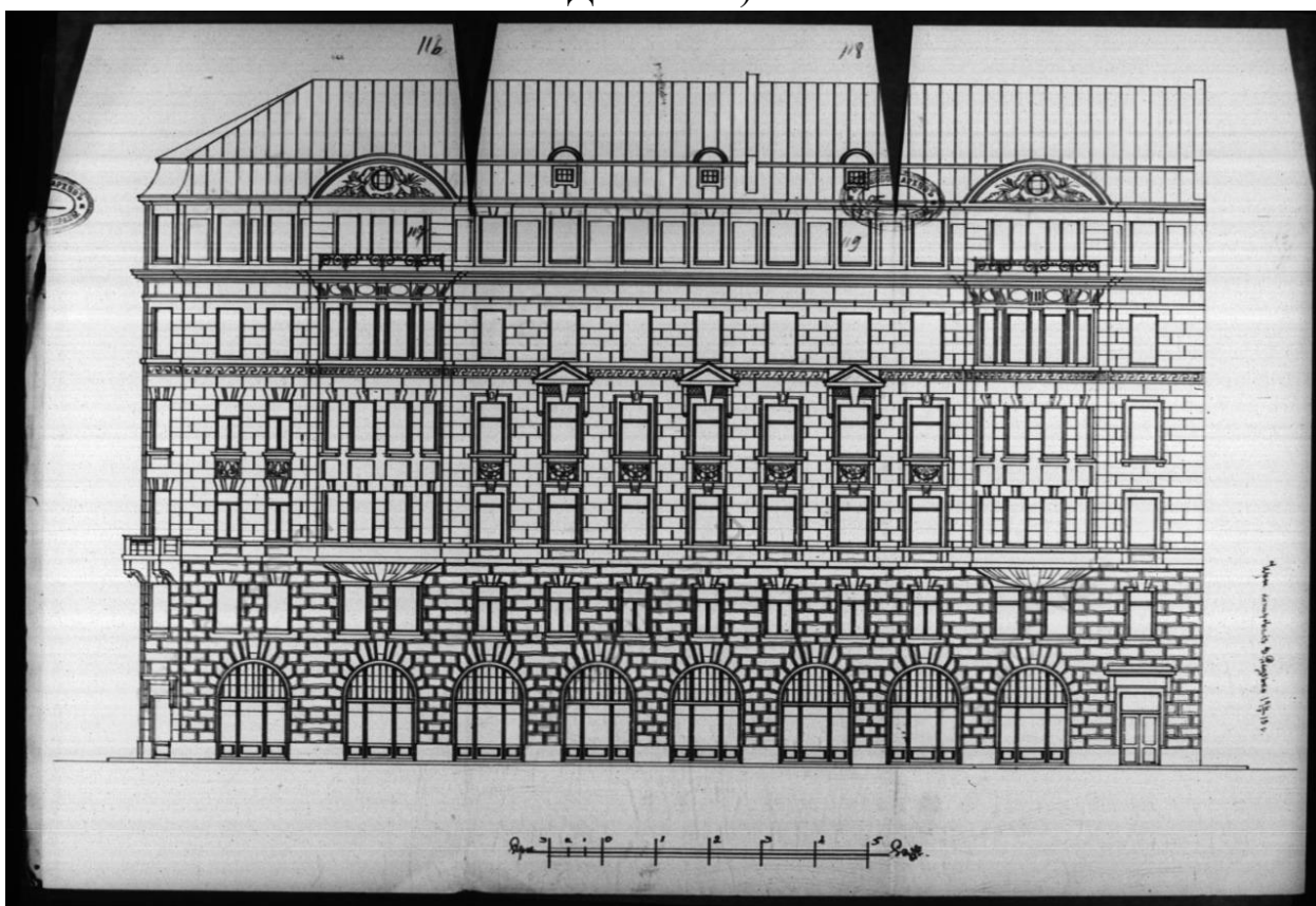
Илл. 51. Фасад. 1913 г. (источник: ЦГИА СПб: Фонд 513. Опись 102. Дело 2369).
