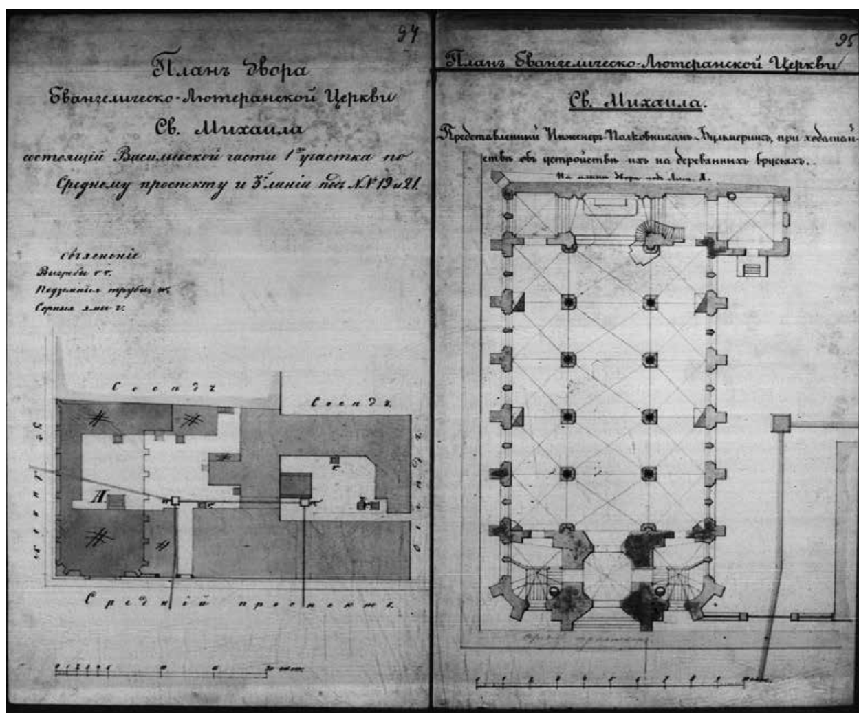
Илл. 46. План двора Евангелическо-Лютеранской Церкви Св. Михаила состоящий Васильевской части 1-го участка по Среднему проспекту и 3-й линии, № 19 и 21. План церкви. 1888 г. (источник: ЦГИА СПб: Фонд 513. Опись 102. Дело 2369).
