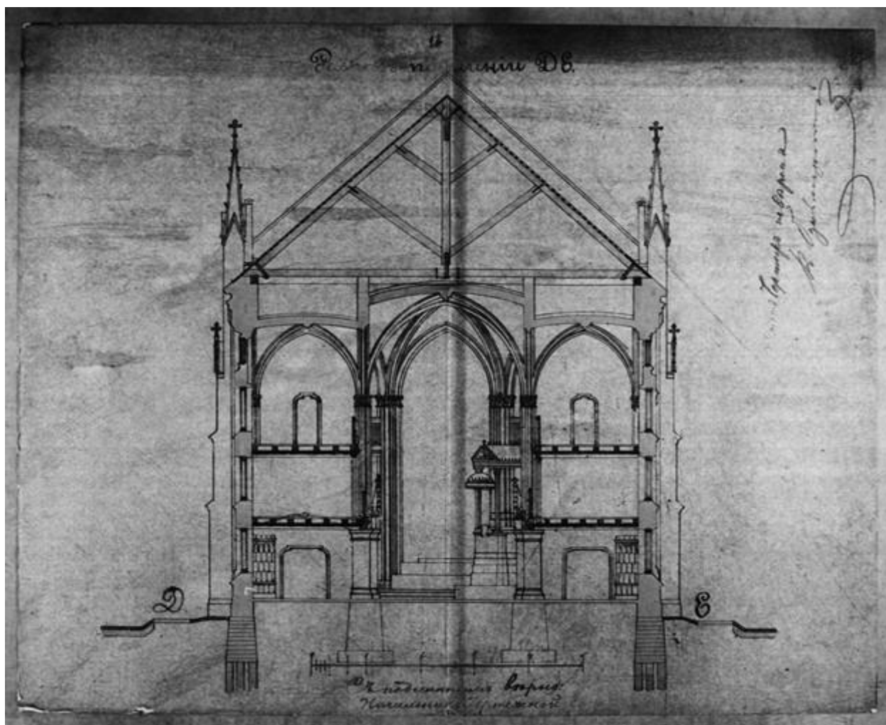
Илл. 29. Разрез по Д-Е. 1874 г. (источник: ЦГИА СПб: Фонд 513. Опись 102. Дело 2369).
