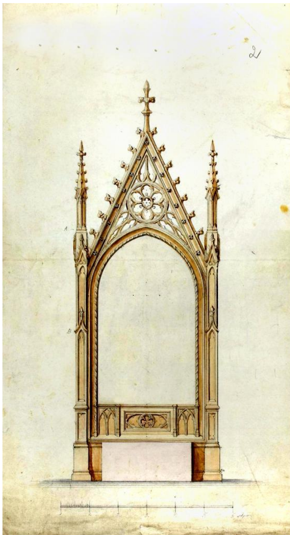
Илл. 40. Чертежи алтаря евангелическо-лютеранской церкви св. Михаила по Среднему пр. В.О., N 18. 1876 г. (источник: ЦГИА СПб: Фонд 513. Опись 169. Дело 154).
