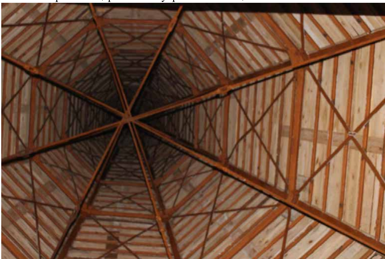
Фото 28. Объект культурного наследия регионального значения «Лютеранская церковь». Стропильная система шпиля башни-колокольни.
