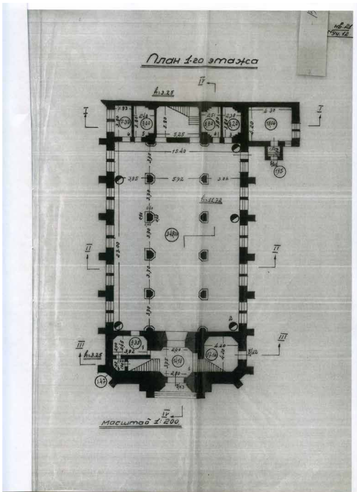
Илл. 53. План 1-го этажа. Архивные чертежи ПИБ здания по адресу: Санкт-Петербург, Средний пр. В.О., 18. 1947 г. (источник: СПб ГБУ «ГУИОН»).
