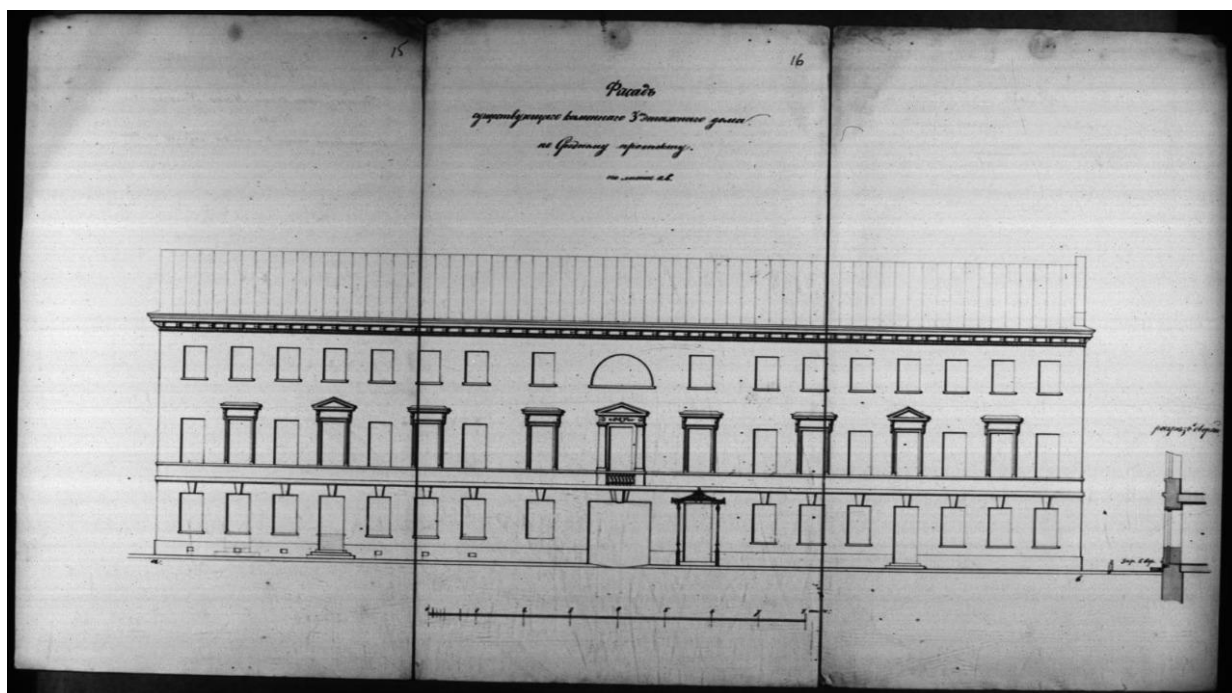
Илл. 19. Фасад существующего каменного 3-х этажного дома по Среднему проспекту по линии а-в. 1872 г. (источник: ЦГИА СПб: Фонд 513. Описание 102. Дело 2369).
