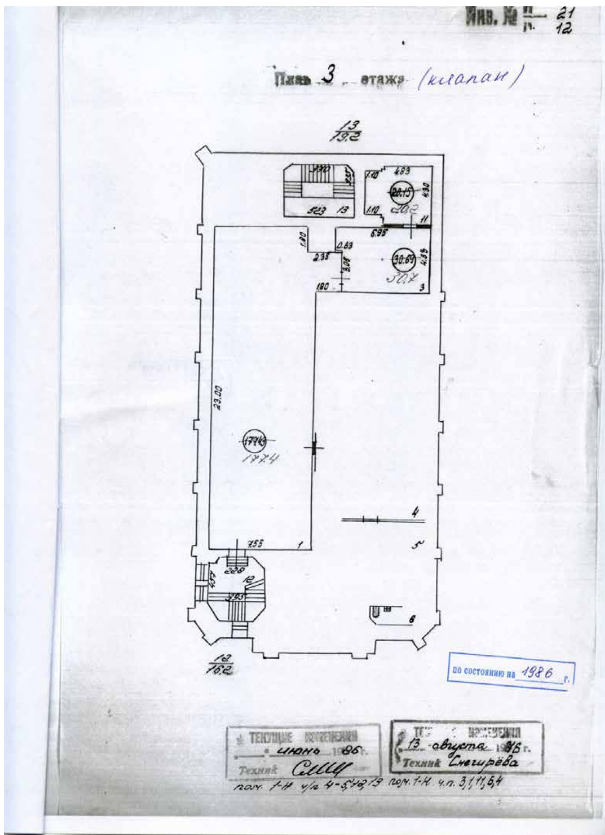
Илл. 71. План 3-го этажа. Архивные чертежи ПИБ здания по адресу: Санкт-Петербург, Средний пр. В.О., 18. 1986 г. (источник: СПб ГБУ «ГУИОН»).
