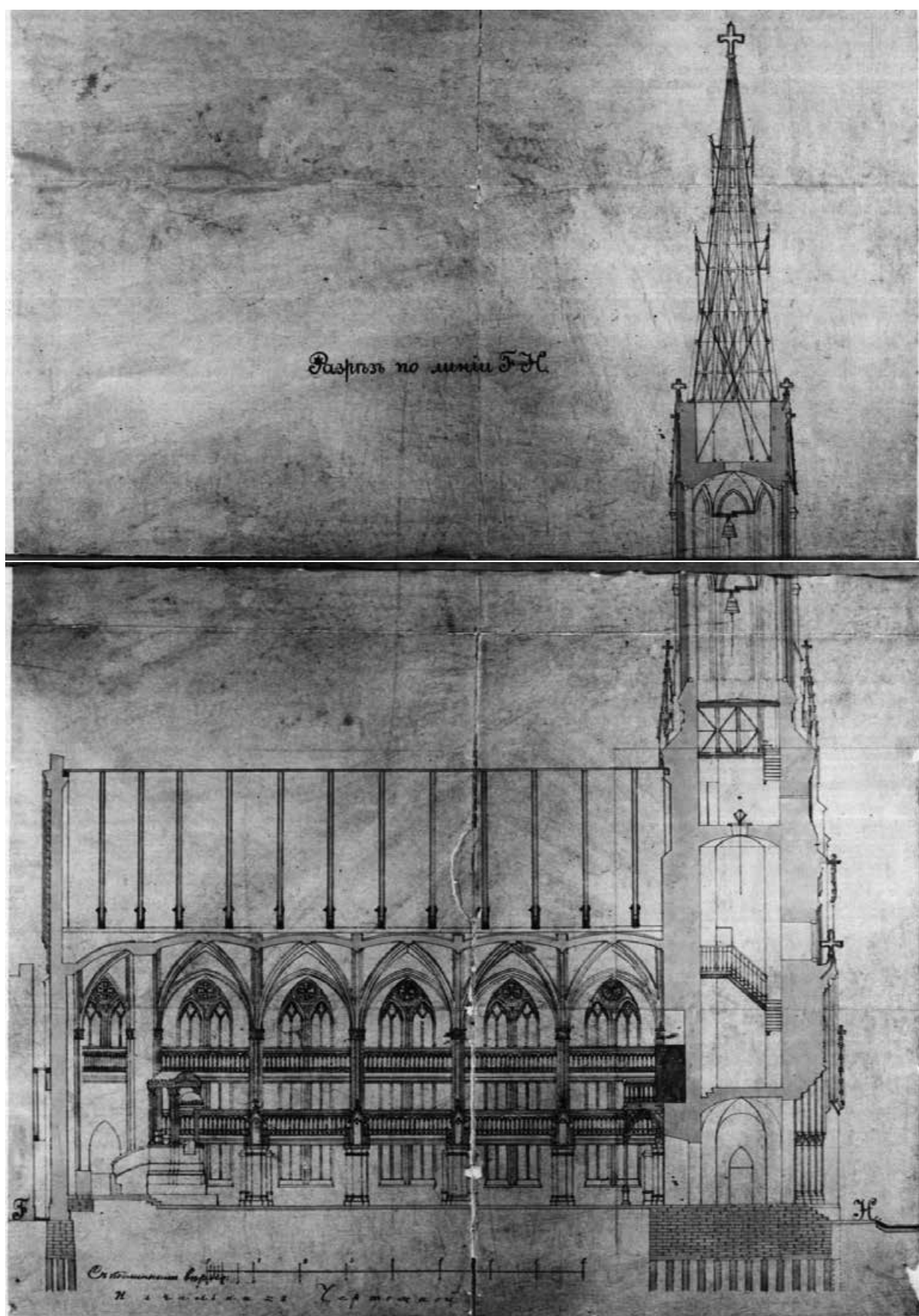
Илл. 23. Разрез по линии Г-Н. 1874 г. (источник: ЦГИА СПб: Фонд 513. Опись 102. Дело 2369).
