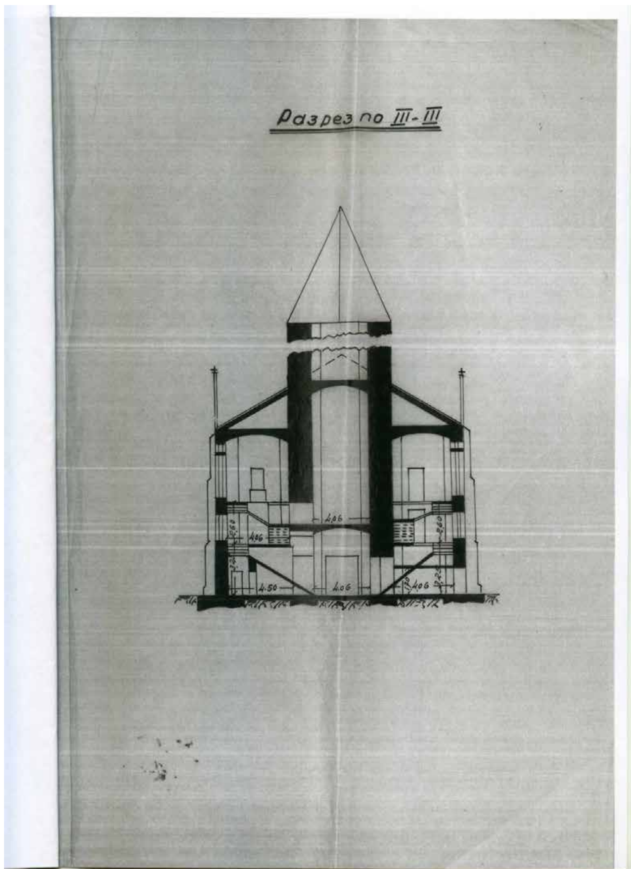
Илл. 57. Поперечный разрез. Архивные чертежи ПИБ здания по адресу: Санкт-Петербург, Средний пр. В.О., 18. 1947 г. (источник: СПб ГБУ «ГУИОН»).
