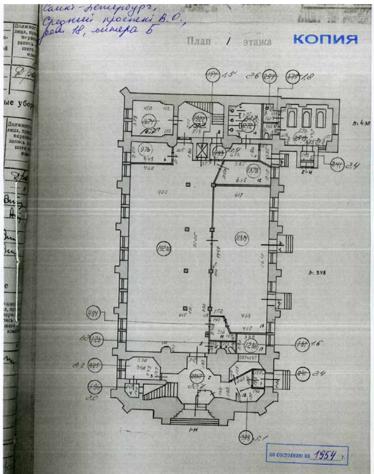
Илл. 60. План 1-го этажа. Архивные чертежи ПИБ здания по адресу: Санкт-Петербург, Средний пр. В.О., 18. 1954 г. (источник: СПб ГБУ «ГУИОН»).
