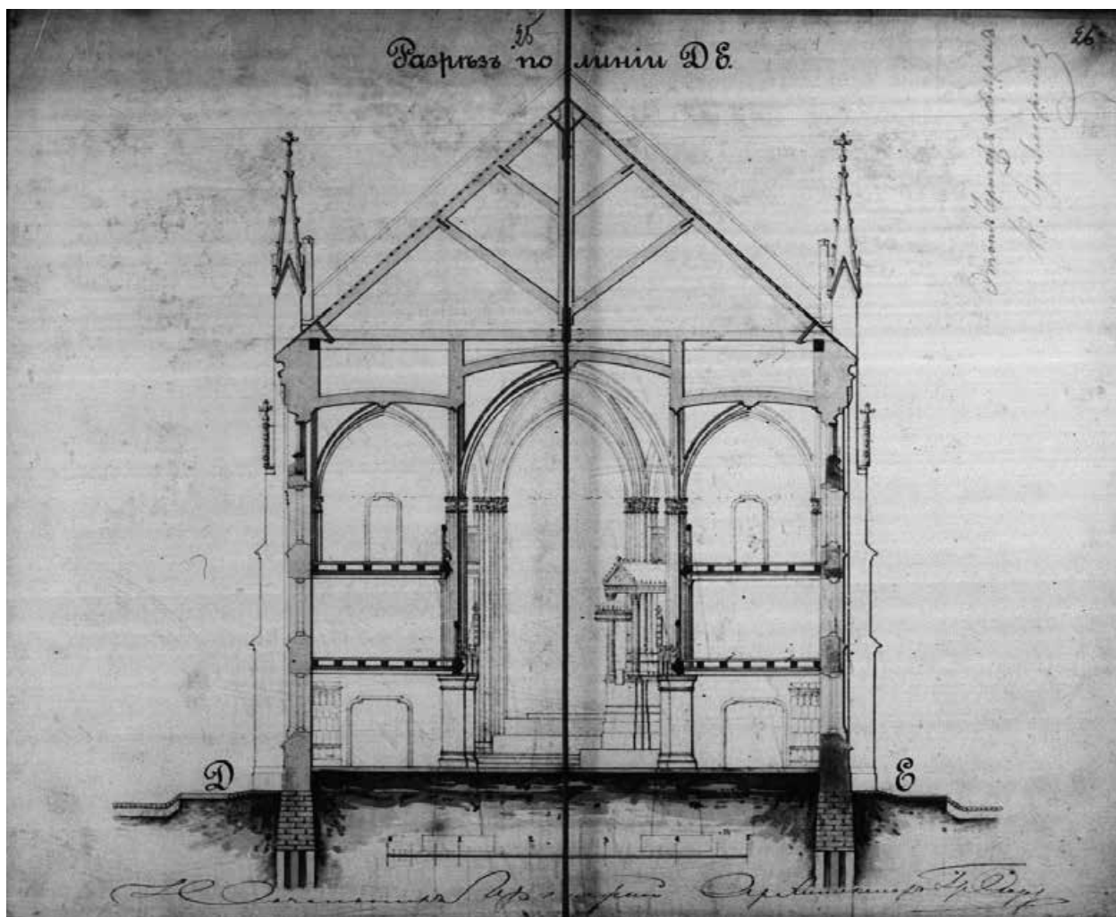
Илл. 22. Разрез по линии Д-Е. 1874 г. (источник: ЦГИА СПб: Фонд 513. Опись 102. Дело 2369).
