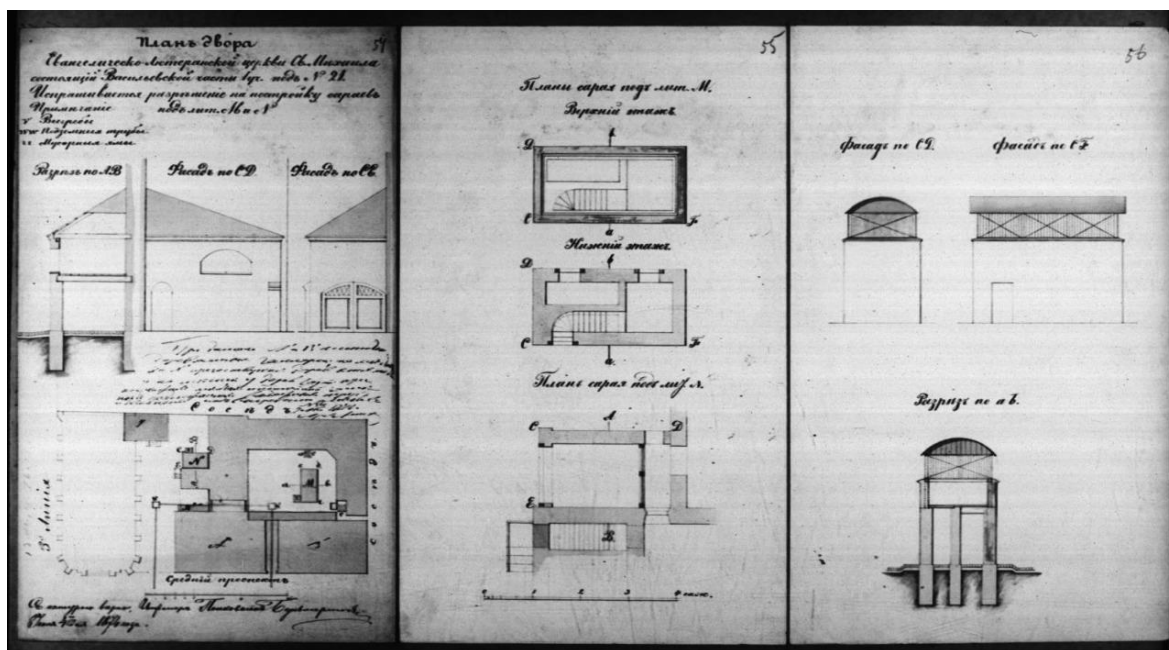
Илл. 35. Фасад существующий по А-В. Планы дома на плане двора лит. В. Фасад, предполагаемый по А-В. 1874 г. (источник: ЦГИА СПб: Фонд 513. Опись 102. Дело 2369).
