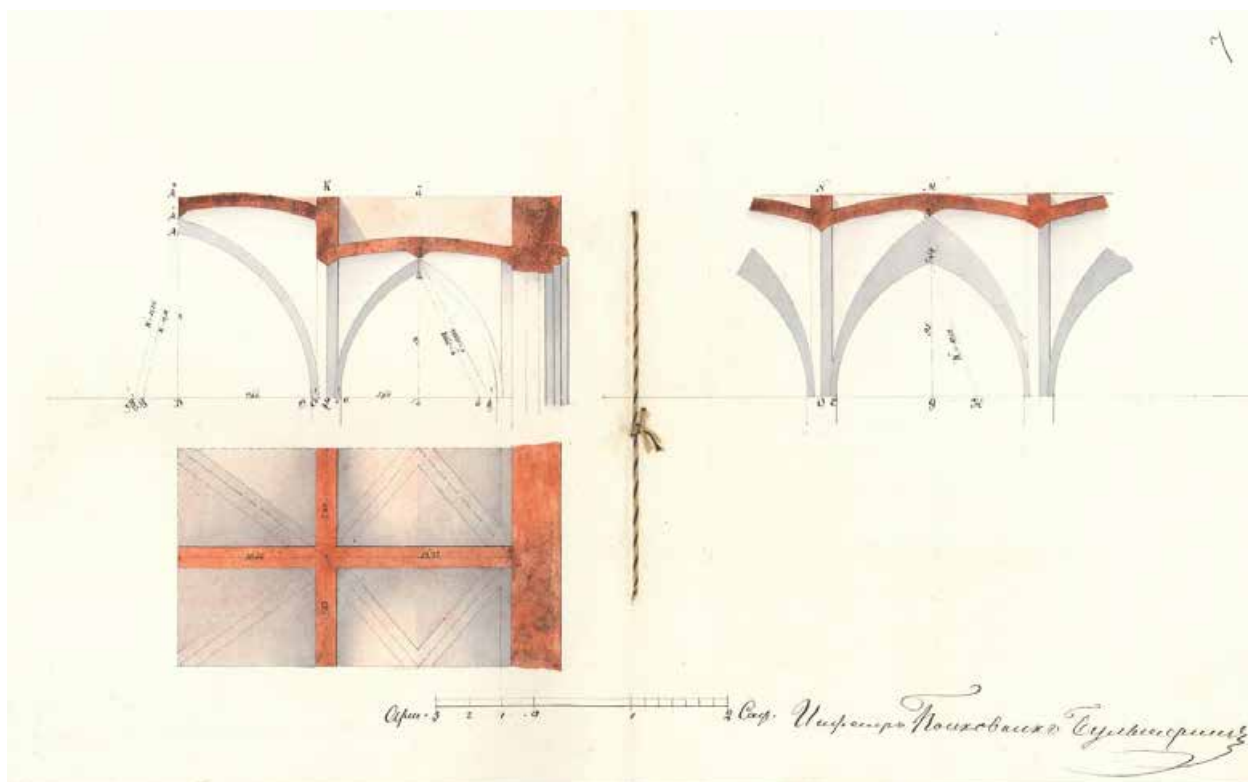
Илл. 32. Чертеж устройства сводов Евангелическо-Лютеранской Церкви Св. Михаила. 1874-1875 гг. (источник: ЦГИА СПб: Фонд 513. Описание 59. Дело 21)
