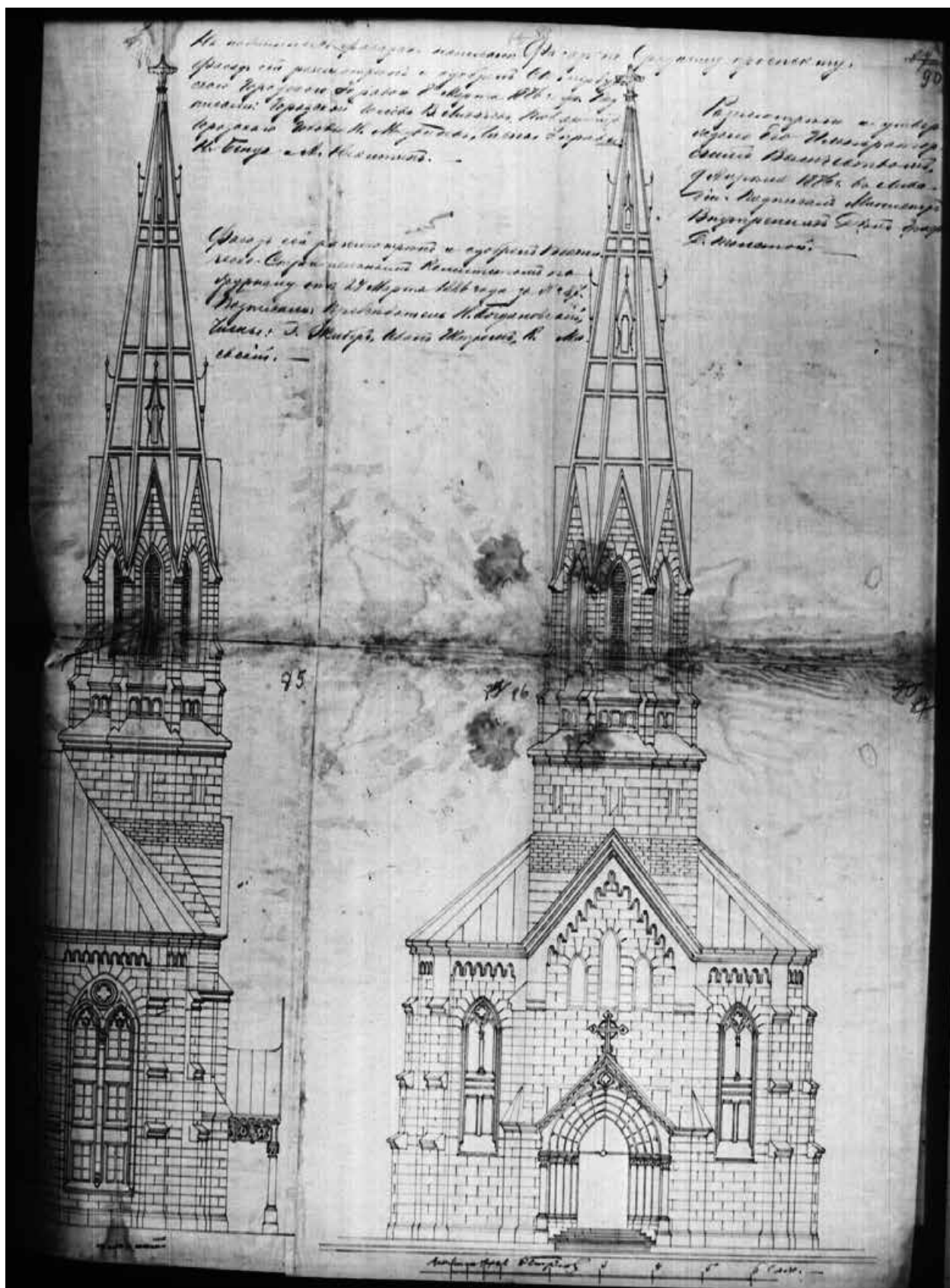
Илл. 43. Фасад по 3-й линии Евангелическо-Лютеранской Церкви Св. Михаила. 1886 г. (источник: ЦГИА СПб: Фонд 513. Опись 102. Дело 2369)
