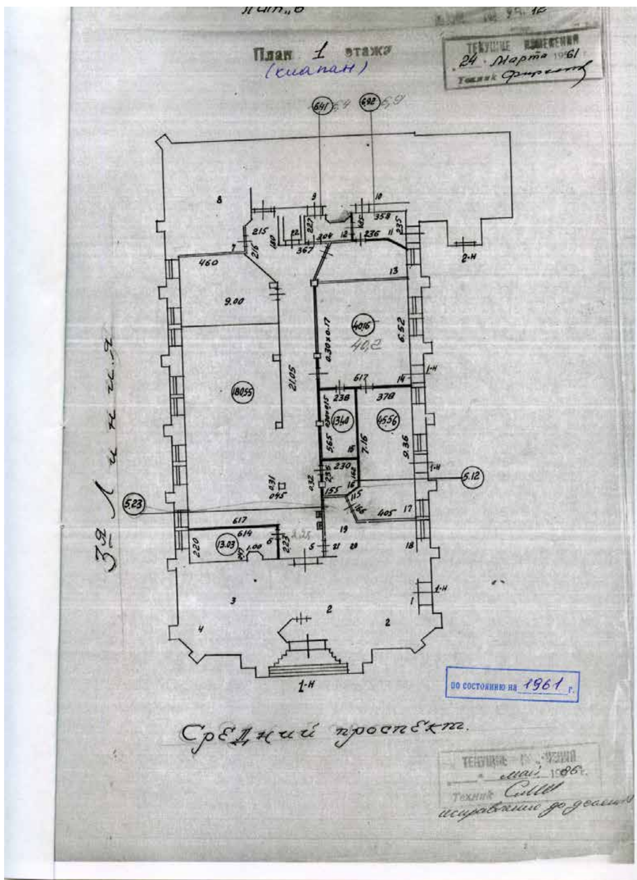
Илл. 63. План 1-го этажа. Архивные чертежи ПИБ здания по адресу: Санкт-Петербург, Средний пр. В.О., 18. 1961 г. (источник: СПб ГБУ «ГУИОН»).
