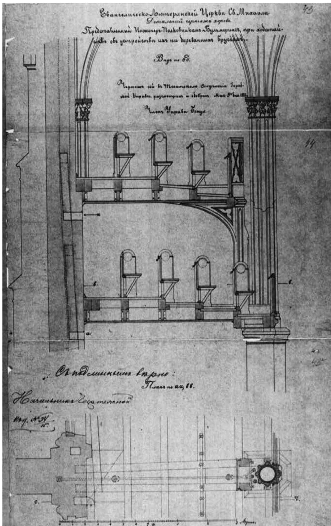
Илл. 28. Детальный чертеж хоров Евангелическо-Лютеранской Церкви Св. Михаила, представленный инженер-полковником Бульмеринг, при хоодатайствии об устройстве их на деревянных брусках. Вид по с-д. План по а-а, в-в. 1874 г. (источник: ЦГИА СПб: Фонд 513. Опись 102. Дело 2369).
