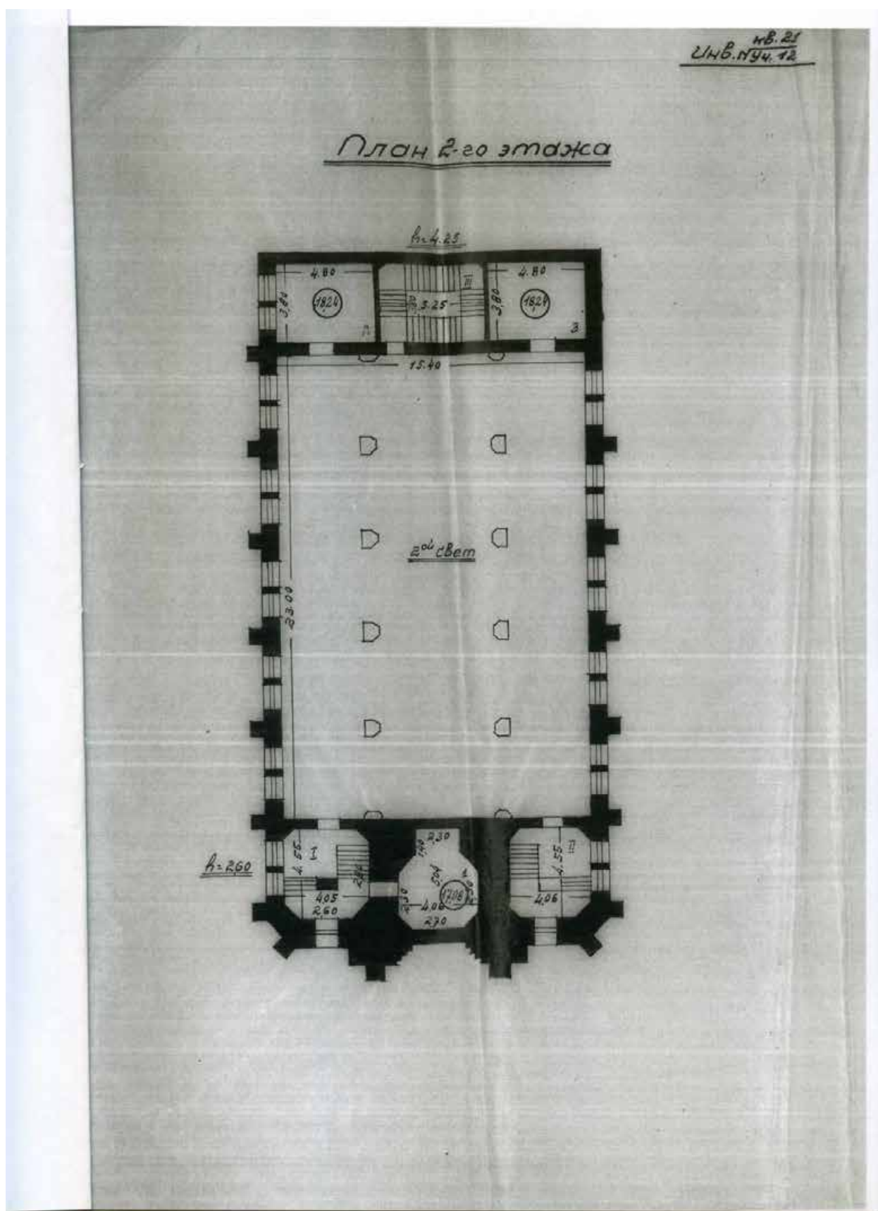
Илл. 54. План 2-го этажа. Архивные чертежи ПИБ здания по адресу: Санкт-Петербург, Средний пр. В.О., 18. 1947 г. (источник: СПб ГБУ «ГУИОН»).
