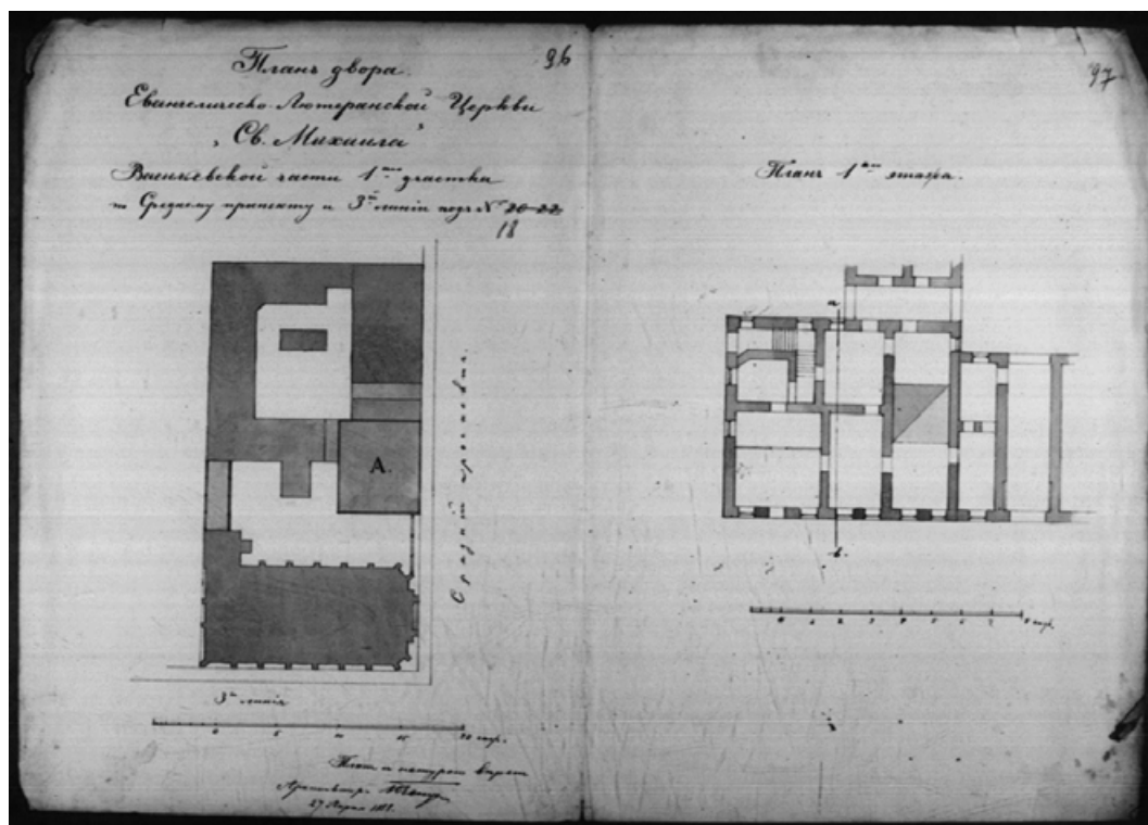
Илл. 47. План двора Евангелическо-Лютеранской Церкви Св. Михаила Васильевской части 1-го участка по Среднему проспекту и 3-й линии под № 18. План 1-го этажа. 1888 г. (источник: ЦГИА СПб: Фонд 513. Опись 102. Дело 2369).
