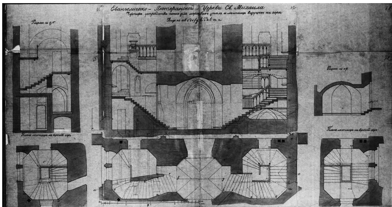
Илл. 37. Чертежи устройства покая для мертвых тел и лестниц, ведущих на хоры Евангелическо-Лютеранской Церкви Св. Михаила (источник: ЦГИА СПб: Фонд 513. Опись 102. Дело 2369).
