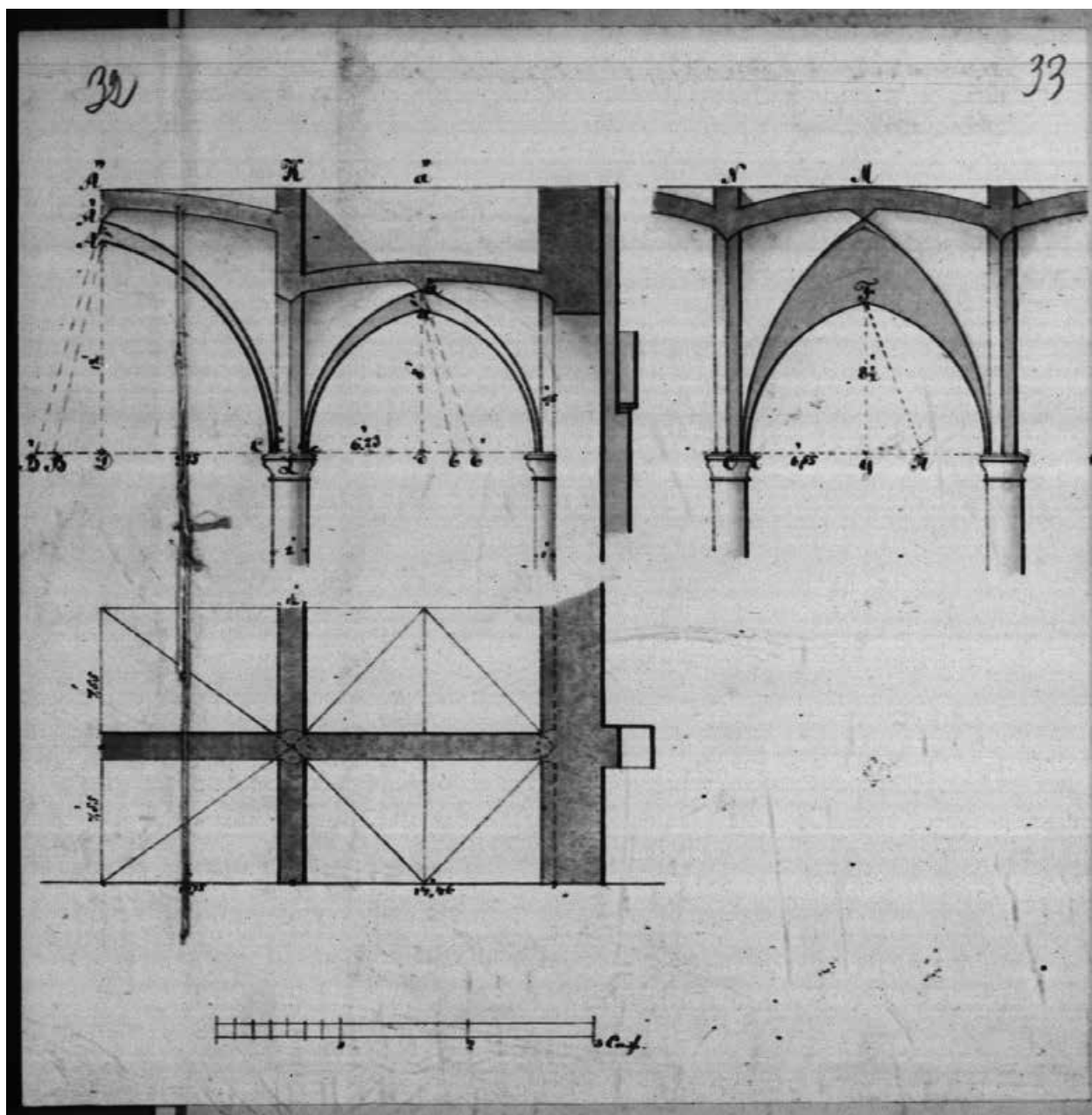
Илл. 25. Конструкции сводов. 1874 г. (источник: ЦГИА СПб: Фонд 513. Опись 102. Дело 2369).
