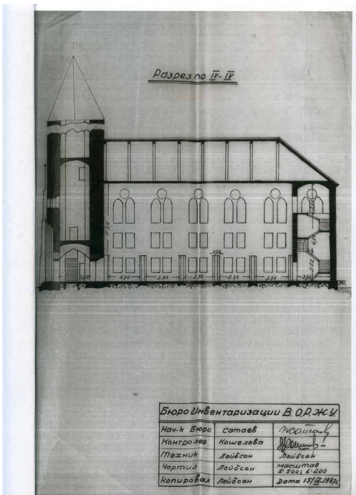
Илл. 58. Продольный разрез. Архивные чертежи ПИБ здания по адресу: Санкт-Петербург, Средний пр. В.О., 18. 1947 г. (источник: СПб ГБУ «ГУИОН»).
