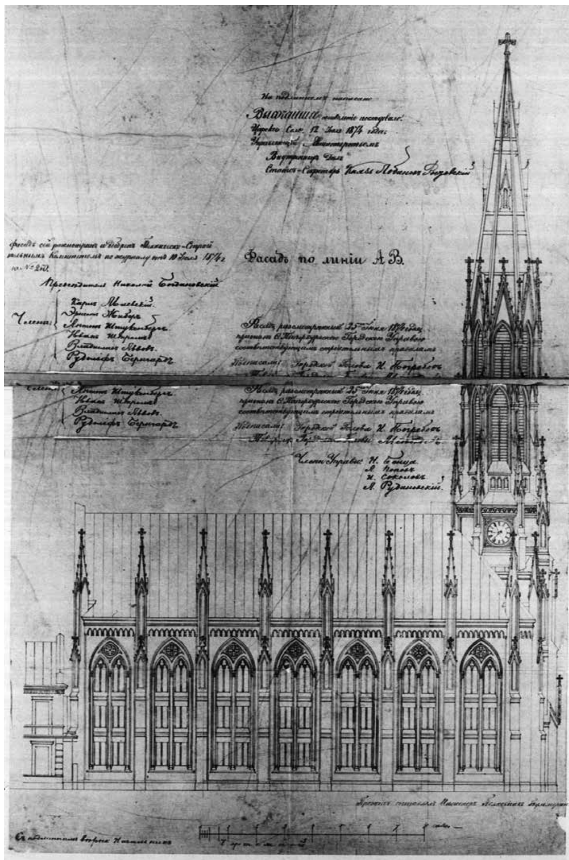
Илл. 26. Фасад по линии А-В. 1874 г. (источник: ЦГИА СПб: Фонд 513. Описание 102. Дело 2369).
