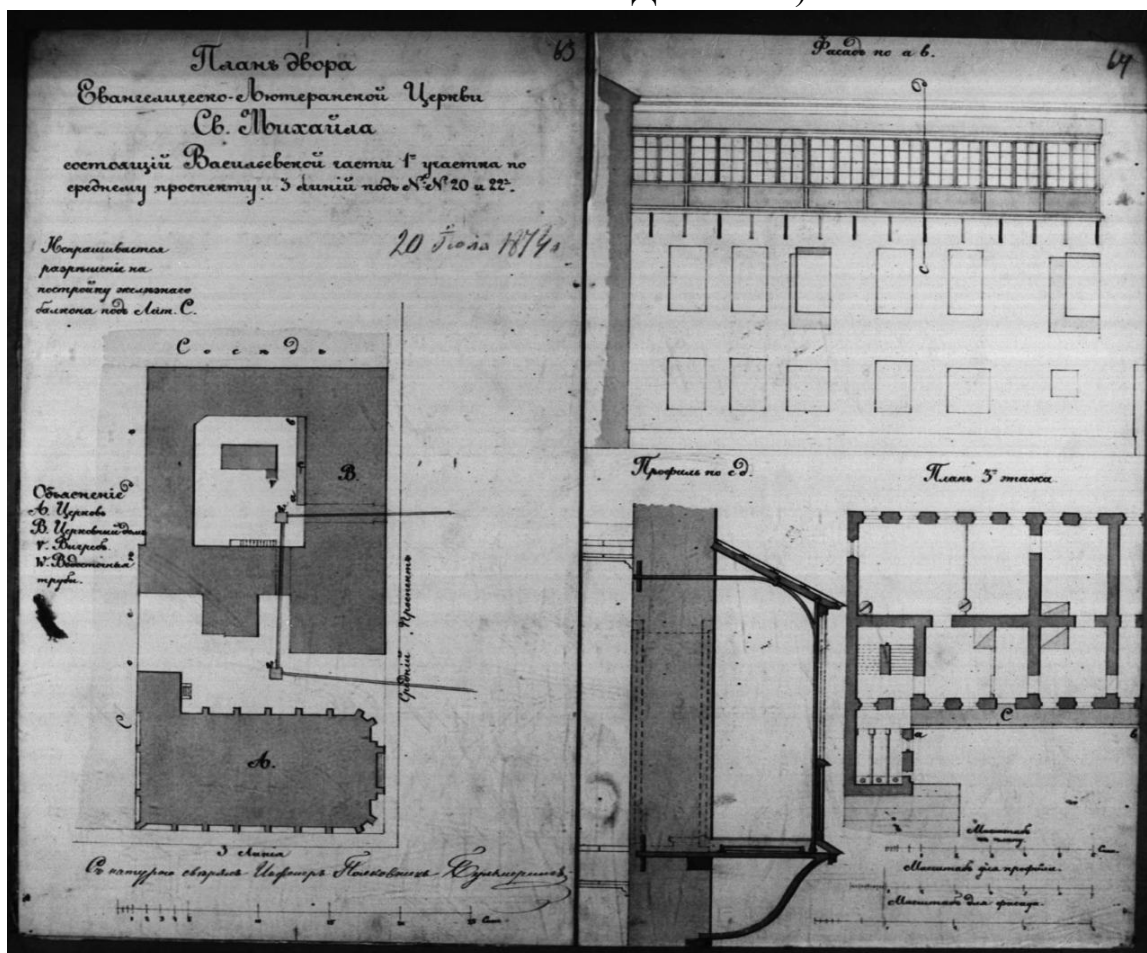
Илл. 36. План двора Евангелическо-Лютеранской Церкви Св. Михаила, состоящий Васильевской части 1-го участка по Среднему проспекту и 3-й линии под №№ 20 и 22. Фасад по а-в. Профиль по с-д. План 3-го этажа. 1874 г. (источник: ЦГИА СПб: Фонд 513. Опись 102. Дело 2369).
