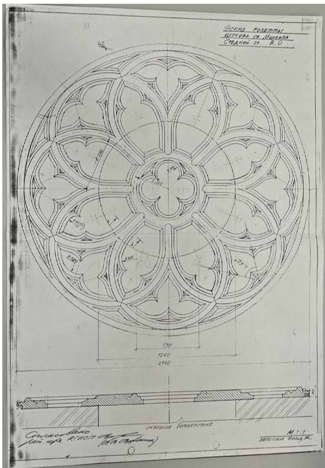
Илл. 72. Проект устройства розетки церкви Св. Михаила. 1999 г. (источник: Местная Религиозная Организация «Русский Евангелическо-Лютеранский Приход Святого Михаила»).
