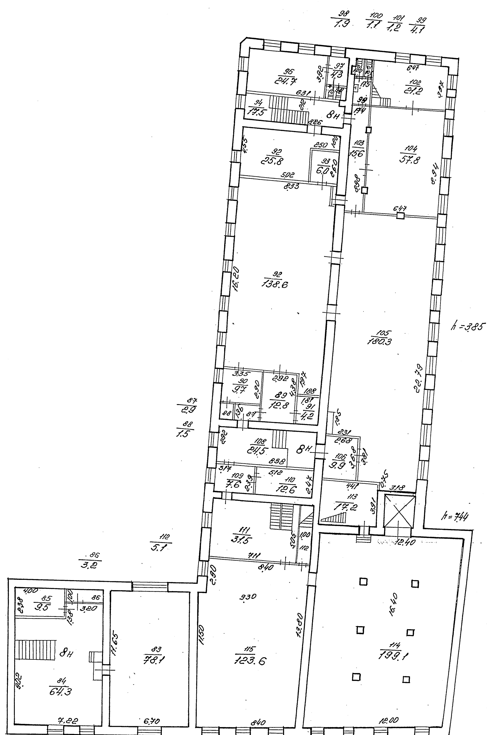
План 3 этажа.
