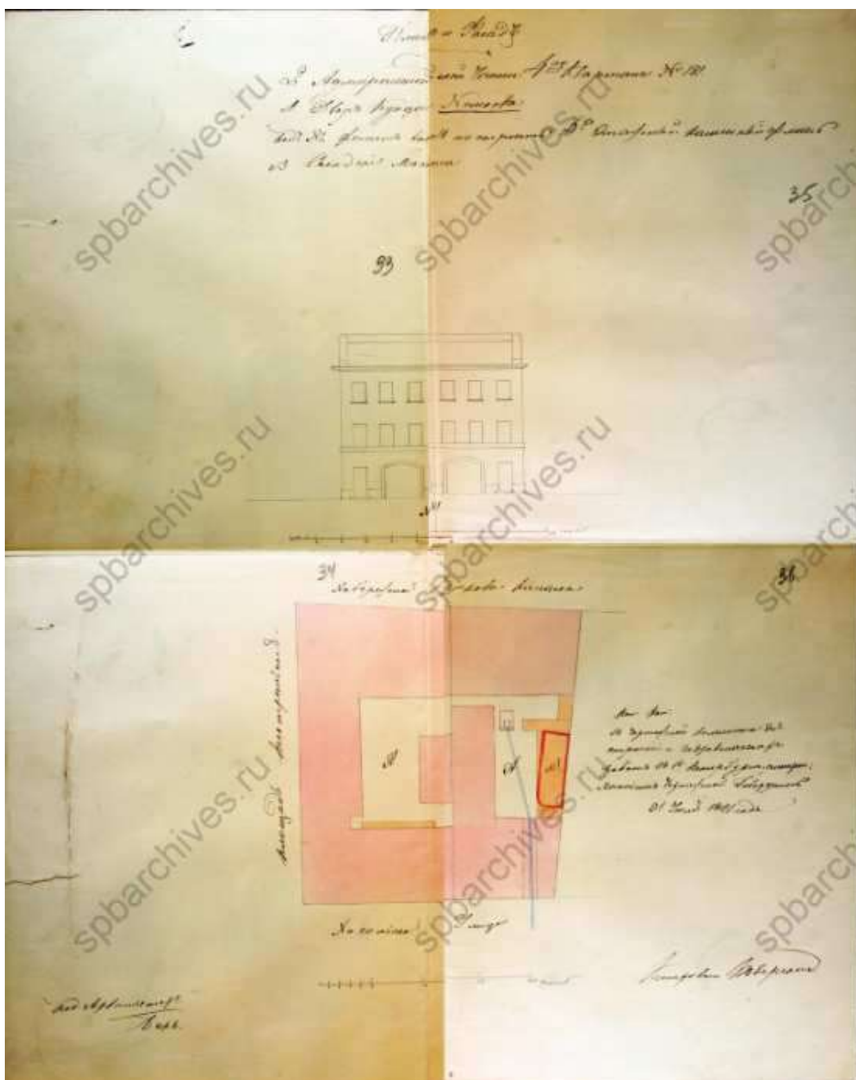
28. План и фасад дома купца Ивана Немкова, 1841 г. Архитектор: Гек. ЦГИА СПб. Фонд 513. Опись 102. Дело 3352
