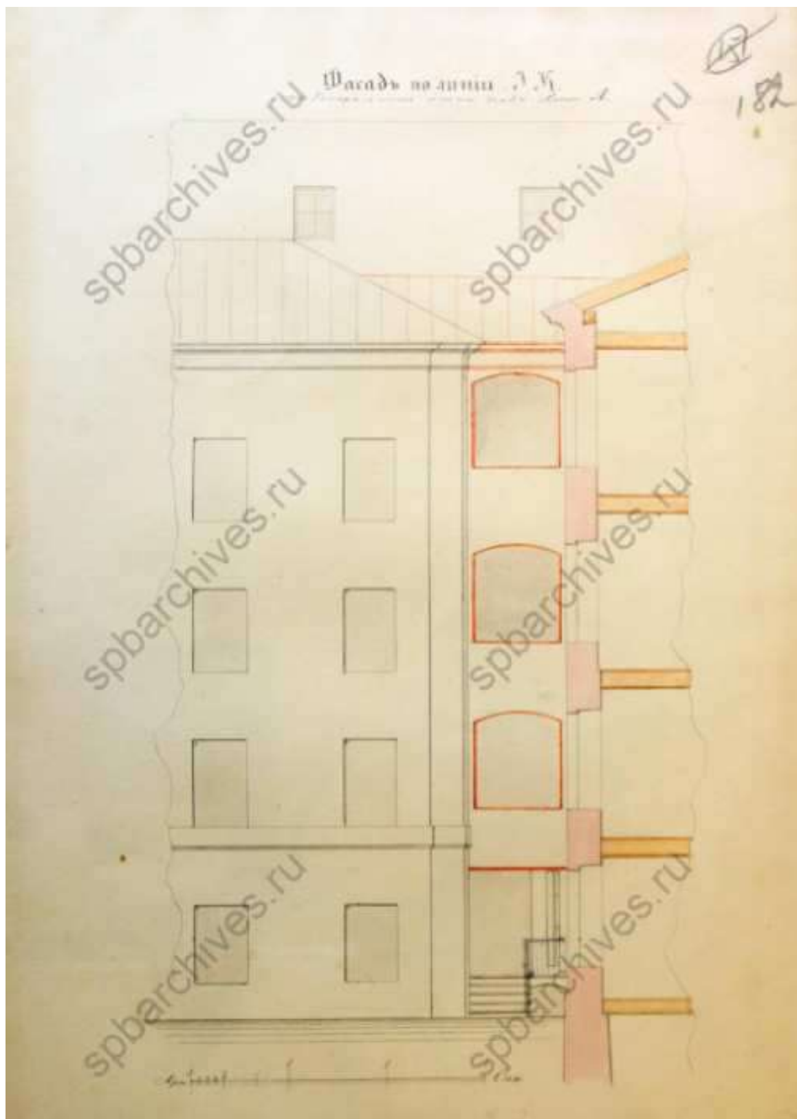
89. Фасад по линии JK. ЦГИА СПб. Фонд 513. Опись 102. Дело 3352
