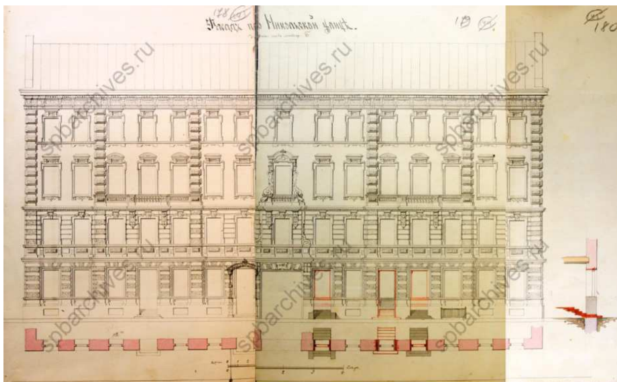
86. Фасад по Никольской улице. ЦГИА СПб. Фонд 513. Описание 102. Дело 3352
