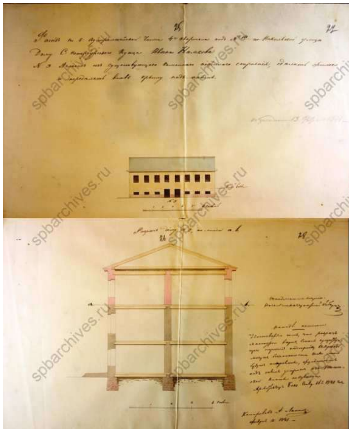
25. Фасад и разрез дома купца Ивана Немкова, 1841 г. ЦГИА СПб. Фонд 513. Опись 102. Дело 3352
