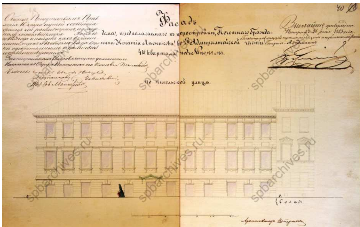
30. Фасад предполагаемого к постройке дома Игнатия Лесникова, 1853 г. Архитектор: Штрот. ЦГИА СПб. Фонд 513. Опись 102. Дело 3352
