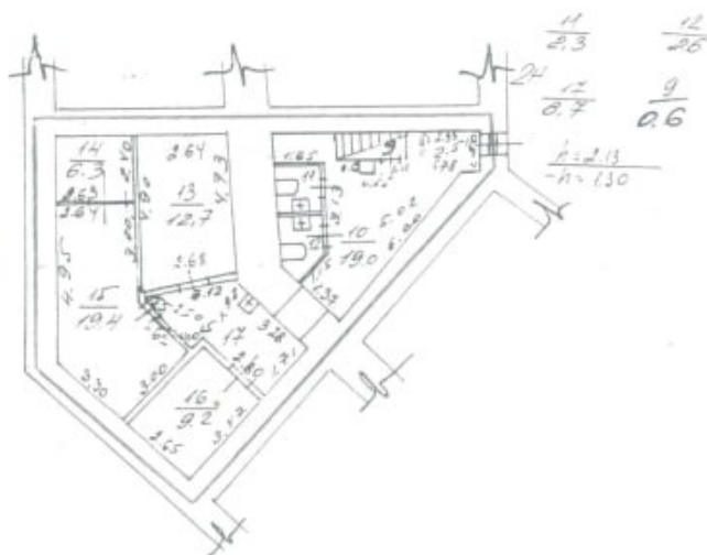
План подвала
