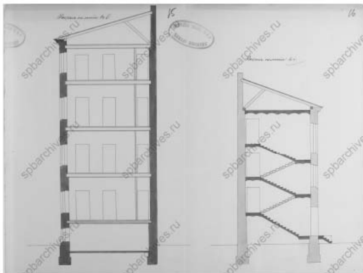
5. Разрез по линии к1. 1896 г. // Источник: ЦГИА СПб Ф. 513 Оп. 102 Д. 9962 Лл. 15-16.
