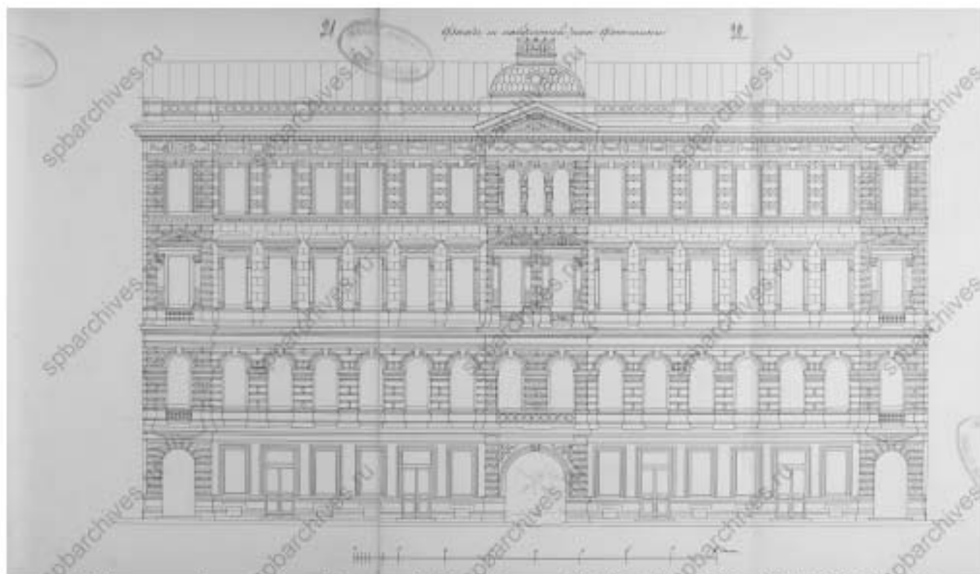
7. Фасад по набережной реки Фонтанки. 1896 г. // Источник: ЦГИА СПб Ф. 513 Оп. 102 Д. 9962 Лл. 21-23.
