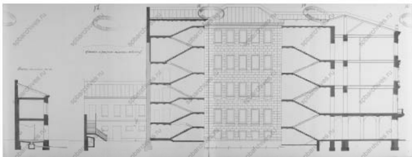
6. Разрез по линии m-l. Фасад и разрез по линии a-b-c-d-e-f. 1896 г. // Источник: ЦГИА СПб Ф. 513 Оп. 102 Д. 9962 Лл. 17-20.
