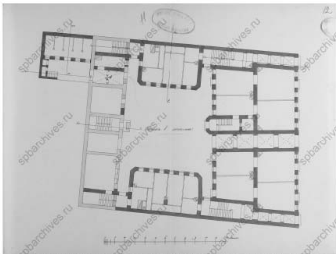
3. План 1 этажа. 1896 г. // Источники: ЦГИА СПб ЦГИА СПб Ф. 513 Оп. 102 Д. 9962 Лл. 11-12.
