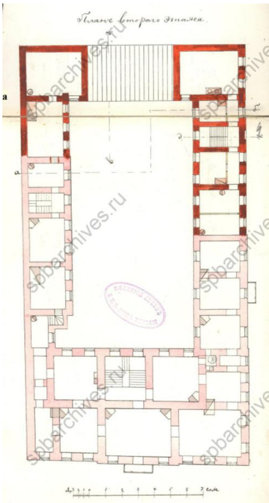
17. Детальные планы подвального, первого, второго этажей.
