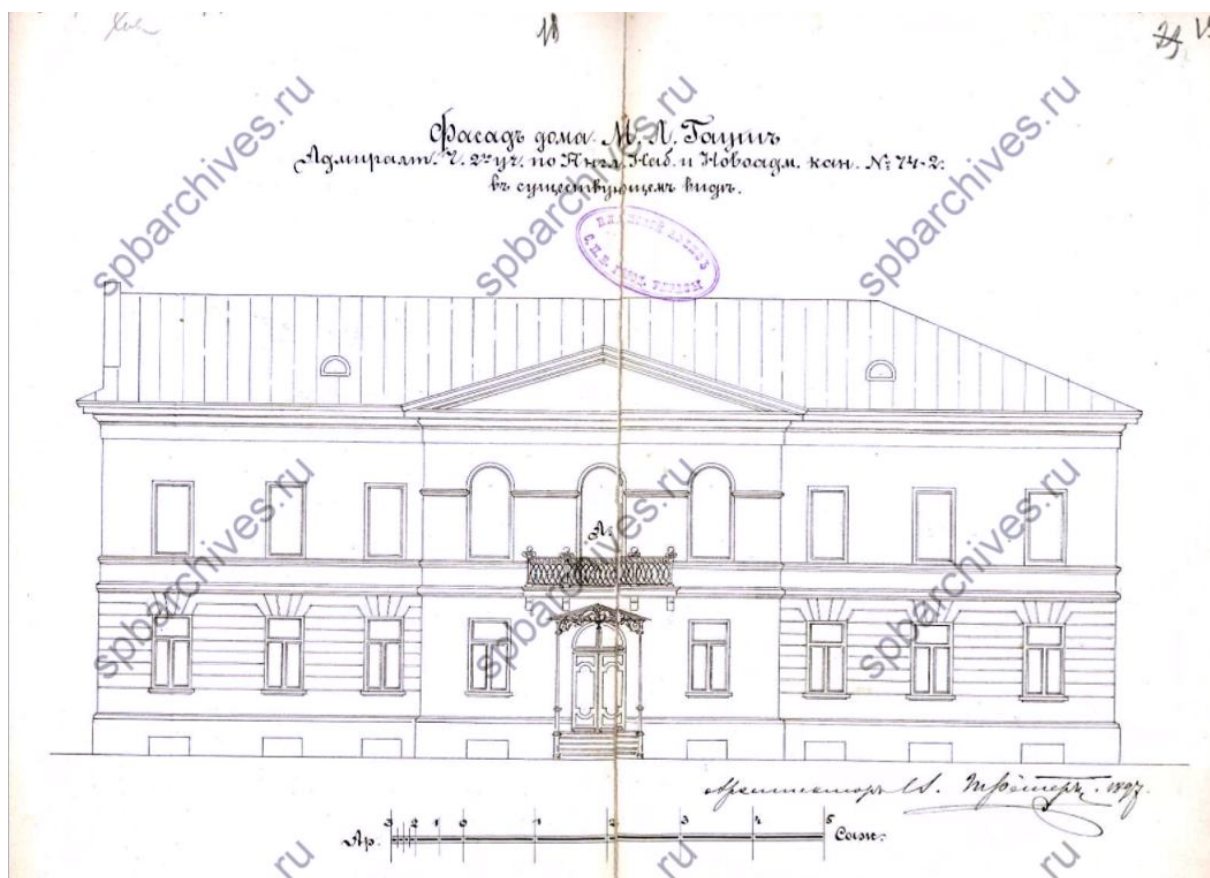
26. Лицевой фасад дома по Английской набережной в существующем виде. 1897 г. Арх. В.А. Шрертер. ЦГИА СПб. Ф.513. Оп.102. Д. 50. Л.Л. 18,19.
