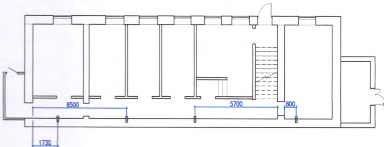
План первого этажа
