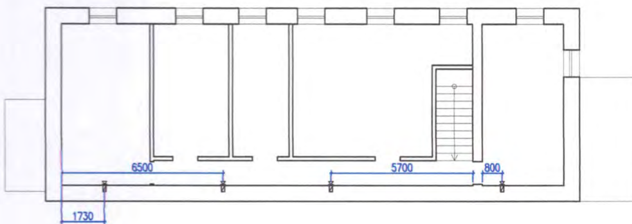
План второго этажа
