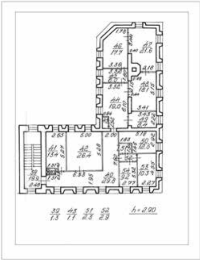
План 3 этажа
