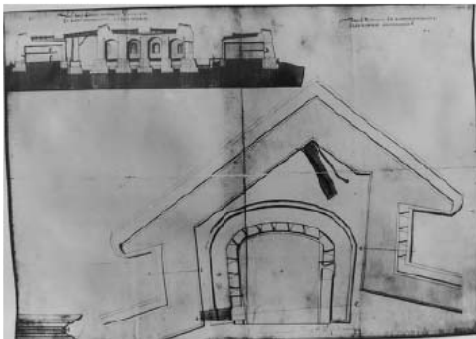
Илл.13. План бастиона с кавальером и разрез по кавальеру и фангам бастиона Анны Иоанновны. РГА ВМФ. Ф. 3л. Оп. 34, Д. 2523. Л. 1 (1748 г.) Копия: КТИОП, п. 90-17 (1) Н 1088.
