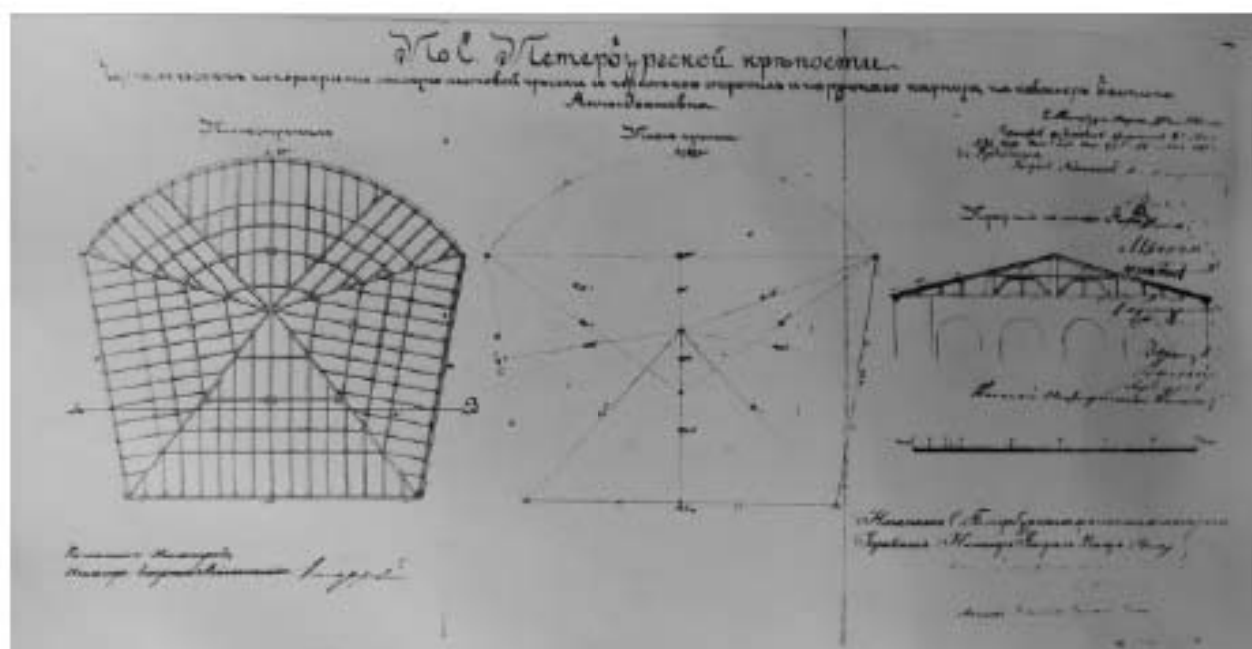
Илл.42. «По Санкт-Петербургской крепости. Чертеж к смете на перекрытие железно листовою крыши с переменной стропил и наружного карниза на кавальере Бастиона Анны Иоанновны. План стропил, план крыши, профиль по линии АБ». 1885 г. Копия: КГИОП, п. 90-17 (1) Н-1088.
