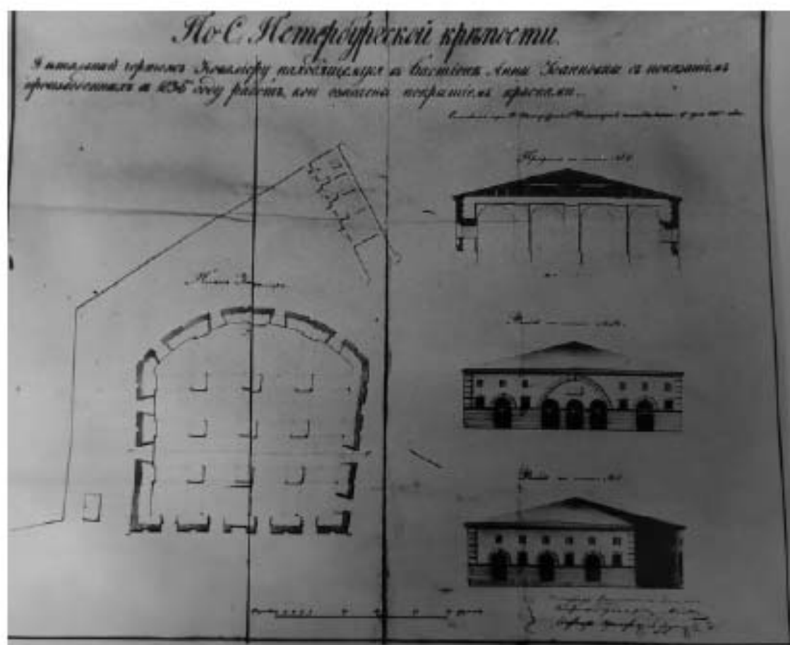
Илл. 36. План кавалер. Разрез по кавалеру с показанием конструкций новой крыши. Новое оформление южного и восточного фасадов кавалера. 1836 г. РГА ВМФ. Ф 3л, Оп. 34, Копия: КГИОП, п. 90-17 (1) Н-1088.
