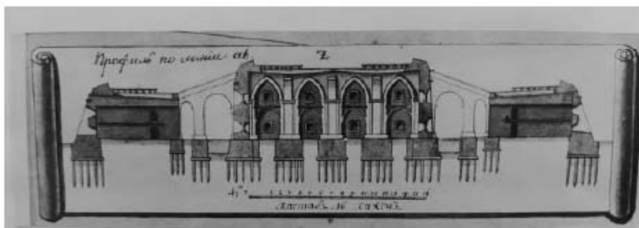
Илл.10. «Санктпетербурх со опробованными рavelинами и контргардами». Проект 1732 г. Часть чертежа X.-Б. Миниха. Разрез по кавальеру и флангам бастиона. Копия архив ГМИ СПб I- Ф-12453-п, ЛПР. нег.61159 а.
