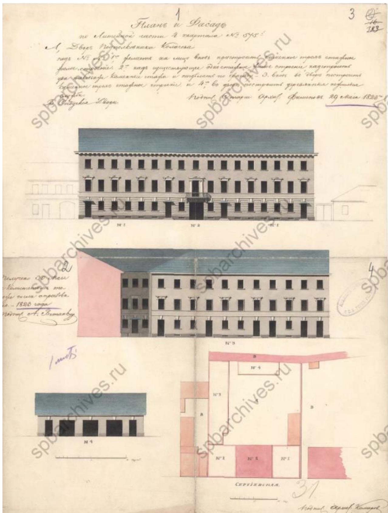
Илл. 5. Чертежи генплана и фасадов дома, разработанного арх. А.З. Комаровым.
