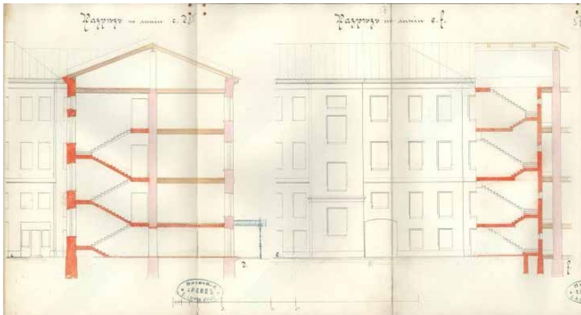
34. Разрез по линии с.д. Разрез по линии е.ф. 1881 г. // Источник: ЦГИА СПб фонд 513, опись 102, дело 213, листы 55-57. Чертежи дома на участке, принадлежавшем В.И.Струбинскому, А.И.Трейбергу по Невскому пр., 11.
