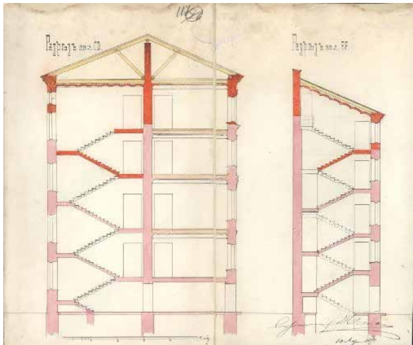
54. Разрезы по СД и ЕФ. Подпись архитектора Л. Бенуа. 1898 г. // Источник: ЦГИА СПб фонд 513, опись 102, дело 213, листы 117-118. Чертежи дома на участке, принадлежавшем В.И.Струбинскому, А.И.Трейбергу по Невскому пр., 11.
