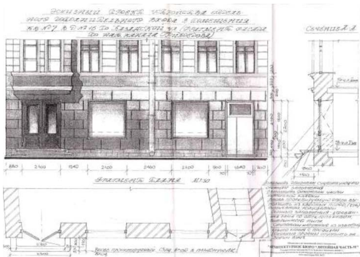
31. Эскизный проект устройства дополнительного отдельного входа в кв. №7, выполненный ООО «Архитектурное бюро «Литейная часть – 91». Архив КГИОП.
