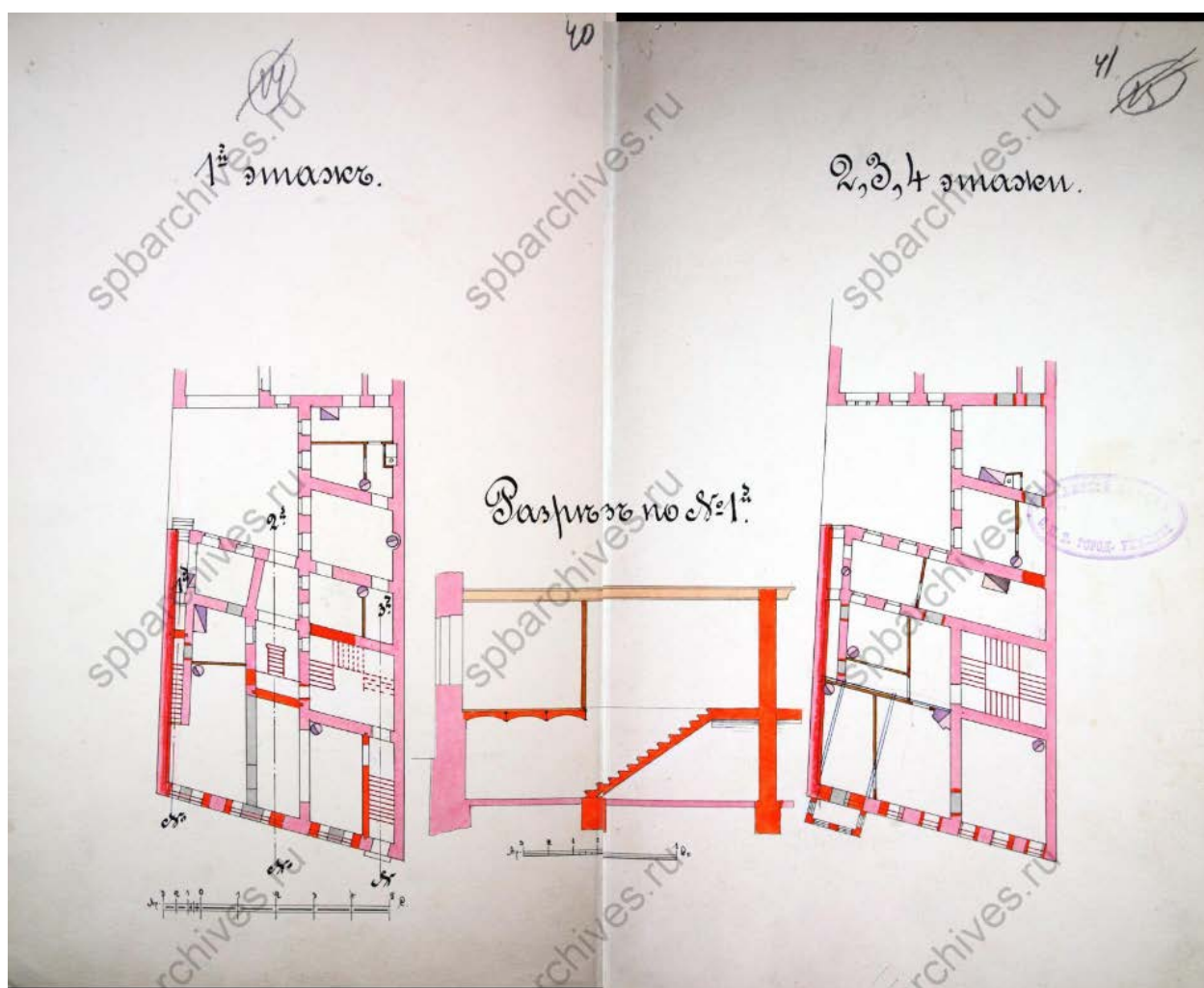
20. Чертежи поэтажных планов. Инж. Н. Архангельский. 1899 г. ЦГИА СПб. Фонд 513. Опись 102. Дело 3291. Лл. 40-41
