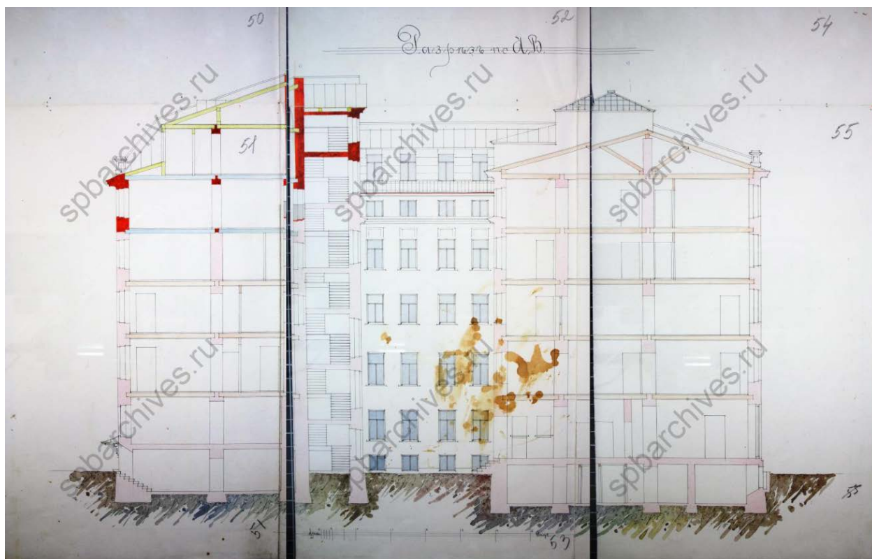
22. Чертеж разреза дома С.М. Литвинова. 1905 г. ЦГИА СПб. Фонд 513. Опись 102. Дело 3291. Лл. 50-54
