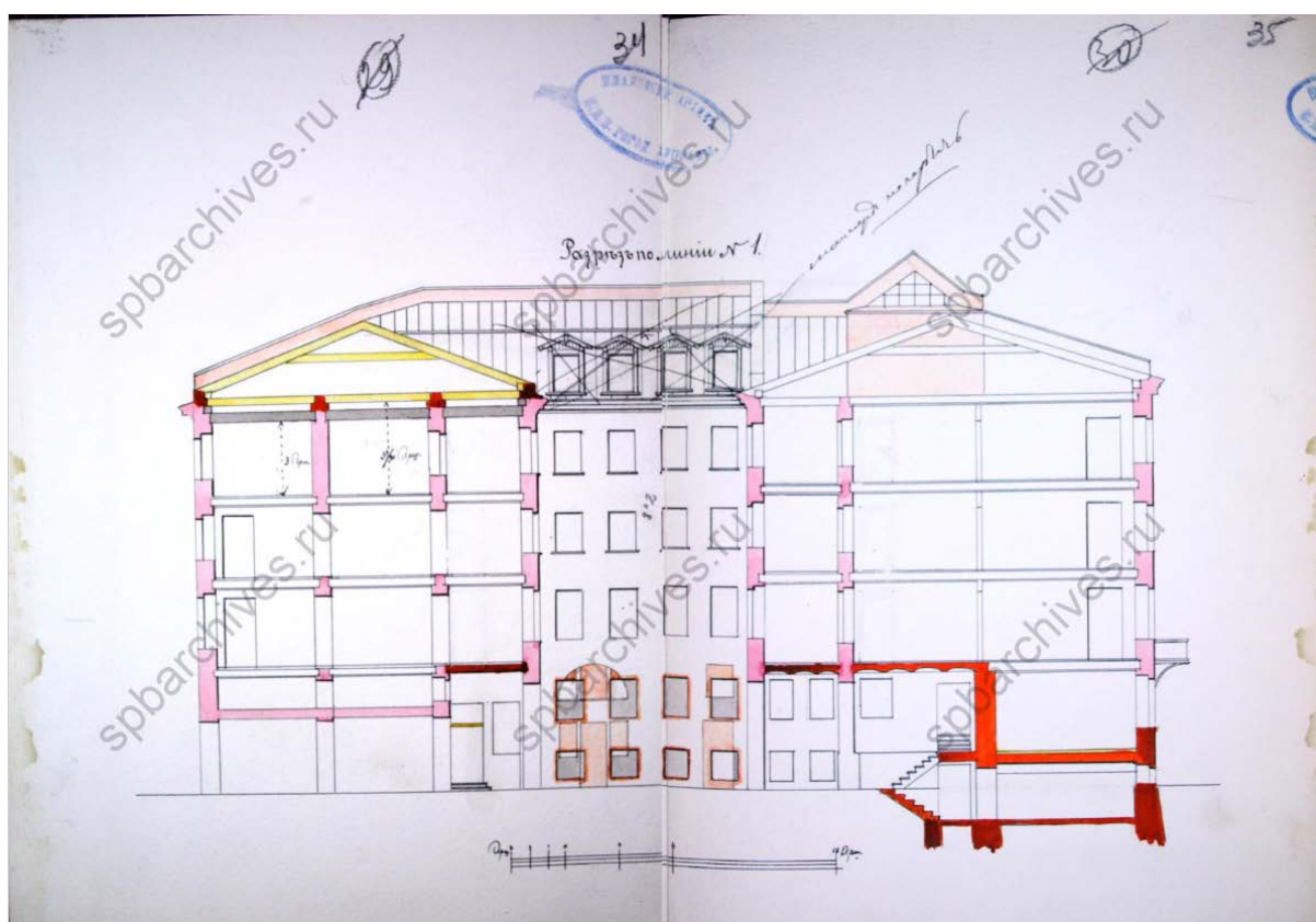
18. Чертеж разреза дома С.М. Литвинова. 1896 г. ЦГИА СПб. Фонд 513. Опись 102. Дело 3291. Лл. 34-35
