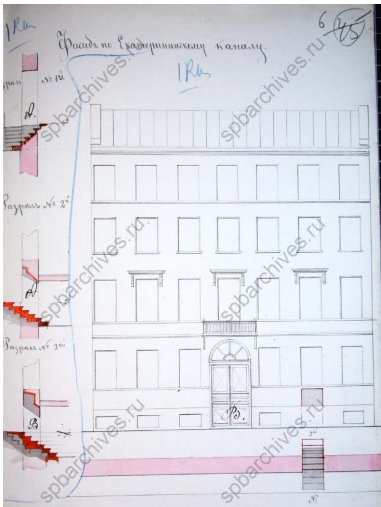
8. Чертеж фасада по Екатерининскому каналу. 1847 г. ЦГИА СПб. Фонд 513. Опись 102. Дело 3291. Л. 6
