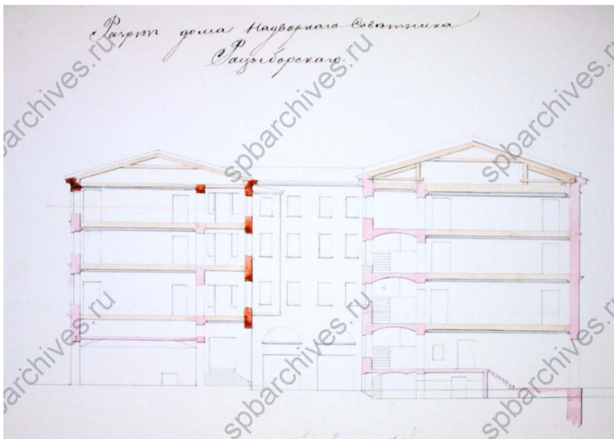
10. Разрез дома надворного советника Рациборского. 1847 г. ЦГИА СПб. Фонд 513. Опись 102. Дело 3291. Л. 8
