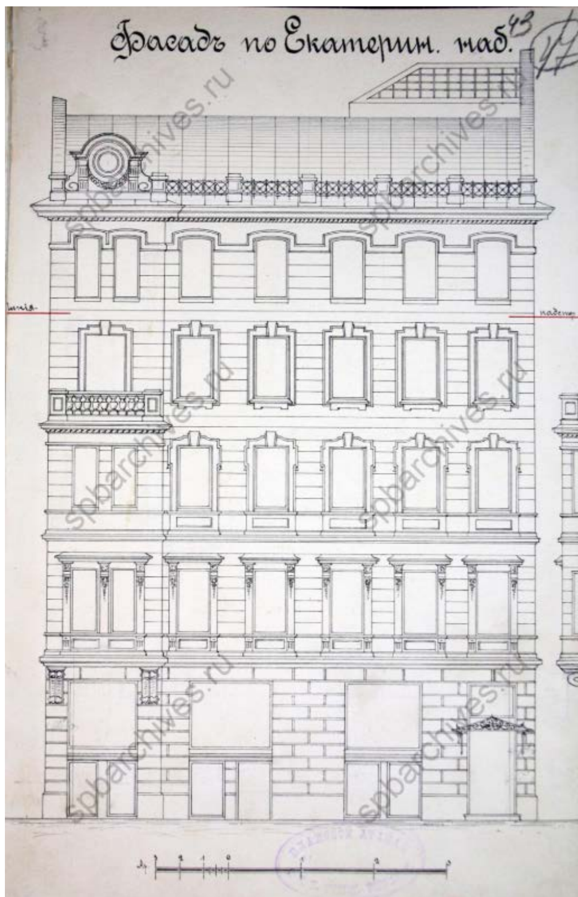
21. Чертеж фасада по Екатерининской наб. Инж. Н. Архангельский. 1899 г. ЦГИА СПб. Фонд 513. Опись 102. Дело 3291. Л. 43.
