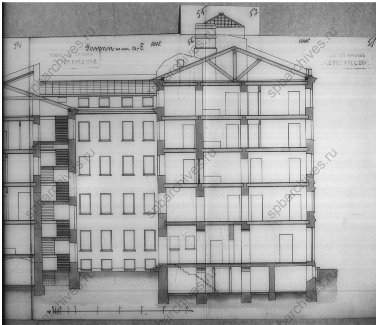
27. Чертеж разреза дома М.Т. Литвиновой. 1910 г. ЦГИА СПб. Фонд 515. Опись 4. Дело 867. Лл. 54-58
