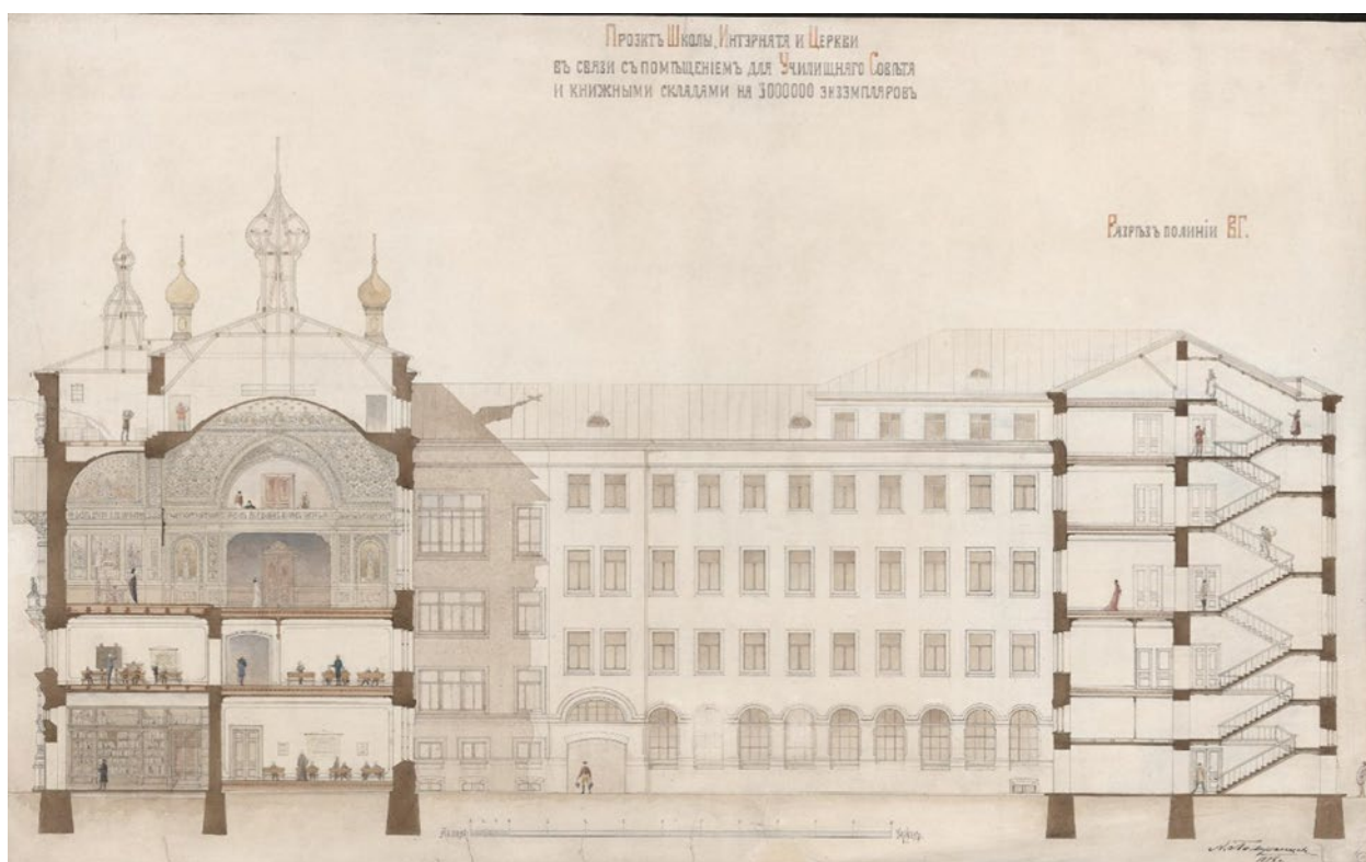
Илл. 26. Померанцев А.Н. Проект школы, интерната, церкви и книгохранилища. 1897 (НИМ РАХ. КП-176/301. А-20395)
