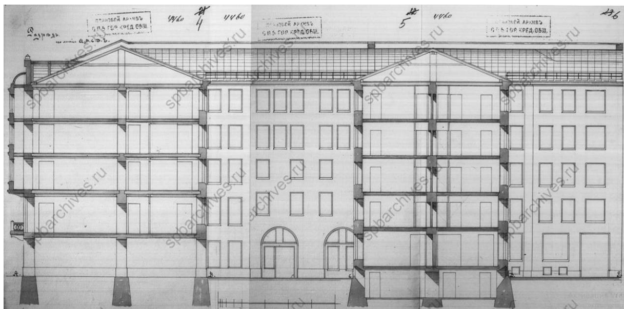
29. Продольный разрез по линии А-В-С-Д-Е. Фиксационный чертеж.
