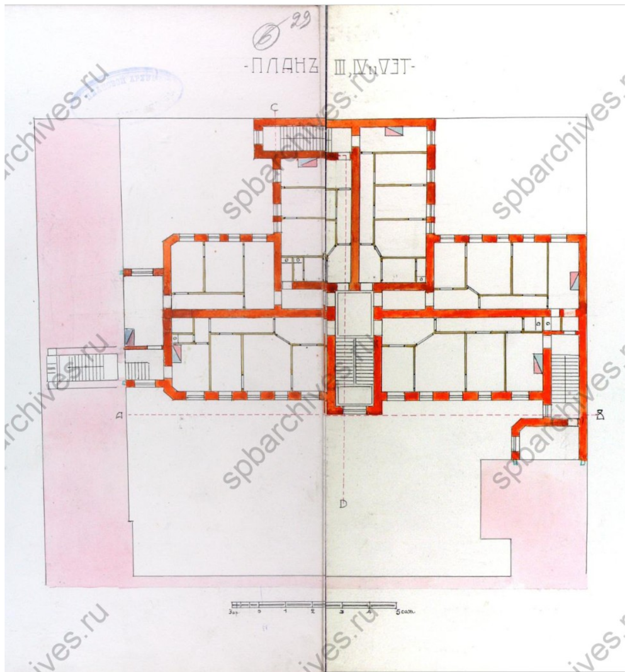
27. Проект поперечного дворового флигеля: план 3, 4 и 5 этажей. Арх. П.Ю. Сюзор. 1906 г.
