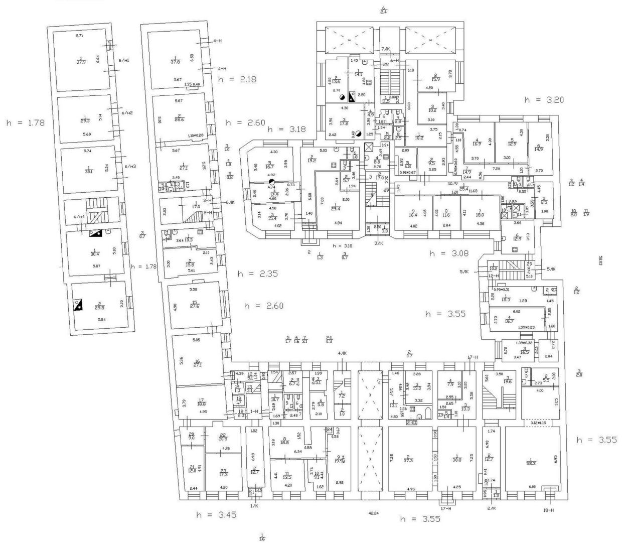
план 1 этаж
