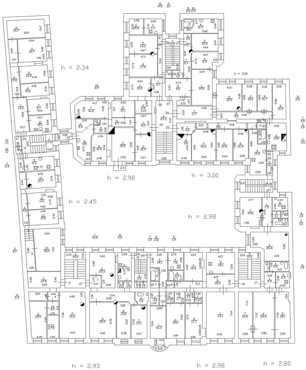
ПЛАН 3 ЭТАЖ
