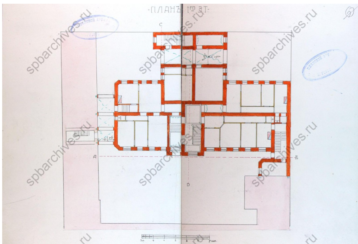
25. Проект поперечного дворового флигеля: план 1 этажа.
