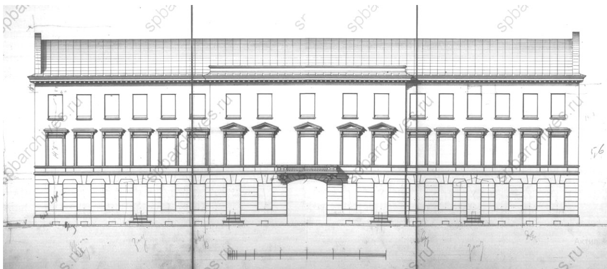
10. Фиксационный чертеж лицевого фасада дома Трухмановых по Большой Мещанской ул. 1879(?) г.
