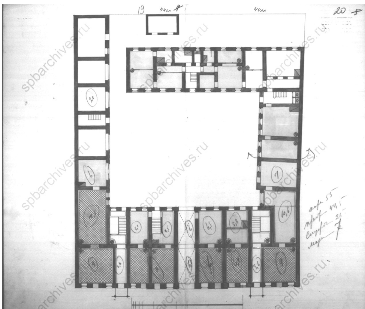
11. Фиксационный план 1 этажа дома Трухмановых. 1879(?) г.
