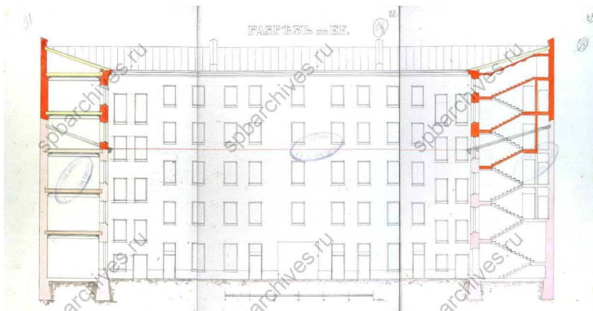
16. Проект надстройки дома: дворовый фасад лицевого дома и разрезы флигелей по линии Е-Е.
