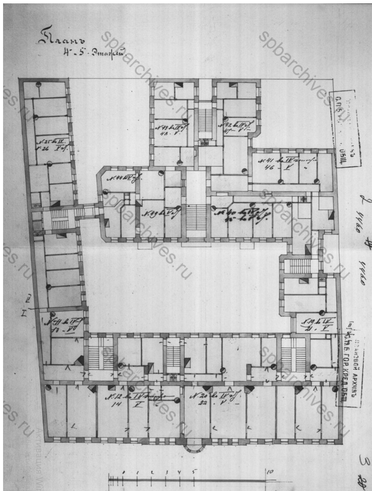
34. План 4 и 5 этажей. Фиксационный чертеж.
