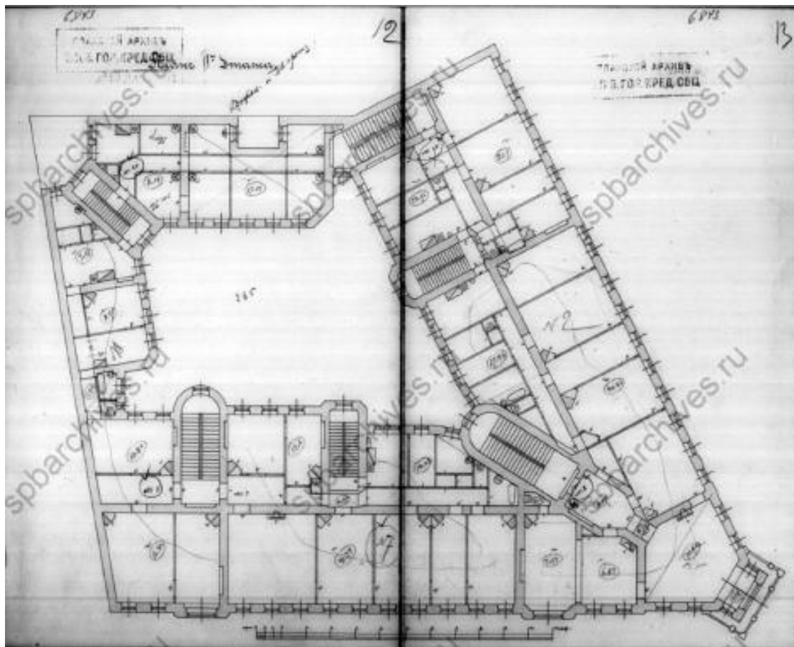
11. План 2-го этажа. 1911 г. // ЦГИА СПб. Ф. 515. Оп. 4. Д. 2194.
