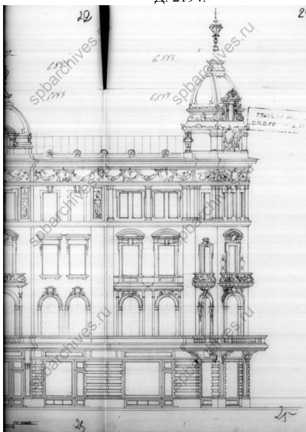
14. Фасад по Каменноостровскому проспекту. Фрагмент. 1911 г. // ЦГИА СПб. Ф. 515. Оп. 4 Д. 2194.
