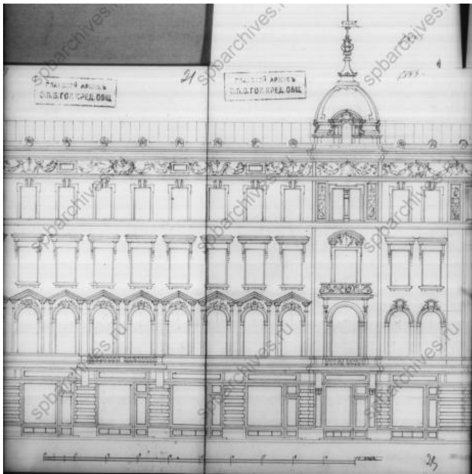
13. Фасад по Каменноостровскому проспекту. Фрагмент. 1911 г. // ЦГИА СПб. Ф. 515. Оп. 4 Д. 2194.
