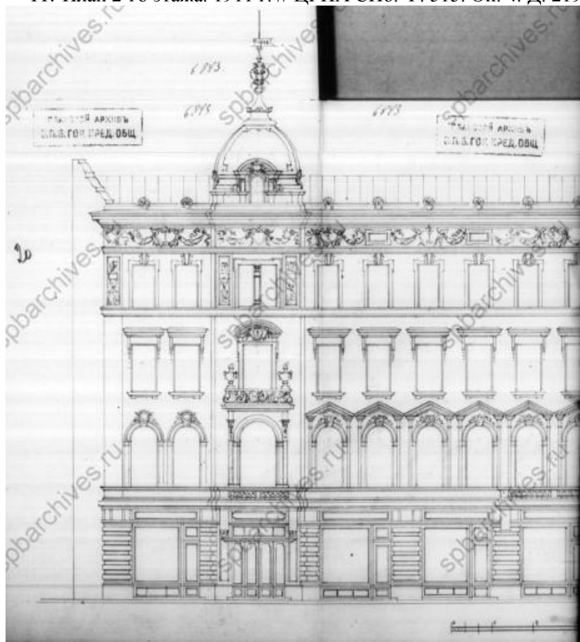
12. Фасад по Каменноостровскому проспекту. Фрагмент. 1911 г. // ЦГИА СПб. Ф. 515. Оп. 4. Д. 2194.
