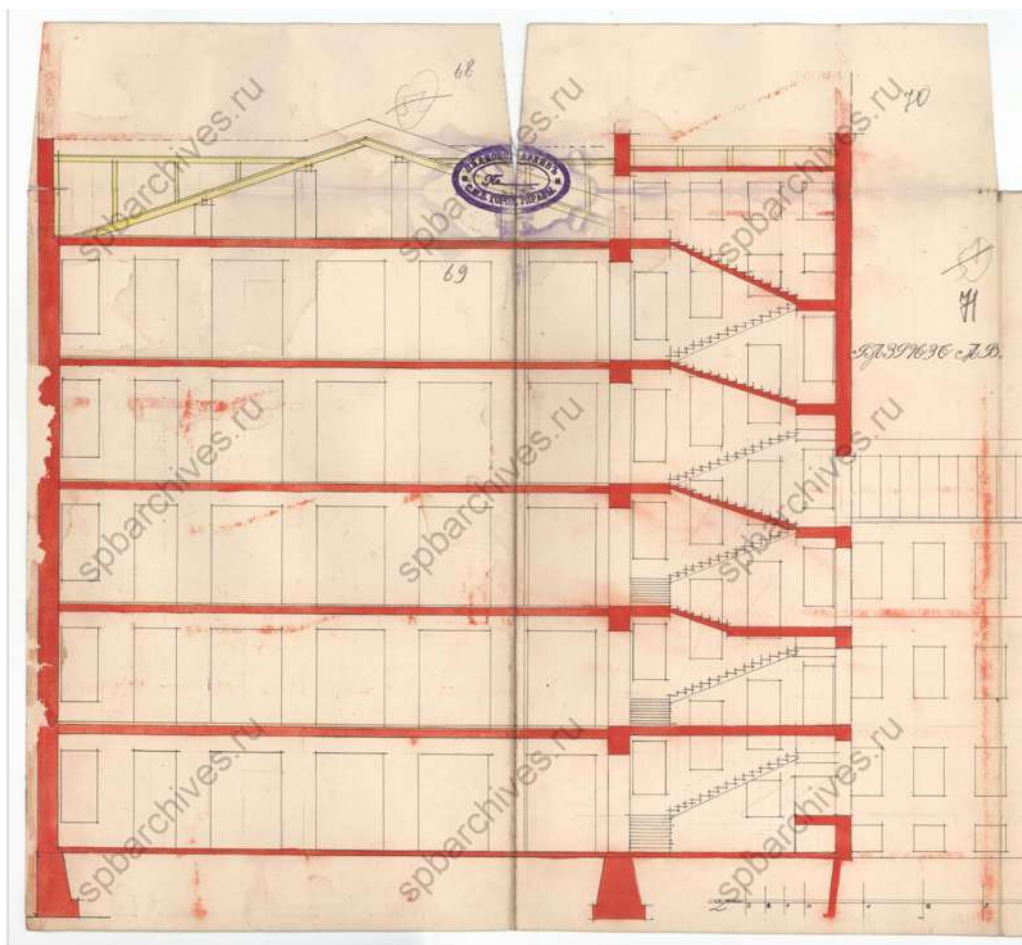
48. Разрез. 1913 г. ЦГИА СПб, ф.513, оп.102, д.1670
