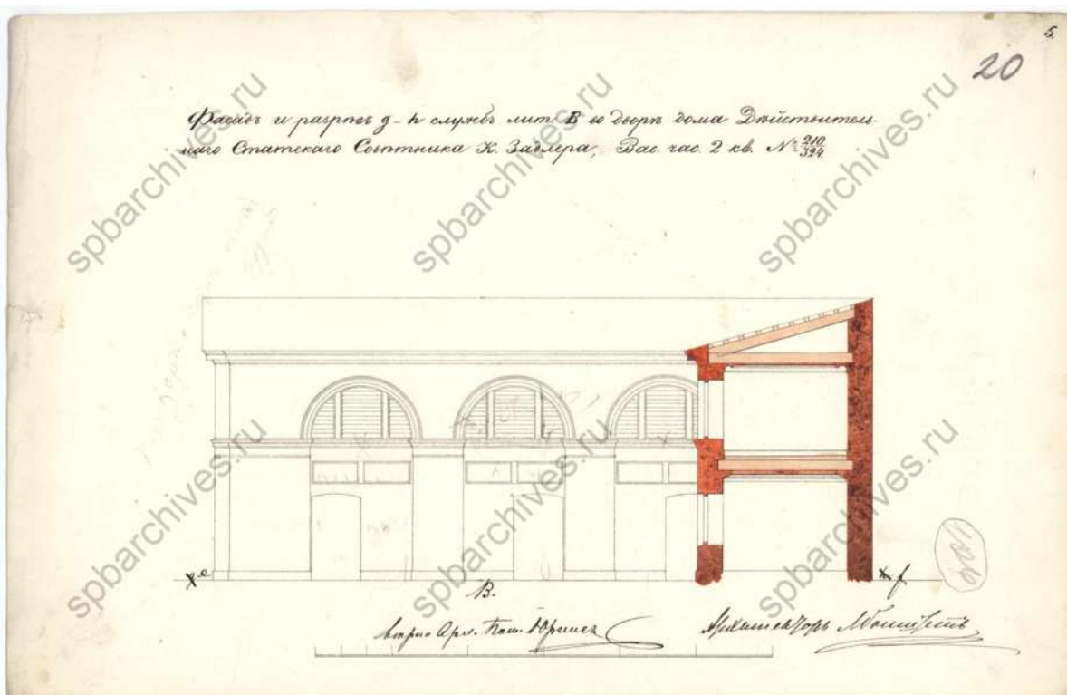
21. Фасад и разрез служб. 1860 г. ЦГИА СПб, ф.513, оп.102, д.1670
