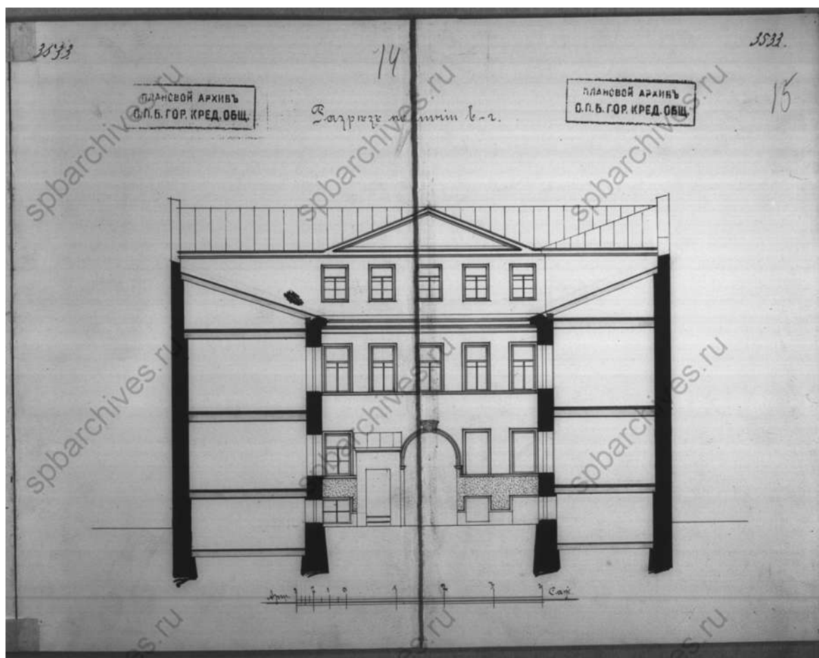
79. Разрез. 1910 г. ЦГИА СПб, ф. 515, оп. 4, д. 2790
