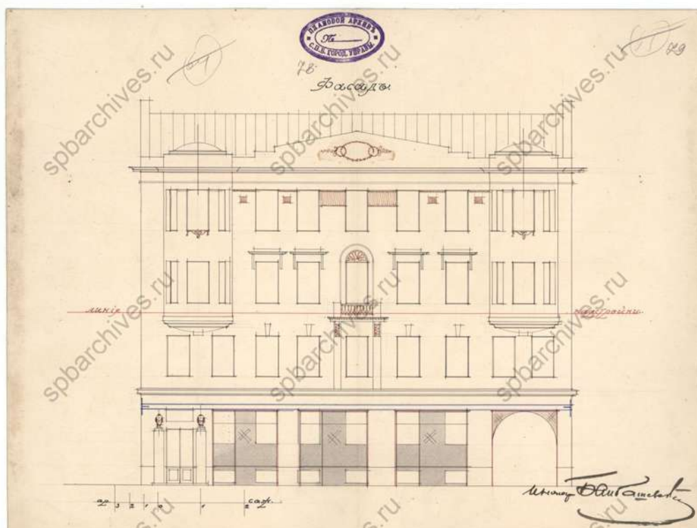
51. Лицевой фасад в предполагаемом виде. 1913 г. ЦГИА СПб, ф.513, оп.102, д.1670
