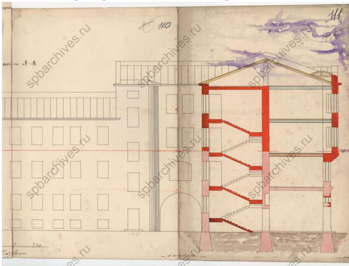
62. Разрез и фасад. 1913 г. ЦГИА СПб, ф.513, оп.102, д.1670
