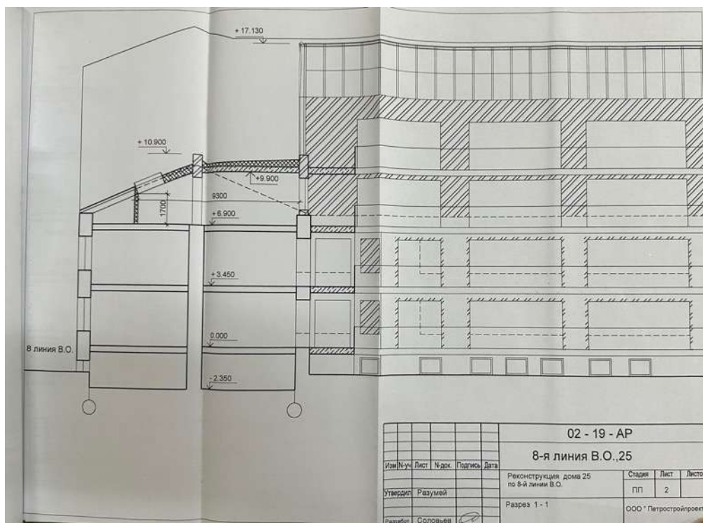
92.Разрез. Объемно-пространственное и архитектурное решение реконструкции дома 25 по 8 линии В.О. СПб, 2002 г. Архив КГИОП П 1500-П ин. 1021
