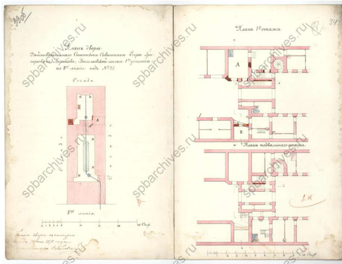
29. План двора Егора Григорьевича Воробьева и планы этажей. 1878 г. ЦГИА СПб, ф.513, оп.102, д.1670
