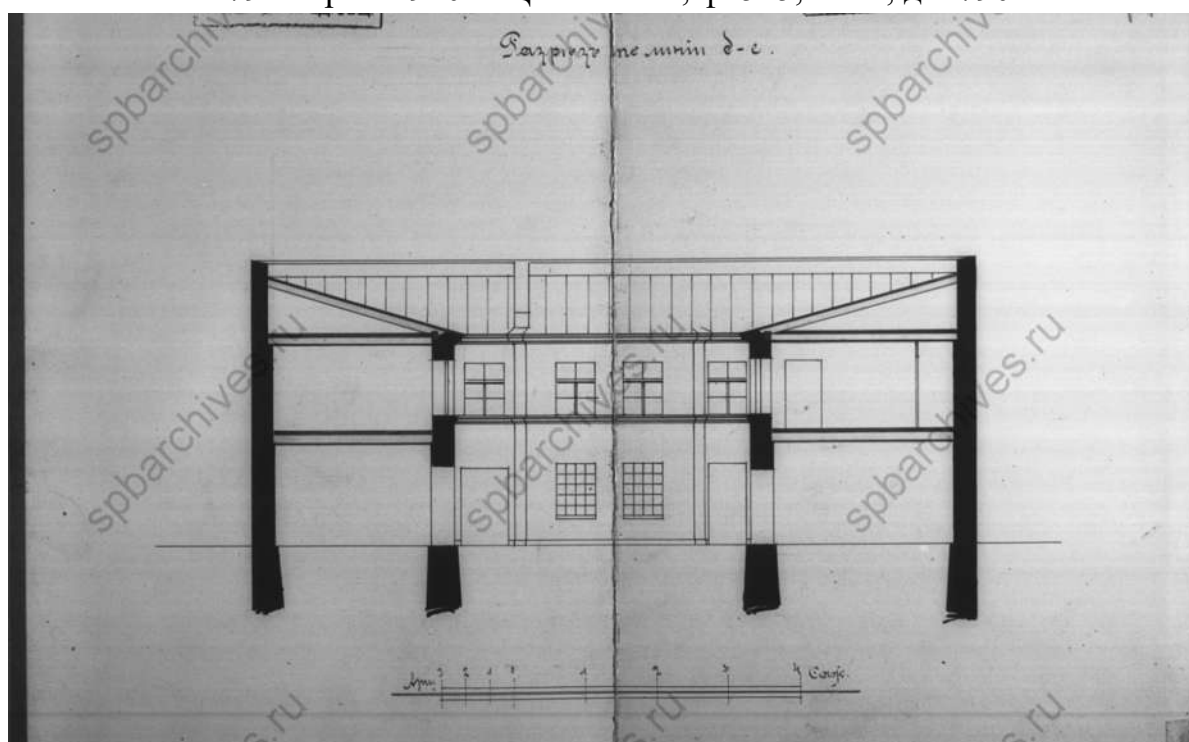
80. Разрез. 1910 г. ЦГИА СПб, ф. 515, оп. 4, д. 2790
