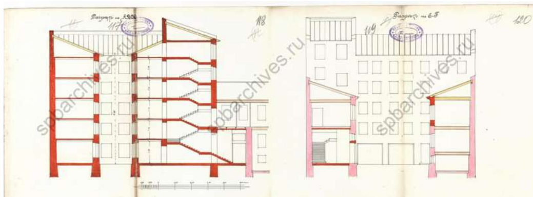
68. Разрезы. 1914 г. ЦГИА СПб, ф.513, оп.102, д.1670
