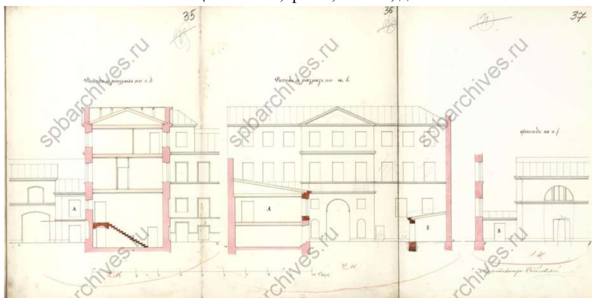
30. Фасады и разрезы. 1878 г. ЦГИА СПб, ф.513, оп.102, д.1670
