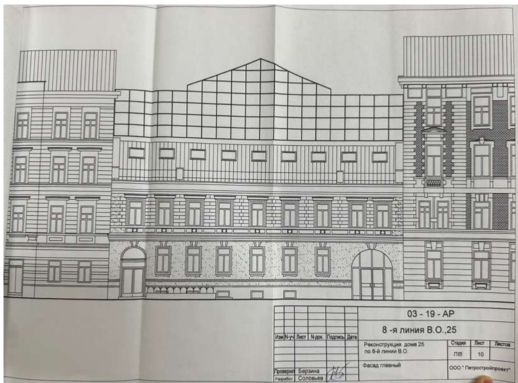
117. Фасад главный. Объемно-пространственное и архитектурное решение реконструкции дома 25 по 8 линии В.О. СПб, 2003 г. Архив КГИОП П 1500-Л ин. 1025
