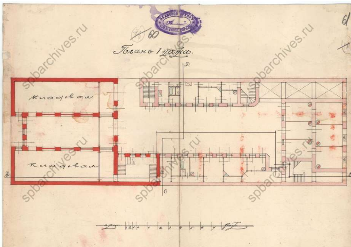
44. План первого этажа. 1913 г. ЦГИА СПб, ф.513, оп.102, д.1670
