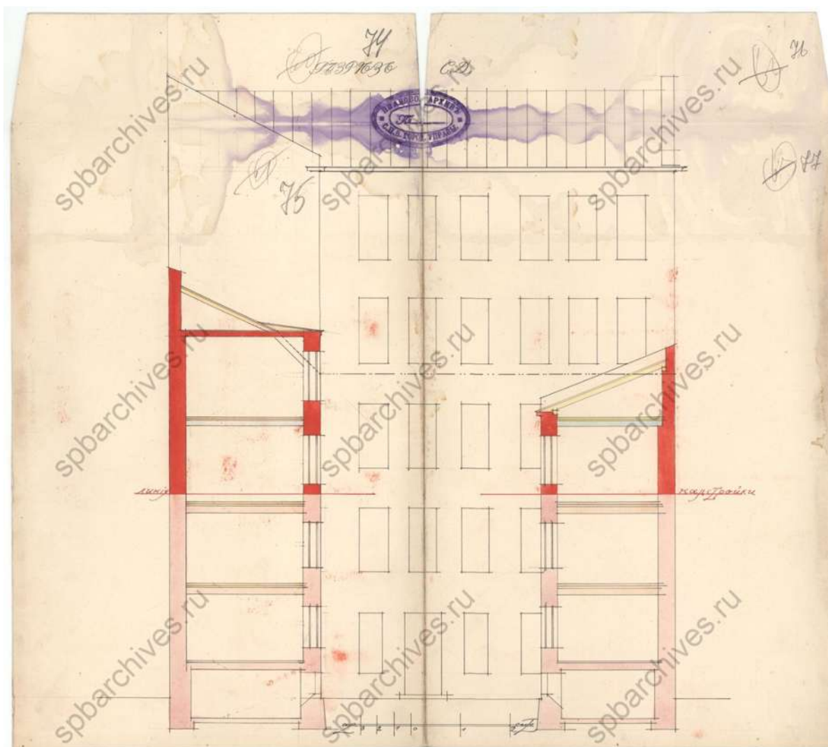
50. Фасад и разрезы. 1913 г. ЦГИА СПб, ф.513, оп.102, д.1670
