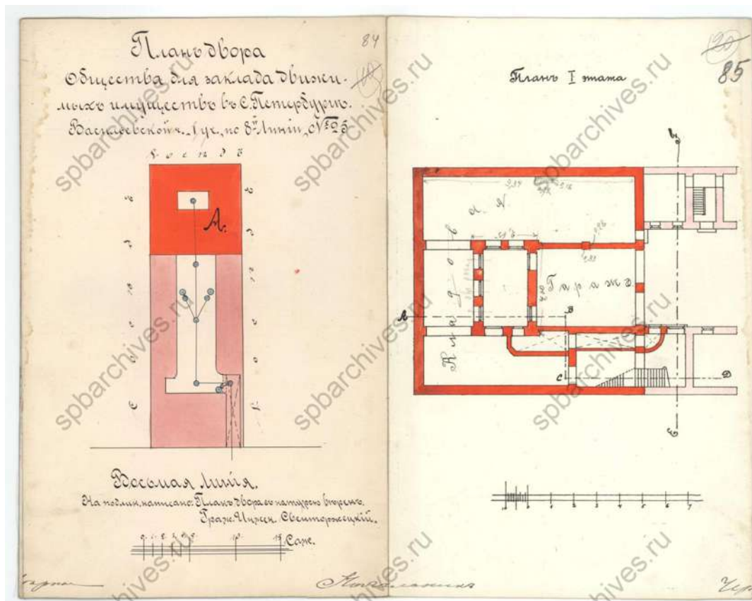
52. План двора Общества Заклада движимого имущества. 1914 г. ЦГИА СПб, ф.513, оп.102, д.1670
