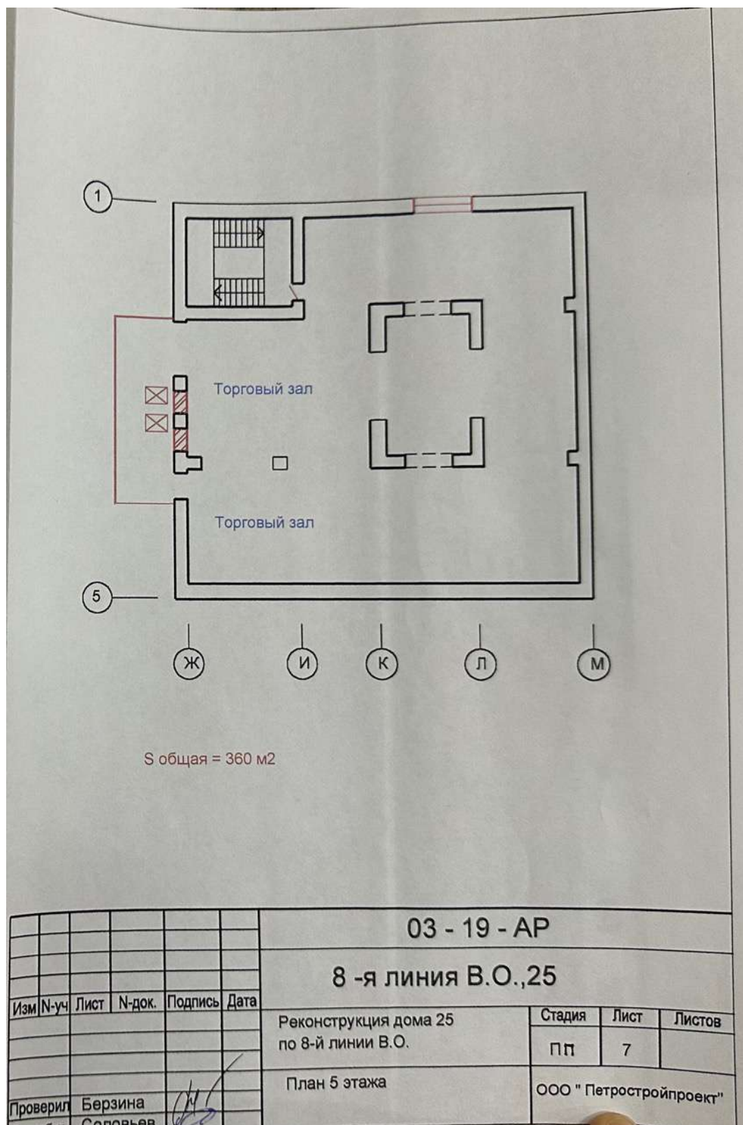
114. План пятого этажа. Объемно-пространственное и архитектурное решение реконструкции дома 25 по 8 линии В.О. СПб, 2003 г. Архив КГИОП П 1500-Л ин. 1025
