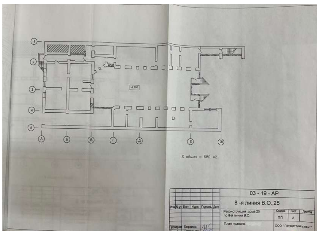
109. План подвала. Объемно-пространственное и архитектурное решение реконструкции дома 25 по 8 линии В.О. СПб, 2003 г. Архив КГИОП П 1500-Л ин. 1025
