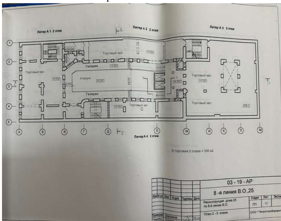
101. План второго-третьего этажей. Объемно-пространственное и архитектурное решение реконструкции дома 25 по 8 линии В.О. СПб, 2003 г. Архив КГИОП П 1500-Л ин. 1024
