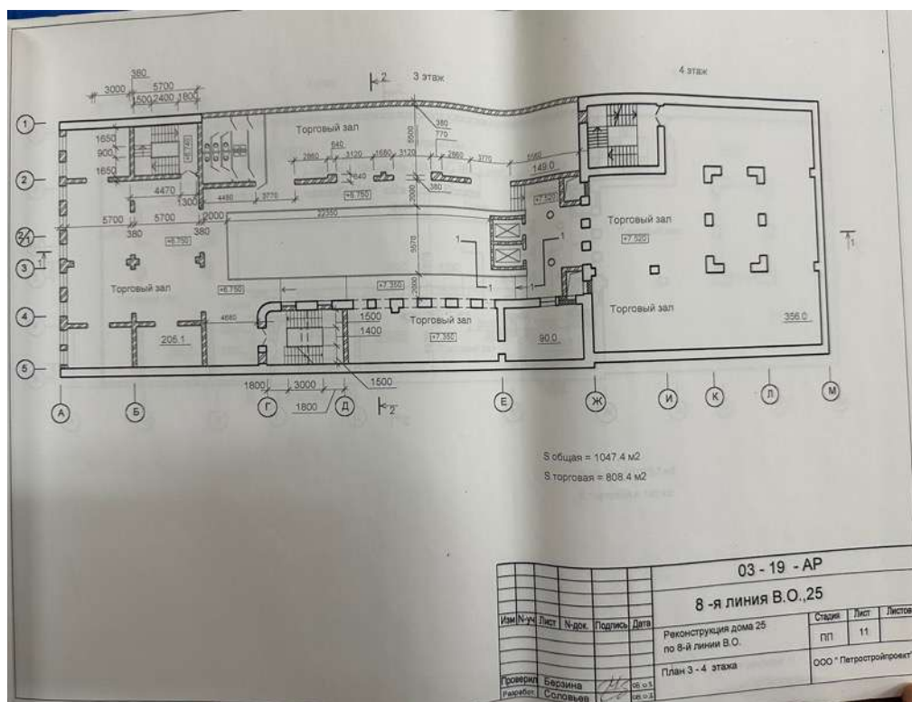
102. План третьего-четвертого этажей. Объемно-пространственное и архитектурное решение реконструкции дома 25 по 8 линии В.О. СПб, 2003 г. Архив КГИОП П 1500-Л ин. 1024
