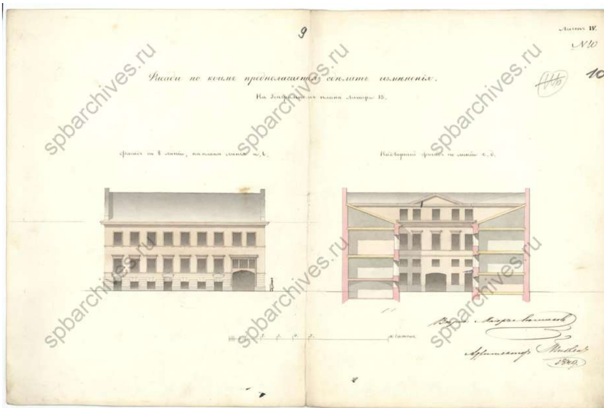
13. Лицевой и дворовой фасады в предполагаемом виде. 1849 г. ЦГИА СПб, ф.513, оп.102, д.1670
