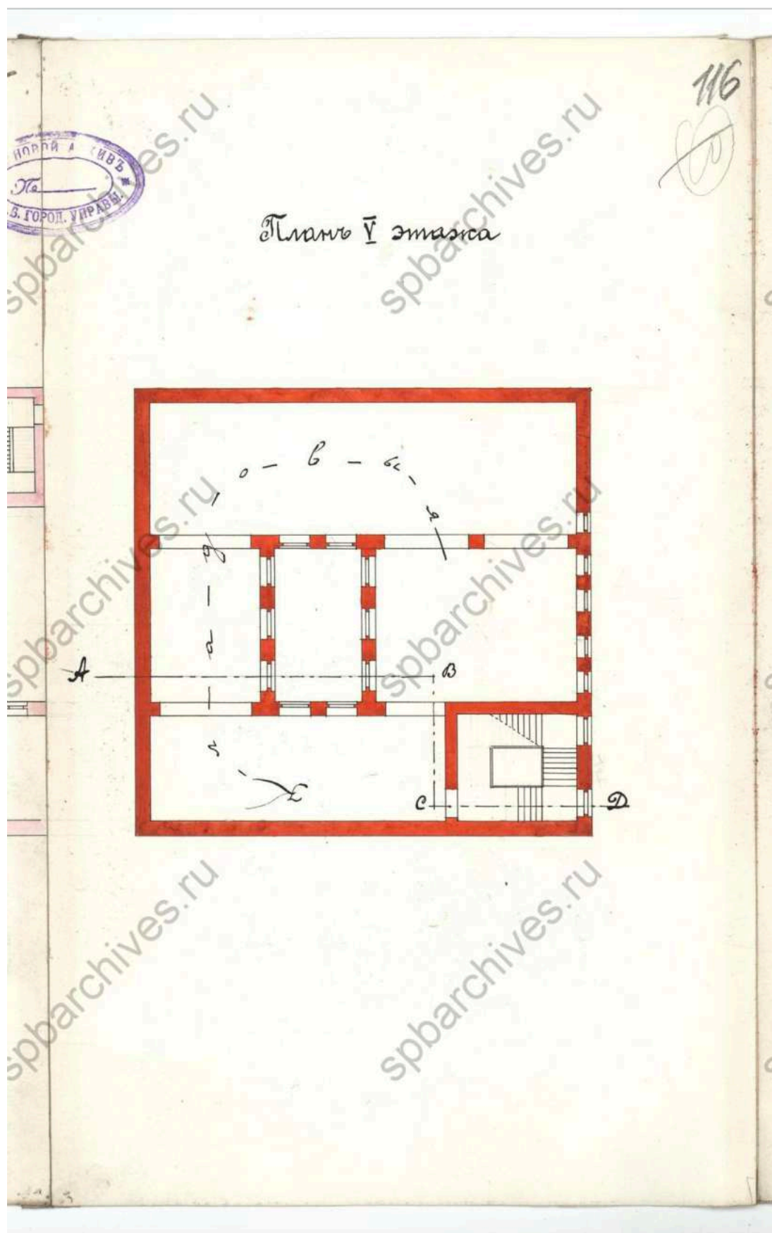
67. План пятого этажа. 1914 г. ЦГИА СПб, ф.513, оп.102, д.1670
