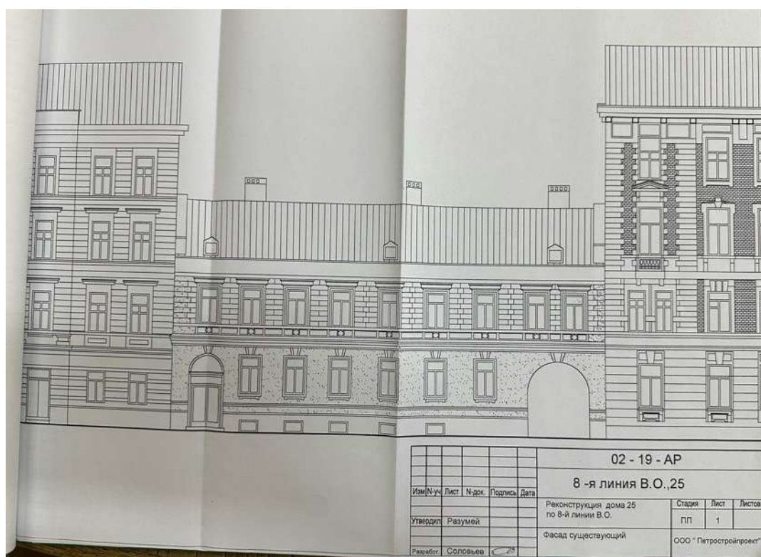
90. Фасад существующий. Объемно-пространственное и архитектурное решение реконструкции дома 25 по 8 линии В.О. СПб, 2002 г. Архив КГИОП П 1500-П ин. 1021
