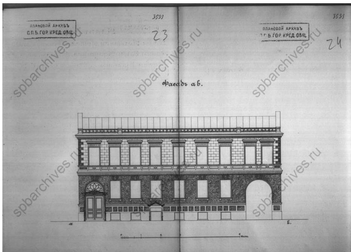
83. Фасад. 1910 г. ЦГИА СПб, ф. 515, оп. 4, д. 2790
