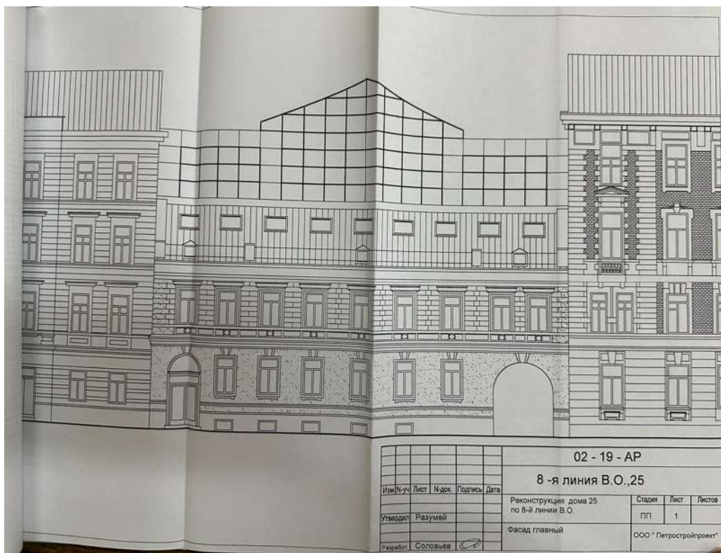
91.Проектируемый фасад. Объемно-пространственное и архитектурное решение реконструкции дома 25 по 8 линии В.О. СПб, 2002 г. Архив КГИОП П 1500-П ин. 1021
