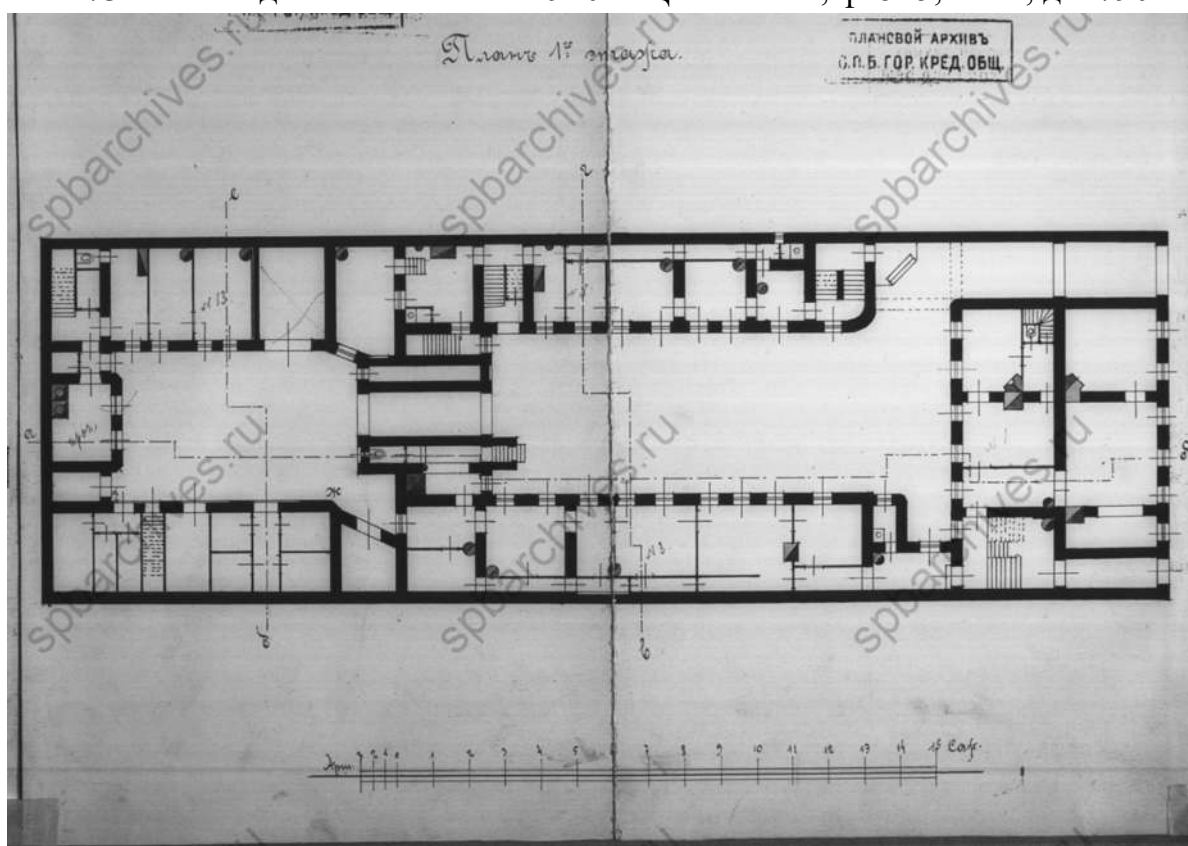
74. План первого этажа. 1910 г. ЦГИА СПб, ф. 515, оп. 4, д. 2790
