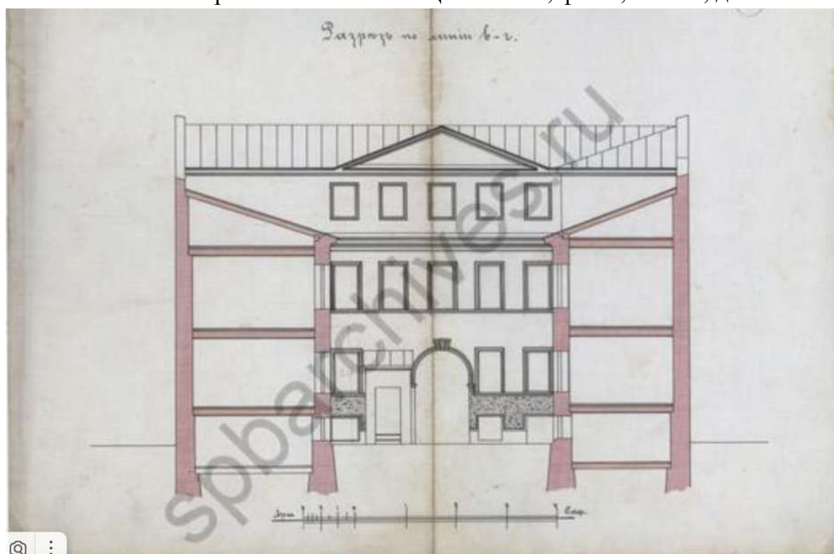
39. Разрез. 1910 г. ЦГИА СПб, ф.513, оп.102, д.1670
