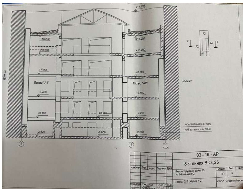
108. Разрез. Объемно-пространственное и архитектурное решение реконструкции дома 25 по 8 линии В.О. СПб, 2003 г. Архив КГИОП П 1500-Л ин. 1024
