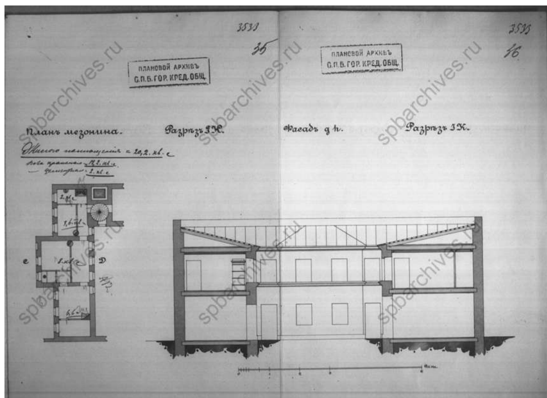
89. План мезонина, разрезы и фасад. 1910 г. ЦГИА СПб, ф. 515, оп. 4, д. 2790
