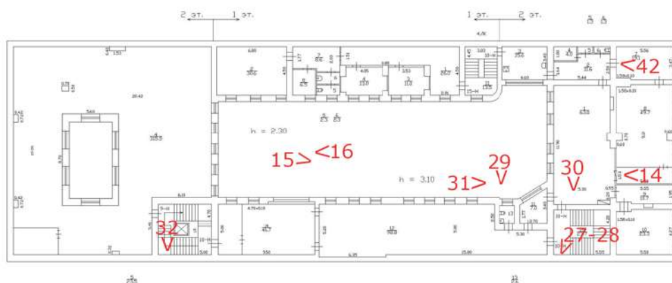
План 1-2 этажа
