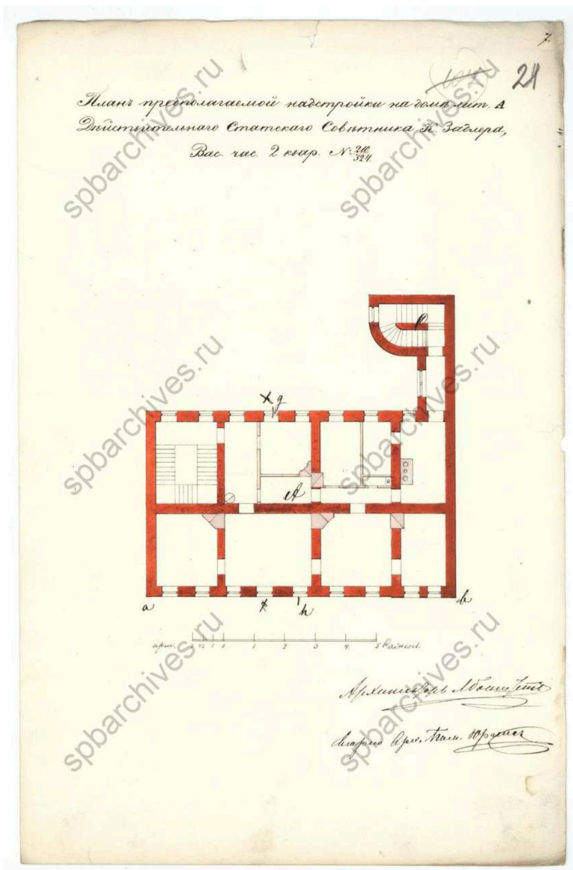
22. План надстройки лицевого корпуса. 1860 г. ЦГИА СПб, ф.513, оп.102, д.1670
