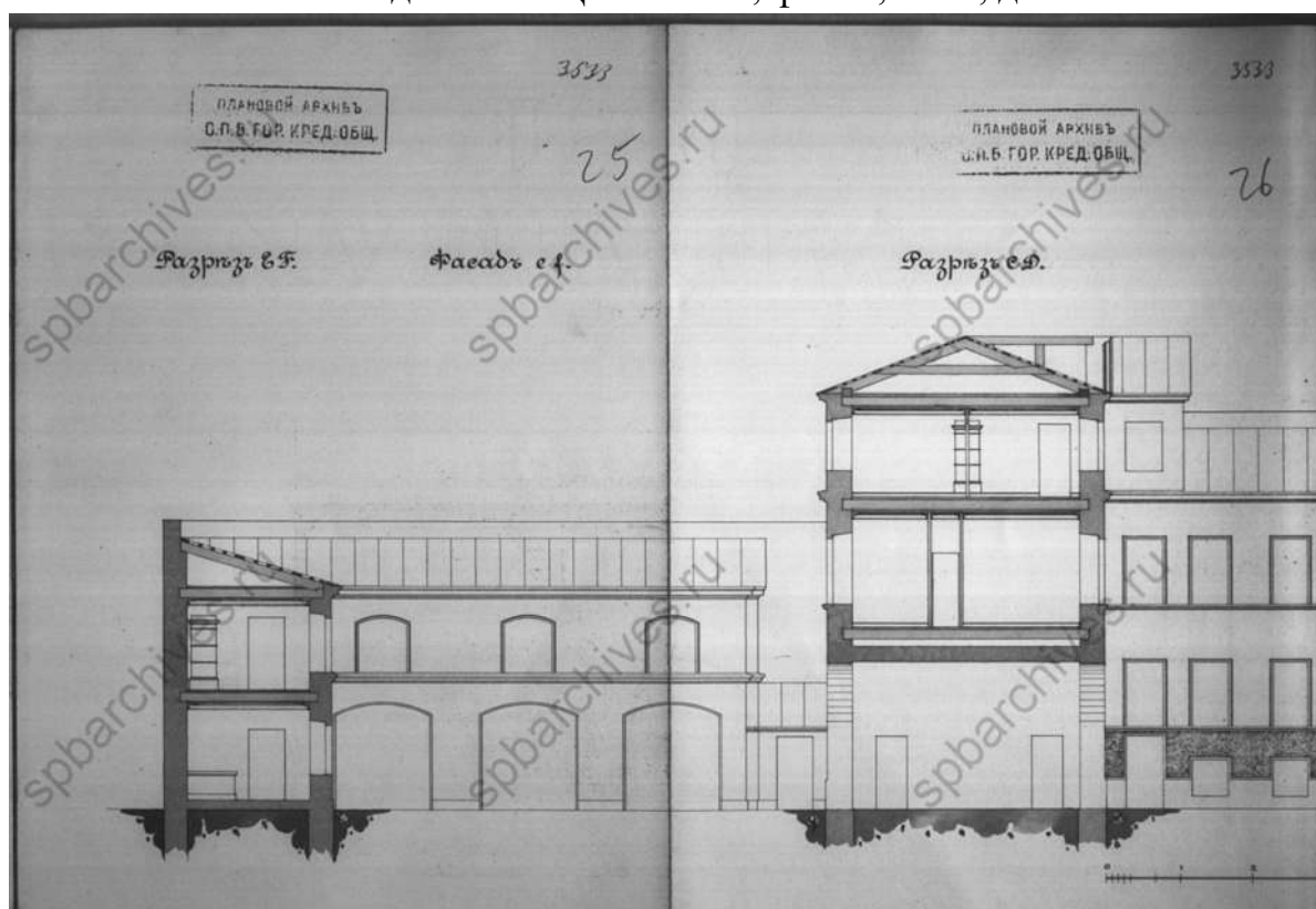
84. Фасады и разрезы. 1910 г. ЦГИА СПб, ф. 515, оп. 4, д. 2790
