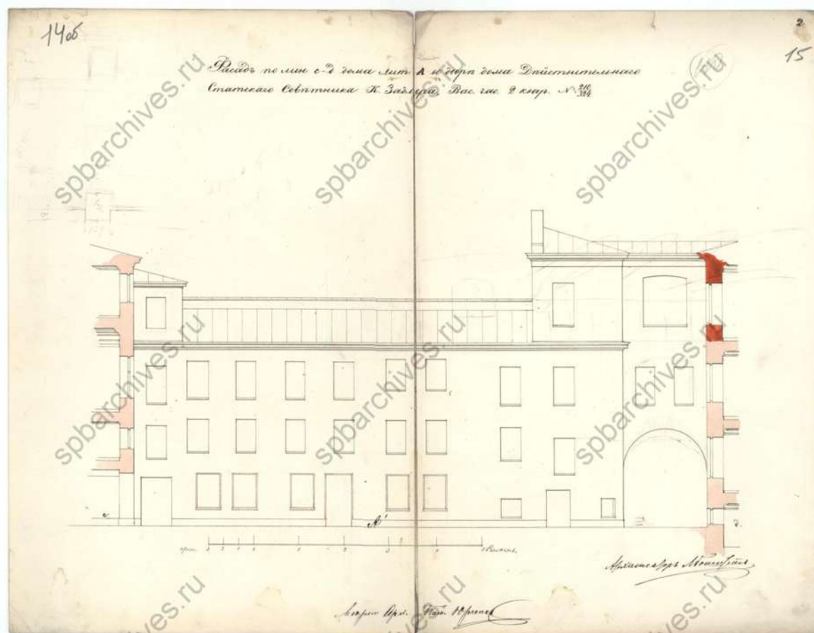
16. Дворовой фасад. 1860 г. ЦГИА СПб, ф.513, оп.102, д.1670
