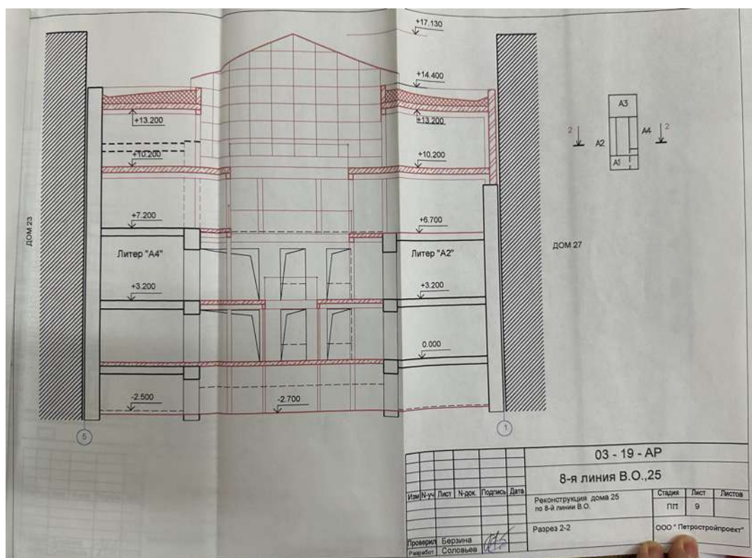
116. Разрез. Объемно-пространственное и архитектурное решение реконструкции дома 25 по 8 линии В.О. СПб, 2003 г. Архив КГИОП П 1500-Л ин. 1025
