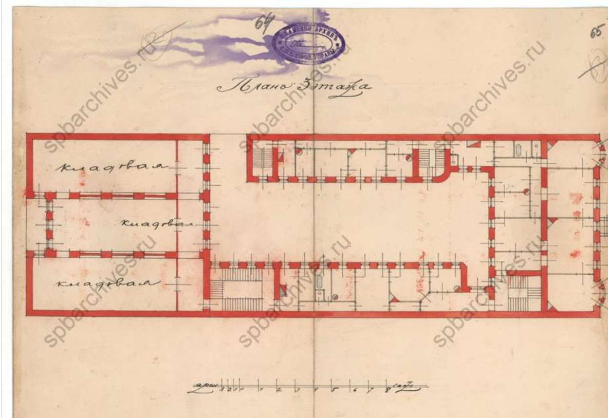
46. План третьего этажа. 1913 г. ЦГИА СПб, ф.513, оп.102, д.1670
