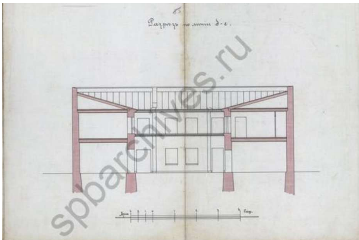
40. Разрез. 1910 г. ЦГИА СПб, ф.513, оп.102, д.1670
