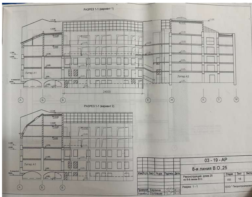
106. Разрез. Объемно-пространственное и архитектурное решение реконструкции дома 25 по 8 линии В.О. СПб, 2003 г. Архив КГИОП П 1500-Л ин. 1024
