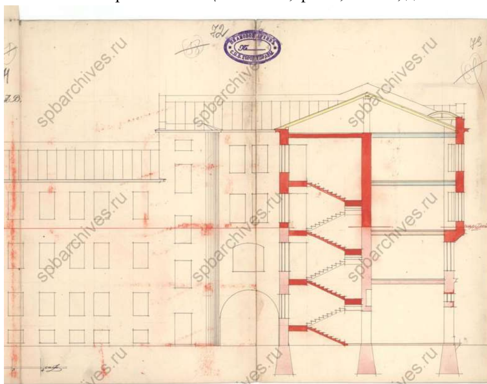
49. Фасад и разрез. 1913 г. ЦГИА СПб, ф.513, оп.102, д.1670
