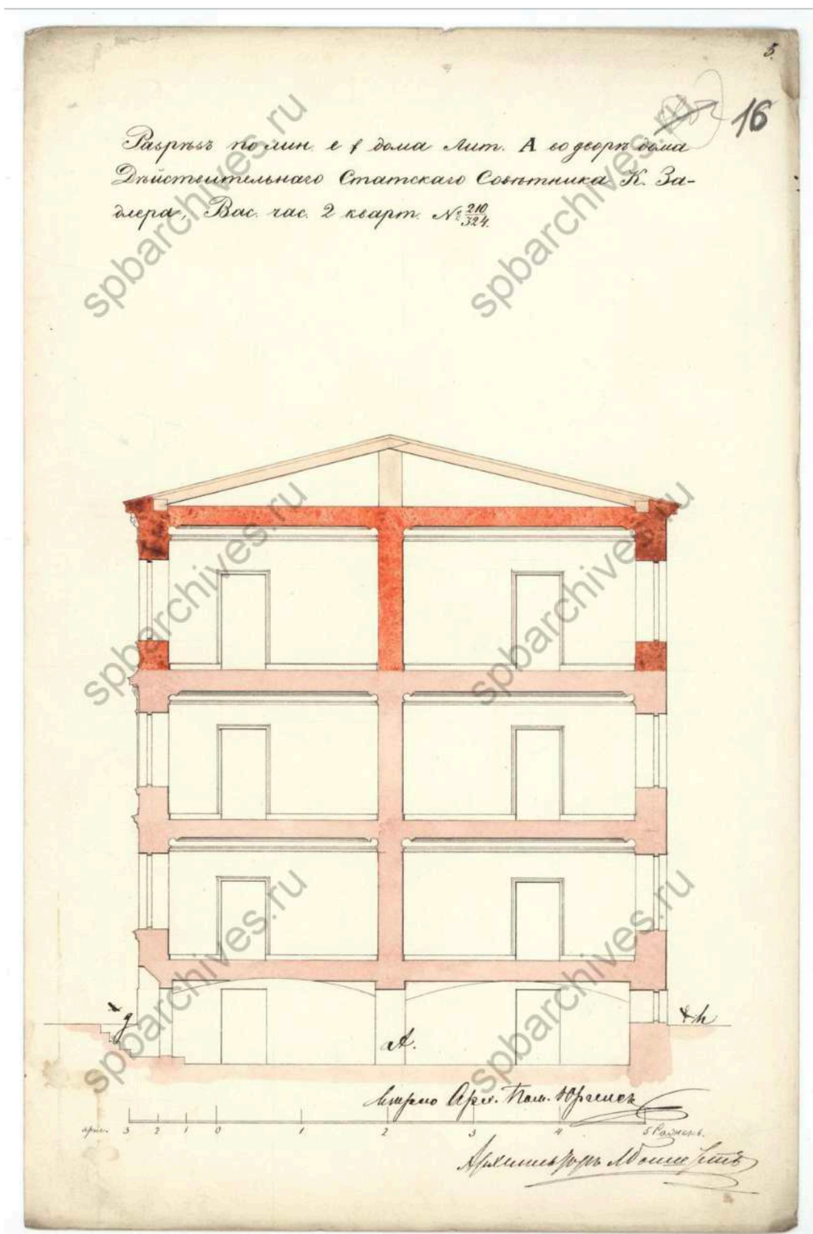
17. Разрез лицевого корпуса. 1860 г. ЦГИА СПб, ф.513, оп.102, д.1670
