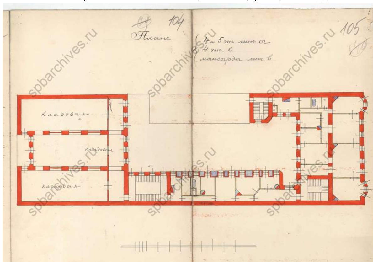
59. План четвертого и пятого этажей и мансарды. 1913 г. ЦГИА СПб, ф.513, оп.102, д.1670
