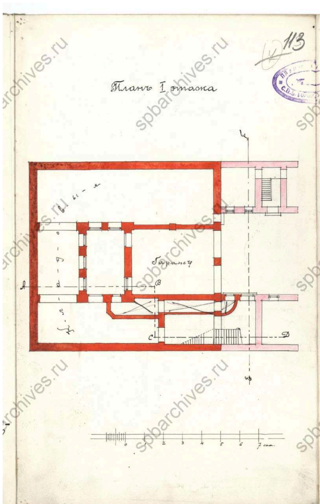
64. План первого этажа. 1914 г. ЦГИА СПб, ф.513, оп.102, д.1670
