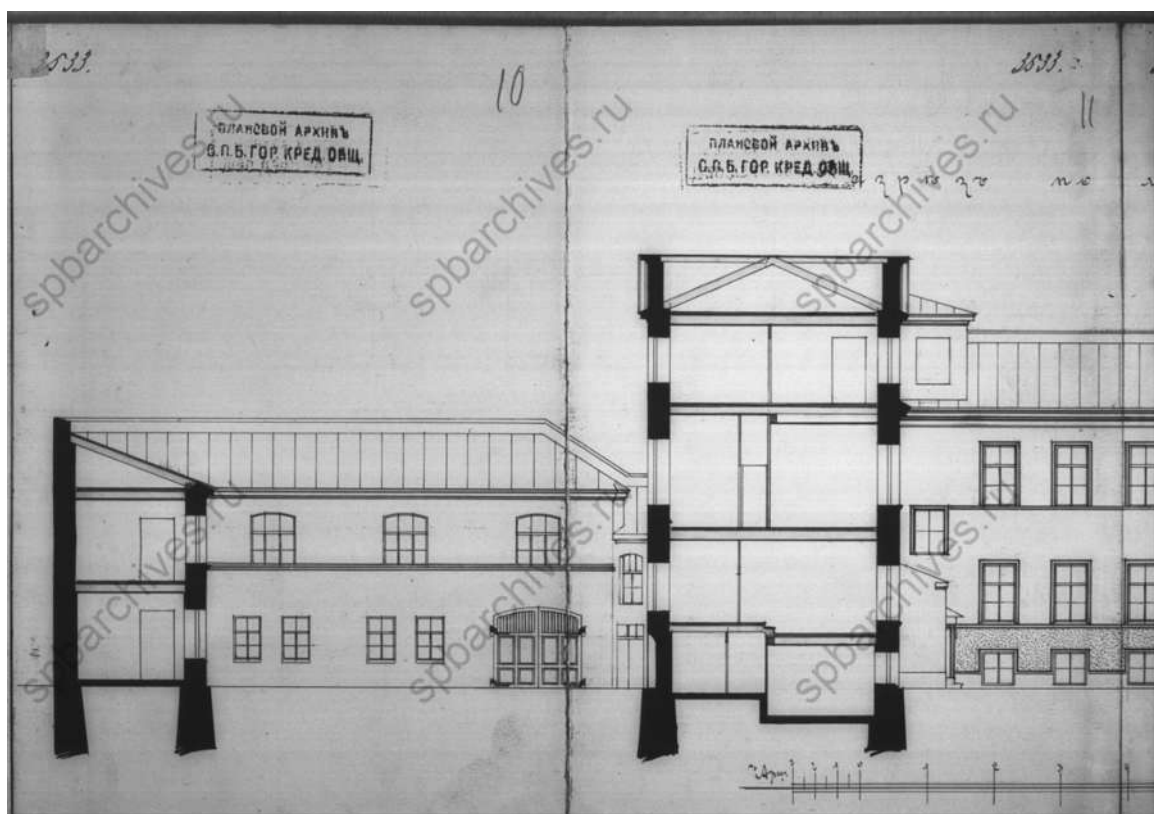
77. Фасады и разрезы. 1910 г. ЦГИА СПб, ф. 515, оп. 4, д. 2790
