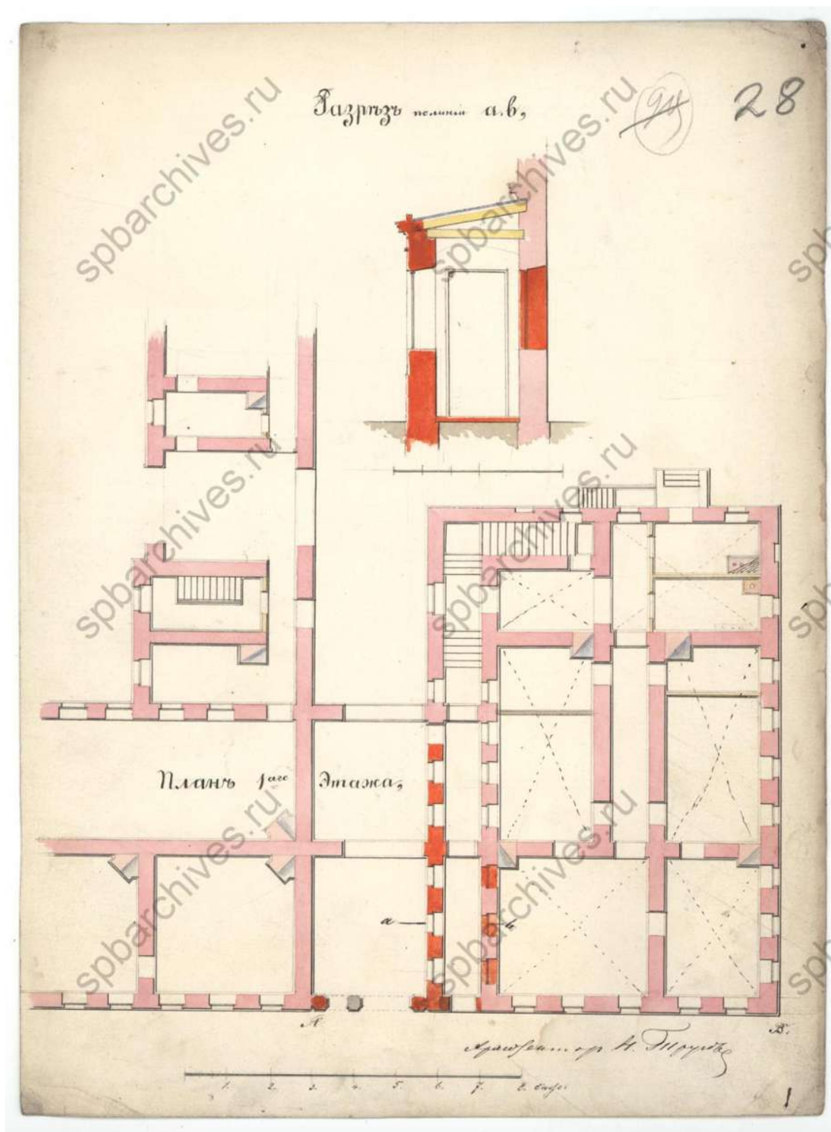
26. Разрез и планы. 1868 г. ЦГИА СПб, ф.513, оп.102, д.1670
