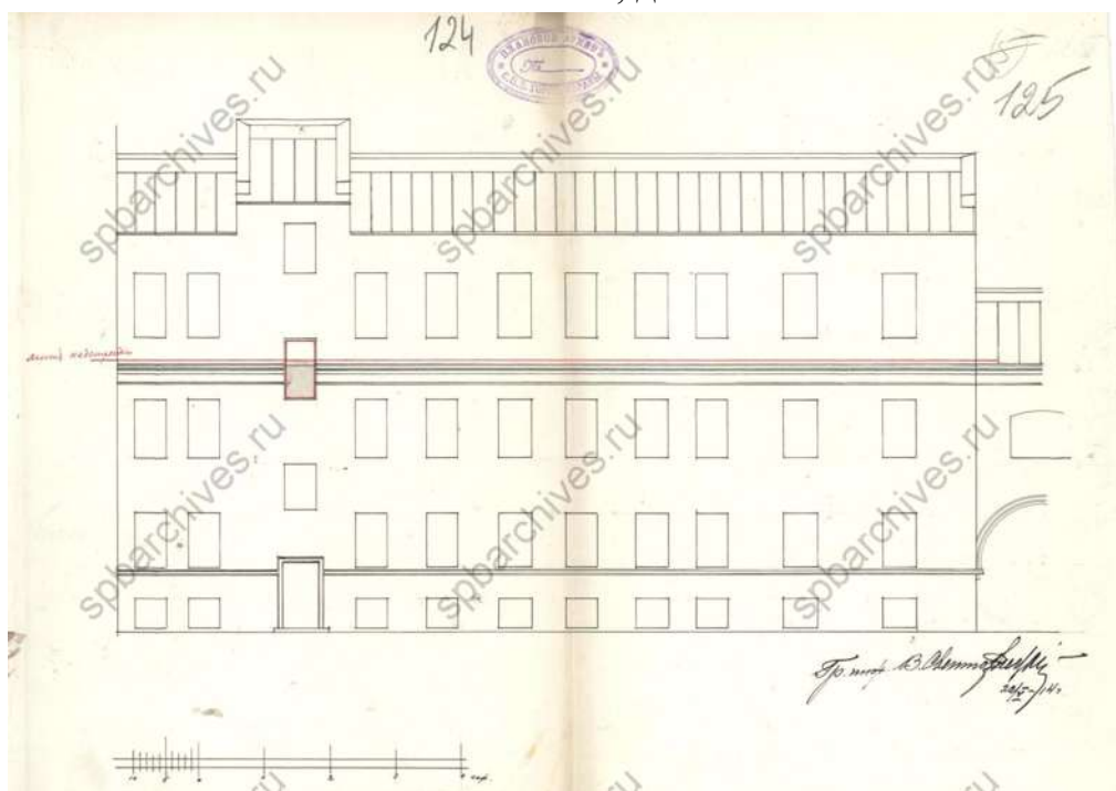
70. Фасад. 1914 г. ЦГИА СПб, ф.513, оп.102, д.1670
