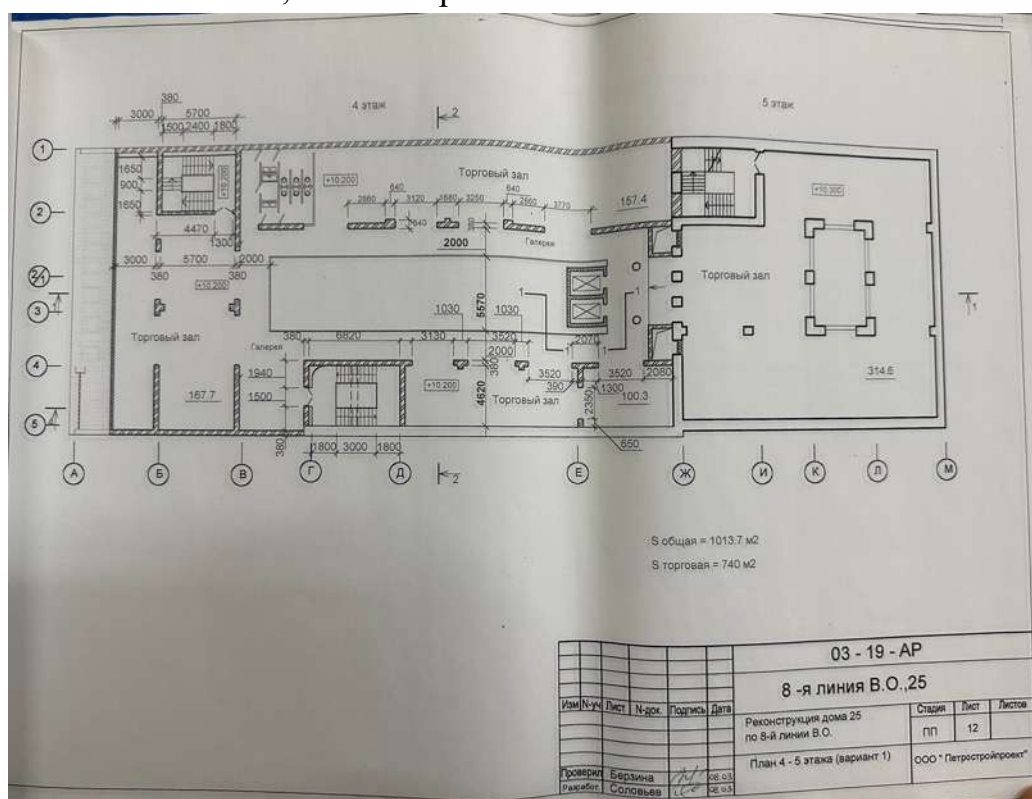
103. План четвертого-пятого этажей (вариант 1). Объемно-пространственное и архитектурное решение реконструкции дома 25 по 8 линии В.О. СПб, 2003 г. Архив КГИОП П 1500-Л ин. 1024
