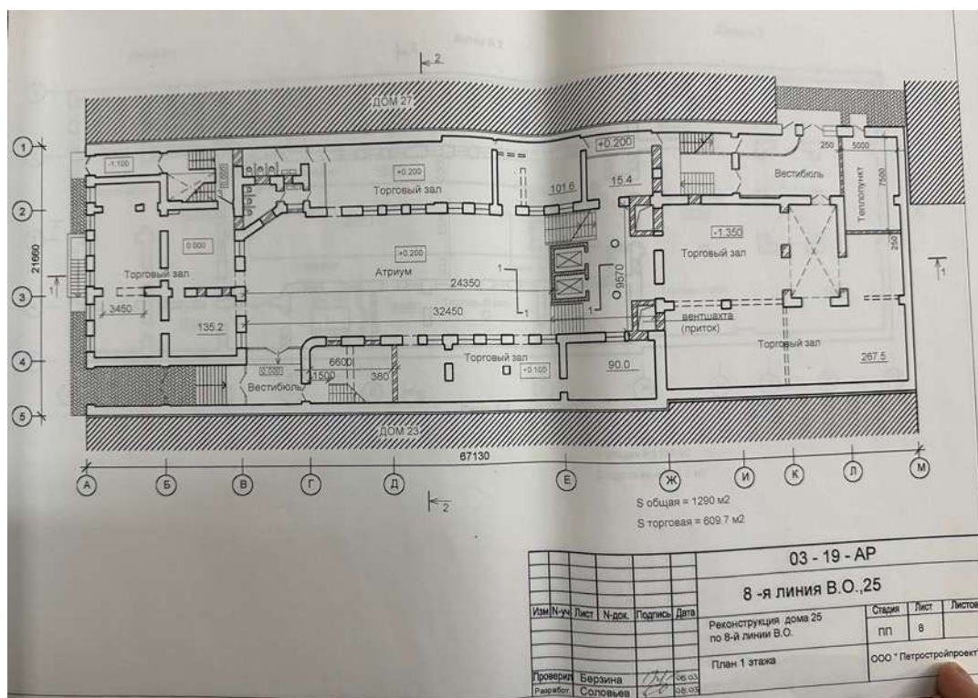
99. План первого этажа. Объемно-пространственное и архитектурное решение реконструкции дома 25 по 8 линии В.О. СПб, 2003 г. Архив КГИОП П 1500-Л ин. 1024
