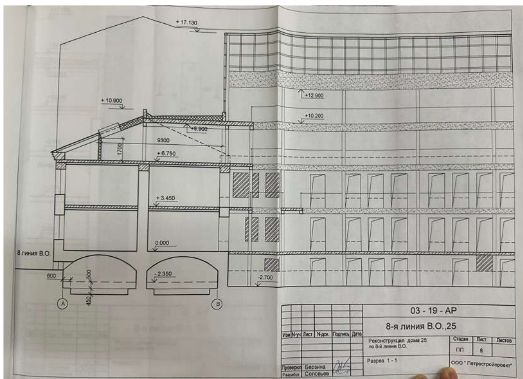
115. Разрез. Объемно-пространственное и архитектурное решение реконструкции дома 25 по 8 линии В.О. СПб, 2003 г. Архив КГИОП П 1500-Л ин. 1025
