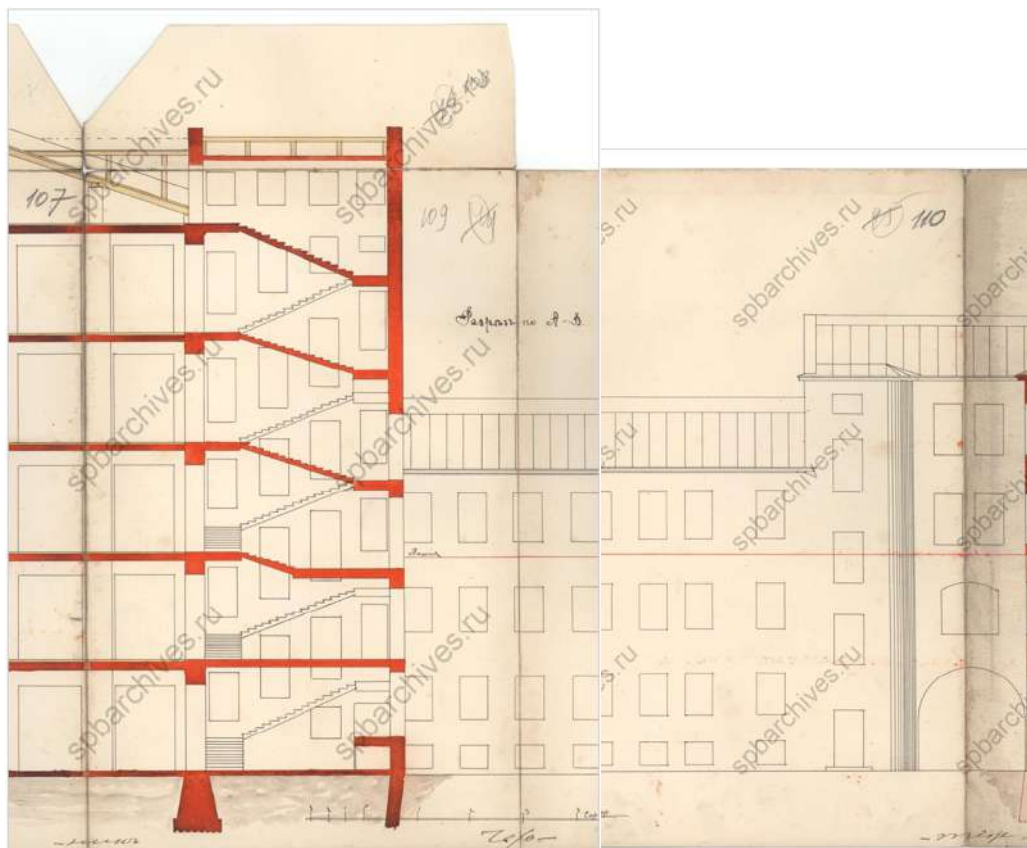
61. Разрез и фасад. 1913 г. ЦГИА СПб, ф.513, оп.102, д.1670
