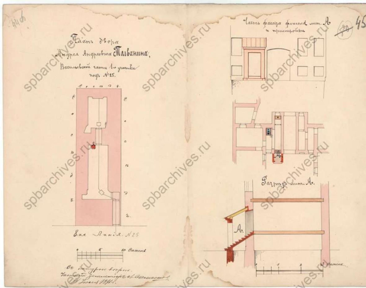
34. План двора Андрея Андреевича Толванина, фрагмент фасада, плана и разреза. 1891 г. ЦГИА СПб, ф.513, оп.102, д.1670
