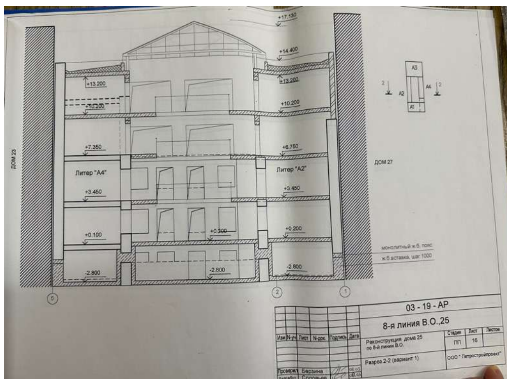
107. Разрез. Объемно-пространственное и архитектурное решение реконструкции дома 25 по 8 линии В.О. СПб, 2003 г. Архив КГИОП П 1500-Л ин. 1024
