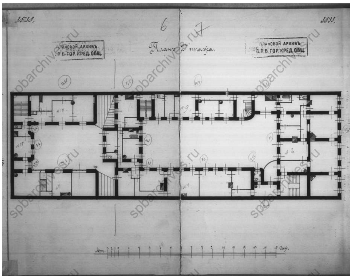
75. План второго этажа. 1910 г. ЦГИА СПб, ф. 515, оп. 4, д. 2790
