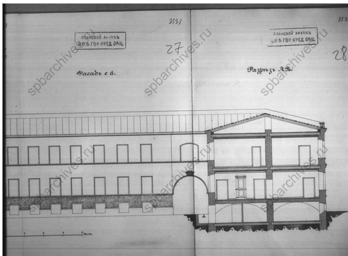
85. Фасад и разрез. 1910 г. ЦГИА СПб, ф. 515, оп. 4, д. 2790
