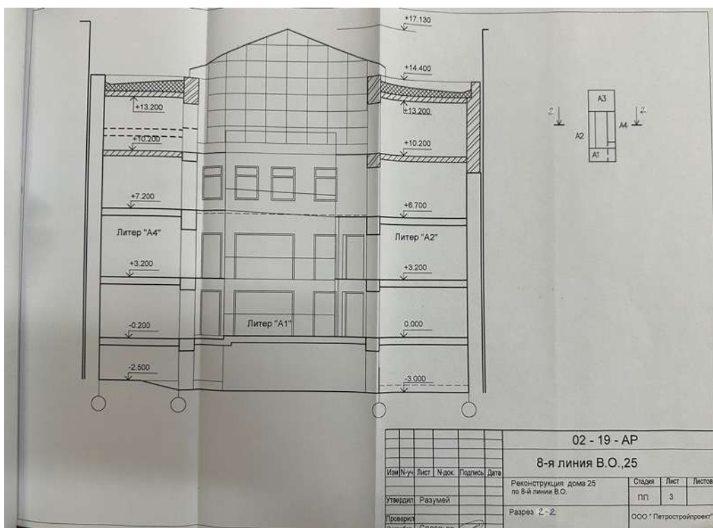
93. Разрез. Объемно-пространственное и архитектурное решение реконструкции дома 25 по 8 линии В.О. СПб, 2002 г. Архив КГИОП П 1500-П ин. 1021
