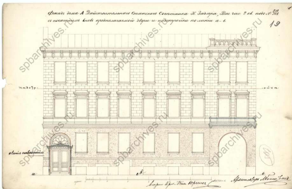
20. Лицевой фасад в предполагаемом виде. 1860 г. ЦГИА СПб, ф.513, оп.102, д.1670
