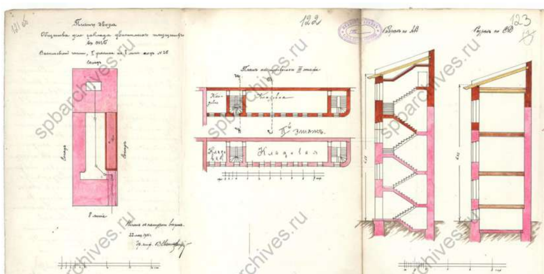
69. План двора, планы этажей и разрезы. 1914 г. ЦГИА СПб, ф.513, оп.102, д.1670
