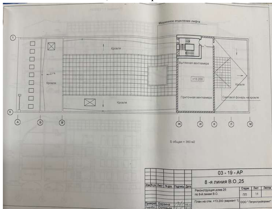
105. План на отметке 13200. Объемно-пространственное и архитектурное решение реконструкции дома 25 по 8 линии В.О. СПб, 2003 г. Архив КГИОП П 1500-Л ин. 1024
