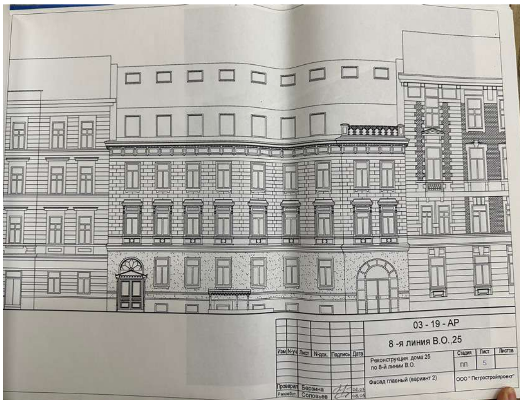
96. Проектируемый фасад. Объемно-пространственное и архитектурное решение реконструкции дома 25 по 8 линии В.О. СПб, 2003 г. Архив КГИОП П 1500-Л ин. 1024
