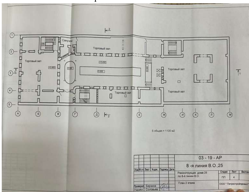
111. План второго этажа. Объемно-пространственное и архитектурное решение реконструкции дома 25 по 8 линии В.О. СПб, 2003 г. Архив КГИОП П 1500-Л ин. 1025
