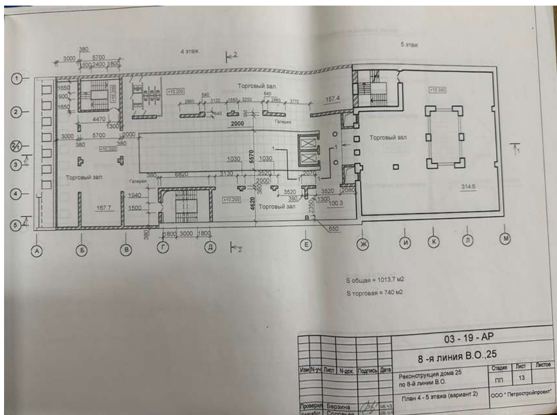
104. План четвертого-пятого этажей (вариант 2). Объемно-пространственное и архитектурное решение реконструкции дома 25 по 8 линии В.О. СПб, 2003 г. Архив КГИОП П 1500-Л ин. 1024
