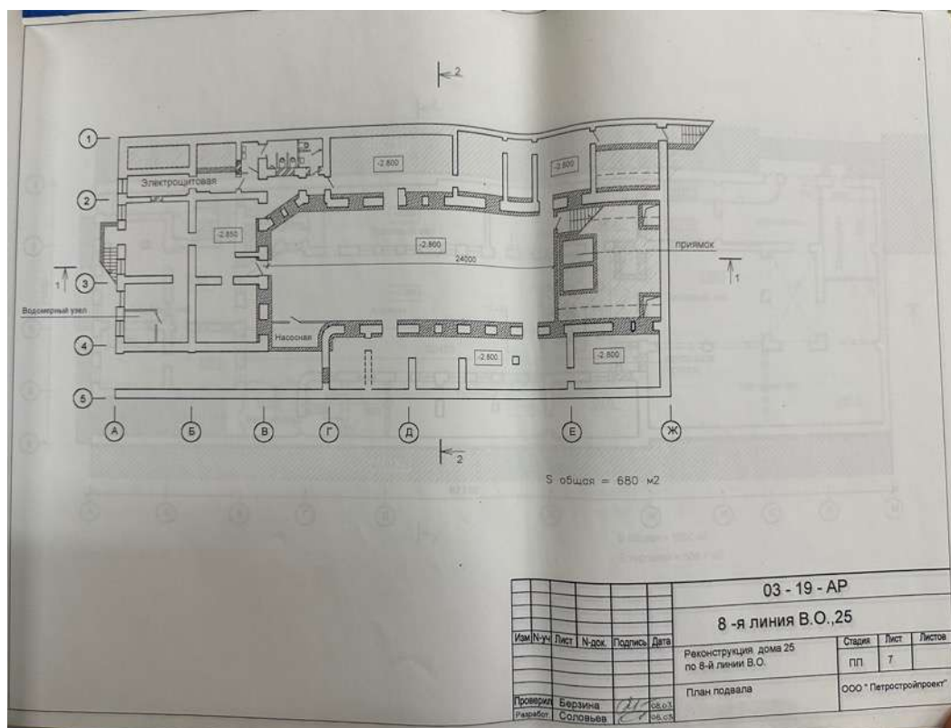
98. План подвала. Объемно-пространственное и архитектурное решение реконструкции дома 25 по 8 линии В.О. СПб, 2003 г. Архив КГИОП П 1500-Л ин. 1024
