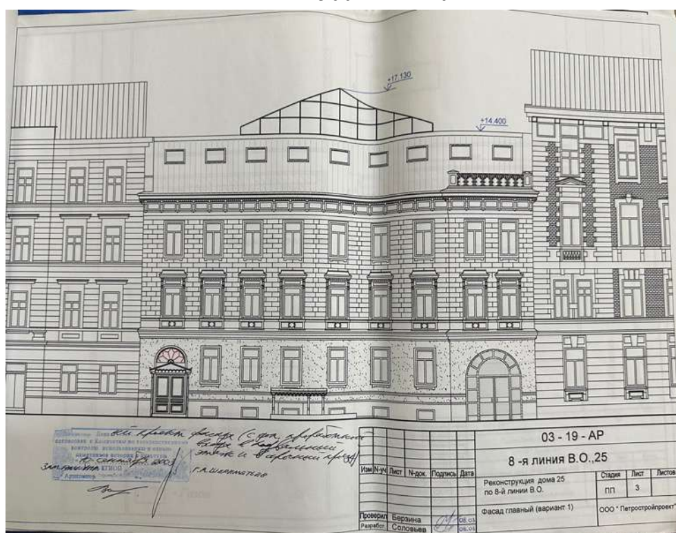
94. Проектируемый фасад. Объемно-пространственное и архитектурное решение реконструкции дома 25 по 8 линии В.О. СПб, 2003 г. Архив КГИОП П 1500-Л ин. 1024
