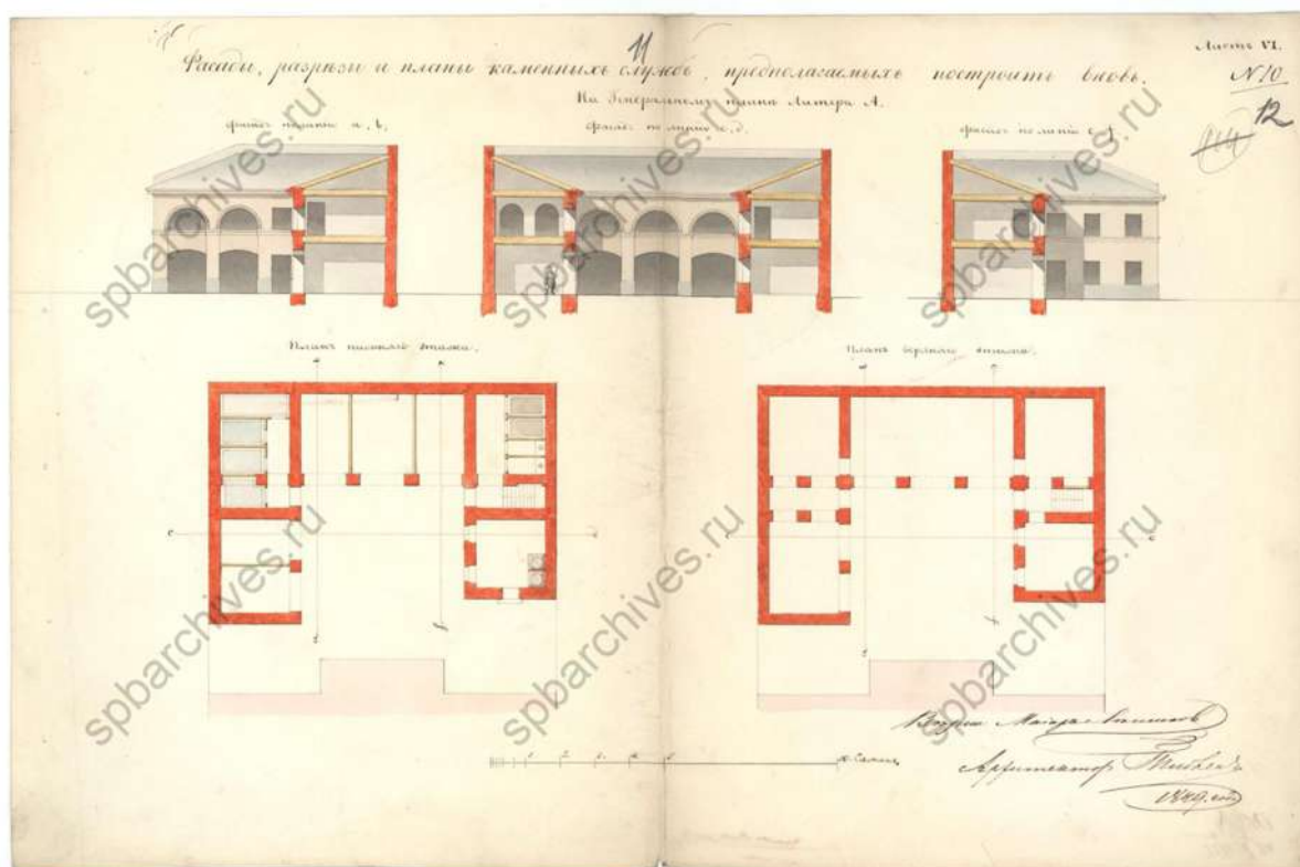
14. Фасады и разрезы предполагаемых к постройке служб. 1849 г. ЦГИА СПб, ф.513, оп.102, д.1670
