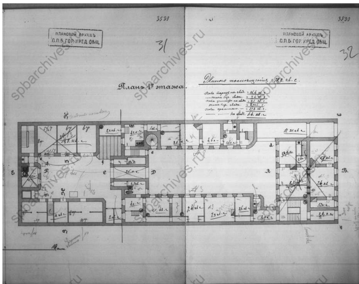
87. План первого этажа. 1910 г. ЦГИА СПб, ф. 515, оп. 4, д. 2790
