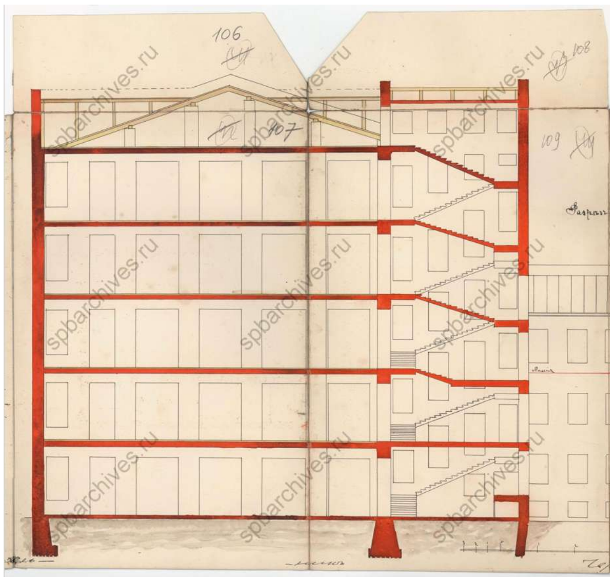
60. Разрез. 1913 г. ЦГИА СПб, ф.513, оп.102, д.1670
