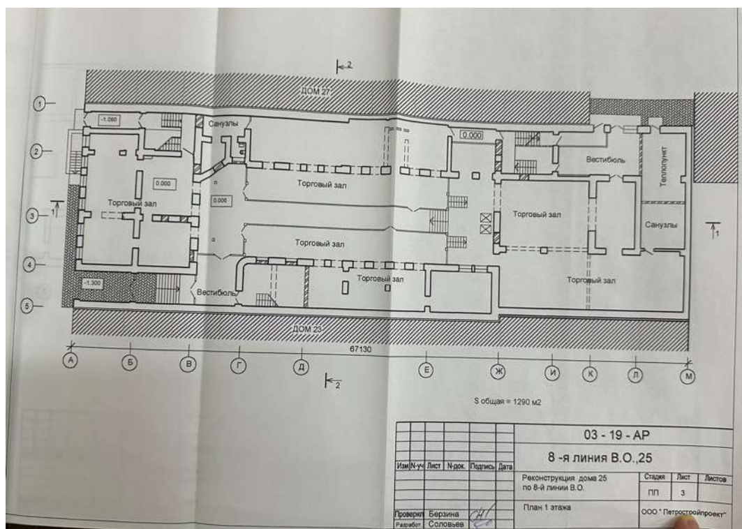
110. План первого этажа. Объемно-пространственное и архитектурное решение реконструкции дома 25 по 8 линии В.О. СПб, 2003 г. Архив КГИОП П 1500-Л ин. 1025
