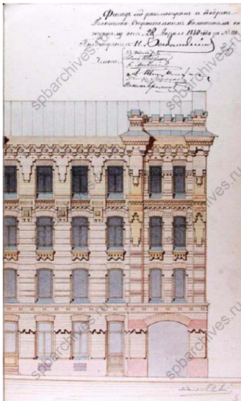
Илл. 23. Фрагмент фасада. Московскому пр. ЦГИА СПб. Ф. 513. О. 102. Д. 5335. 1878-1880 г.
