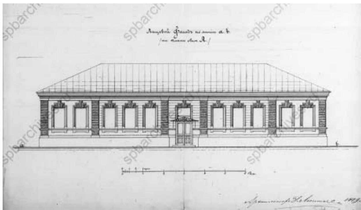
16. 1879. Лицевой (южный) фасад предполагаемой больницы С.Петербургской Духовной Семинарии. Арх. Д.В. Люшин. 1879 г. ЦГИА СПб. Ф. 513. Оп. 102. Д. 760
