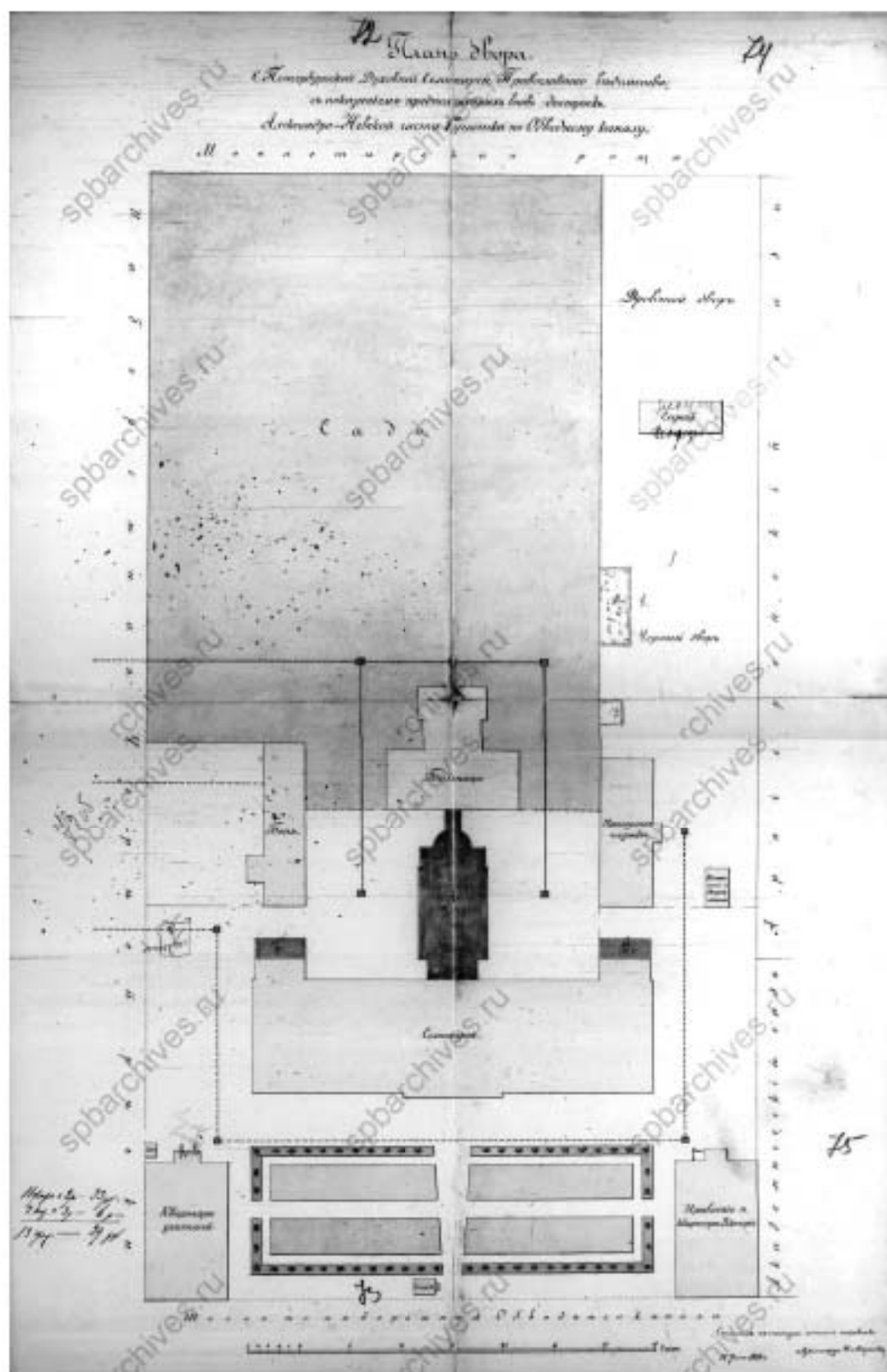
1886. План двора С.Петербургской Духовной Семинарии с показанием предполагаемых вновь достроек. Арх. Н.Л. Марков. ЦГИА СПб. Ф. 513. Оп. 102. Д. 760
