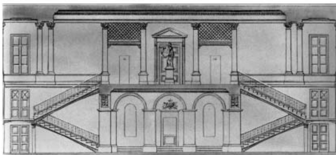
28. «Театр Михайловский» (пл. Искусств, д. 1, лит. А). Разрез по главной лестнице. Проект А.П.Брюллова (22).
