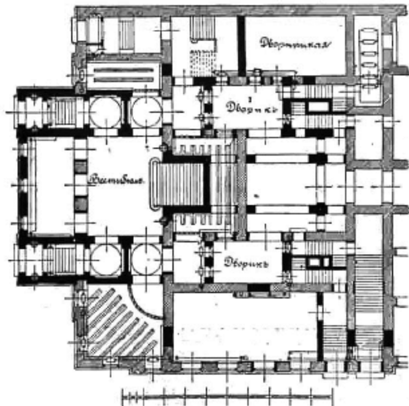
195. План 1-го этажа.
