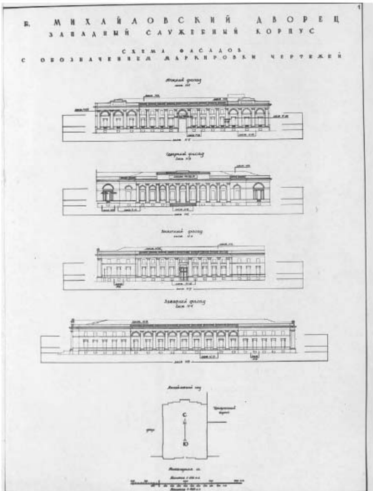
14. «Корпус западный Русского музея (в составе «Дворец Великого князя Михаила Павловича (Русский музей Императора Александра III)») (Инженерная ул., д. 2-4, лит. А). Обмеры 1956 г., Т.В.Берсенева, Д.А.Кючарианц (Паспорт ОКН, инв. 167-4 193П).
