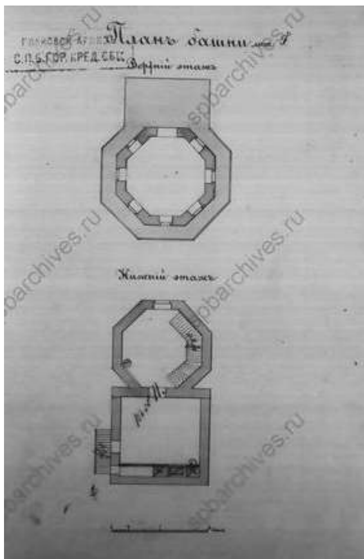
20. План 5 этажа и башенного объема дома по Николаевской улице № 72 (76) (ЦГИА СПб, ф. 515, оп. 4, д. 3311)
