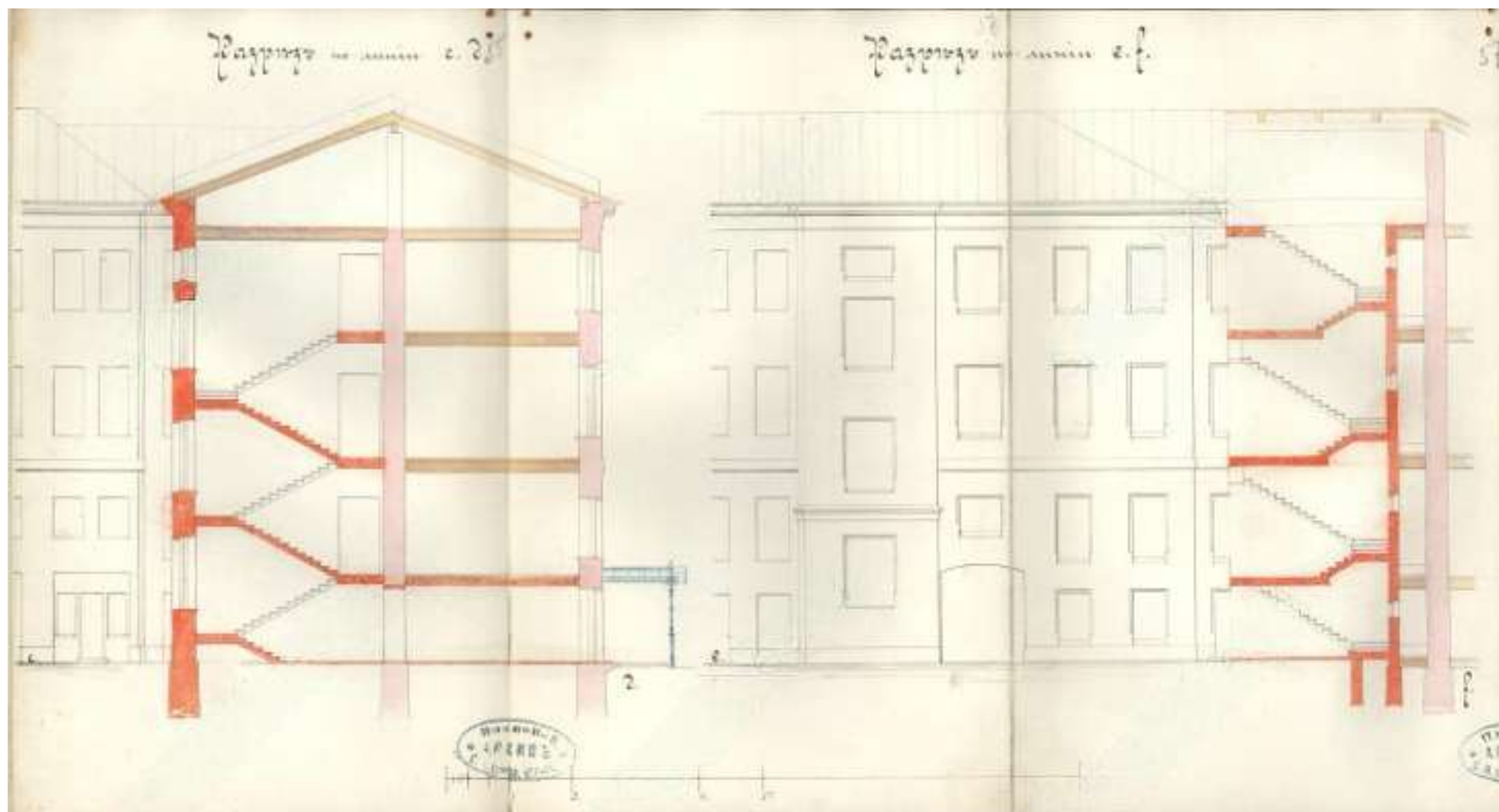
34. Разрез по линии cd. Разрез по линии ef. 1881 г. // Источник: ЦГИА СПб фонд 513, опись 102, дело 213, листы 55-57. Чертежи дома на участке, принадлежавшем В.И.Струбинскому, А.И.Трейбергу по Невскому пр., 11.
