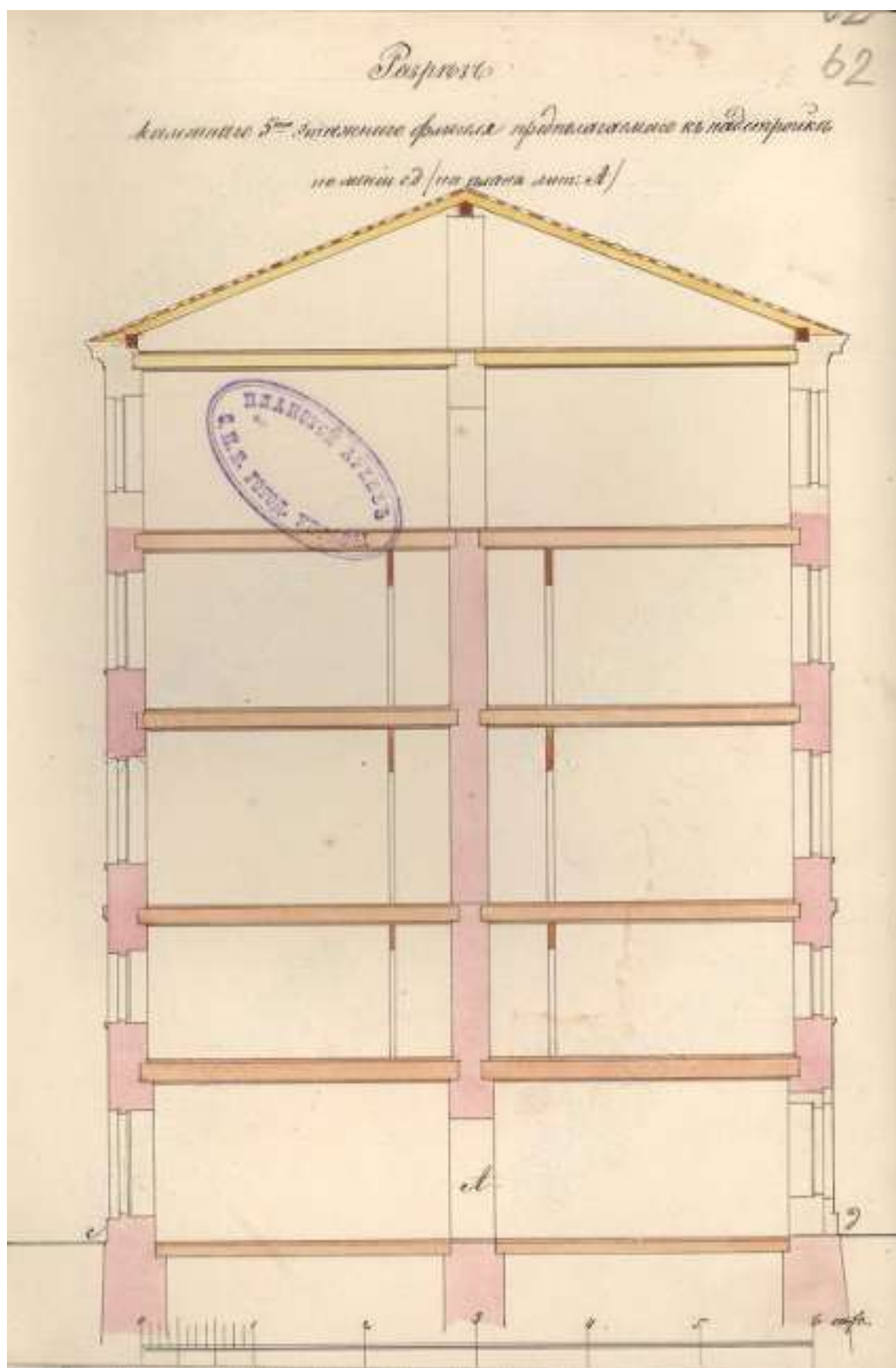
39. Разрез каменного 5-тиэтажного флигеля предполагаемого к постройке по линии сд / на плане лит. А / 1891 г. // Источник: ЦГИА СПб фонд 513, опись 102, дело 213, лист 62. Чертежи дома на участке, принадлежавшем В.И.Струбинскому, А.И.Трейбергу по Невскому пр., 11.
