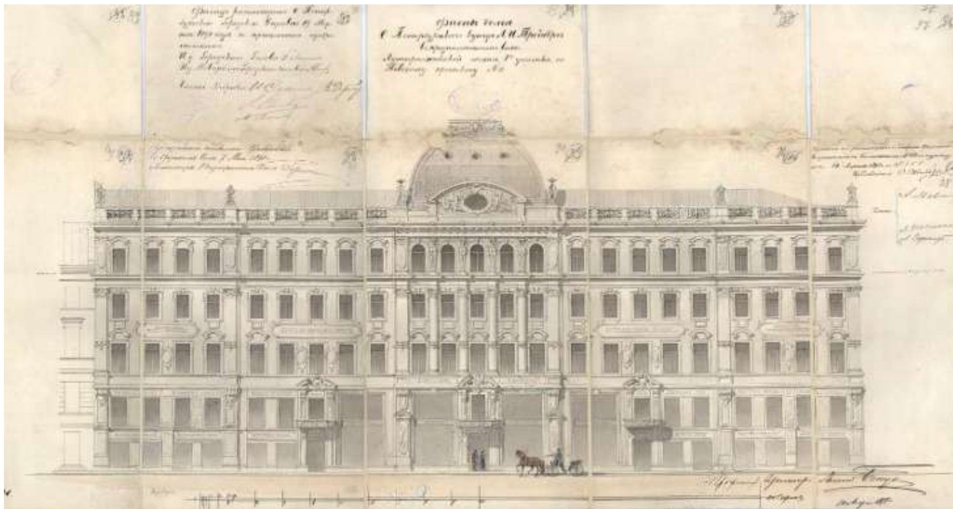
48. Фасад дома СПбербургского купца А.И. Трейберга в предполагаемом виде Адмиралтейской части 1-го участка по Невскому проспекту №11. Подпись архитектора Л.Бенуа. 1898 г. // Источник: ЦГИА СПб фонд 513, опись 102, дело 213, листы 89-98. Чертежи дома на участке, принадлежавшем В.И.Струбинскому, А.И.Трейбергу по Невскому пр., 11.
