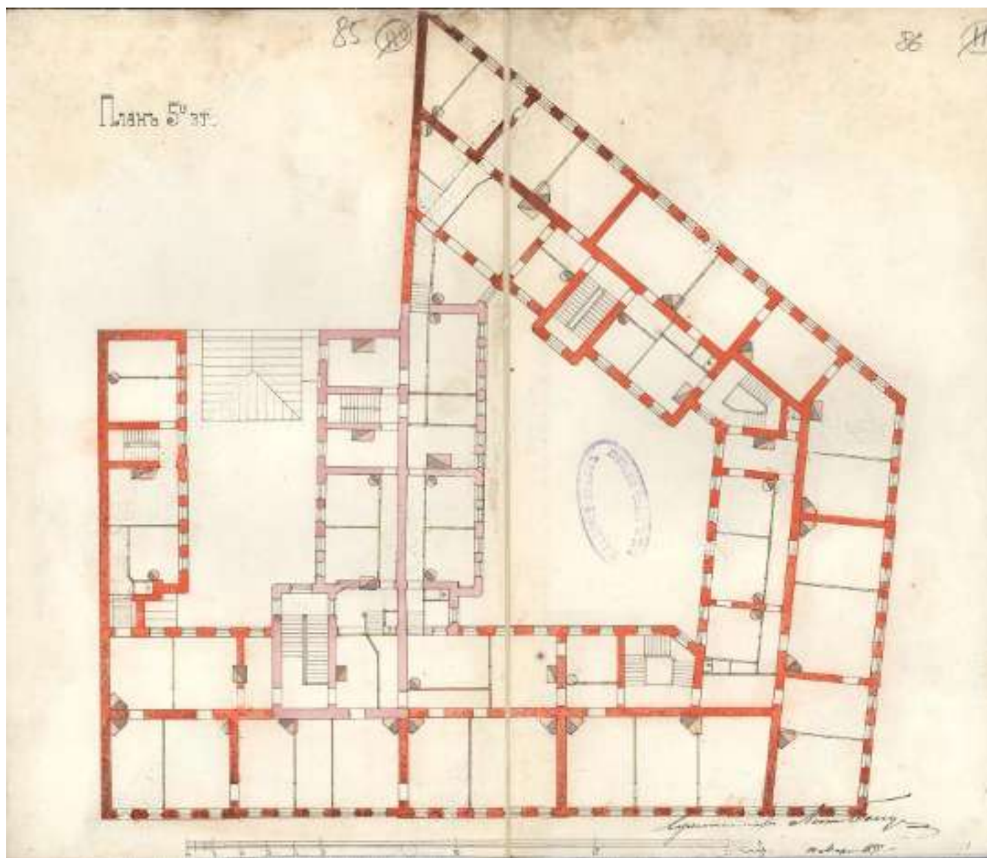
47. План 5 этажа. Подпись архитектора Л.Бенуа. 1898 г. // Источник: ЦГИА СПб фонд 513, описание 102, дело 213, листы 85-86. Чертежи дома на участке, принадлежавшем В.И.Струбинскому, А.И.Трейбергу по Невскому пр., 11.
