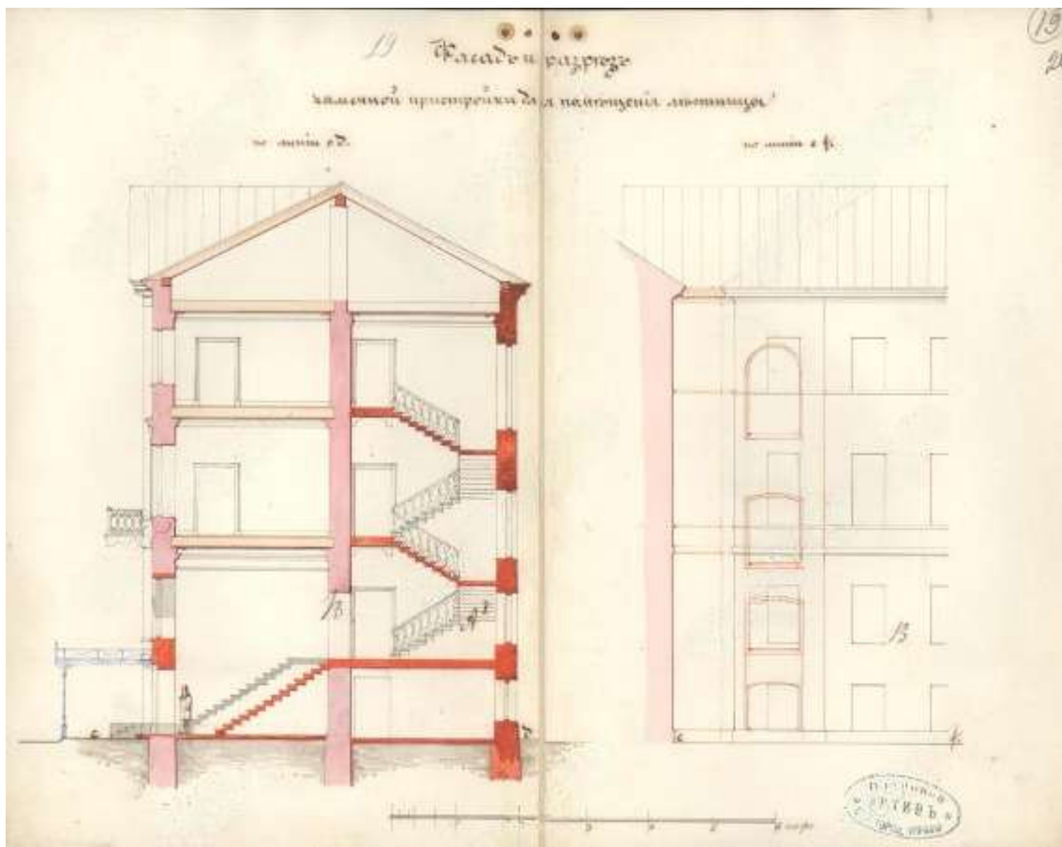
21. Фасад и разрез каменной пристройки для помещения лестницы. 1870 г. // Источник: ЦГИА СПб фонд 513, опись 102, дело 213, листы 19-20. Чертежи дома на участке, принадлежавшем В.И.Струбинскому, А.И.Трейбергу по Невскому пр., 11.
