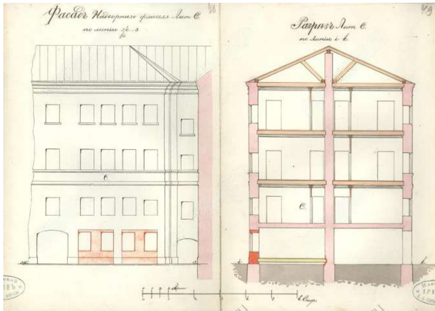
31. Фасад надворного флигеля лит.С по линии ж-з. Разрез лит.С по линии і-к. 1873 г. // Источник: ЦГИА СПб фонд 513, опись 102, дело 213, листы 48-49. Чертежи дома на участке, принадлежавшем В.И.Струбинскому, А.И.Трейбергу по Невскому пр., 11.
