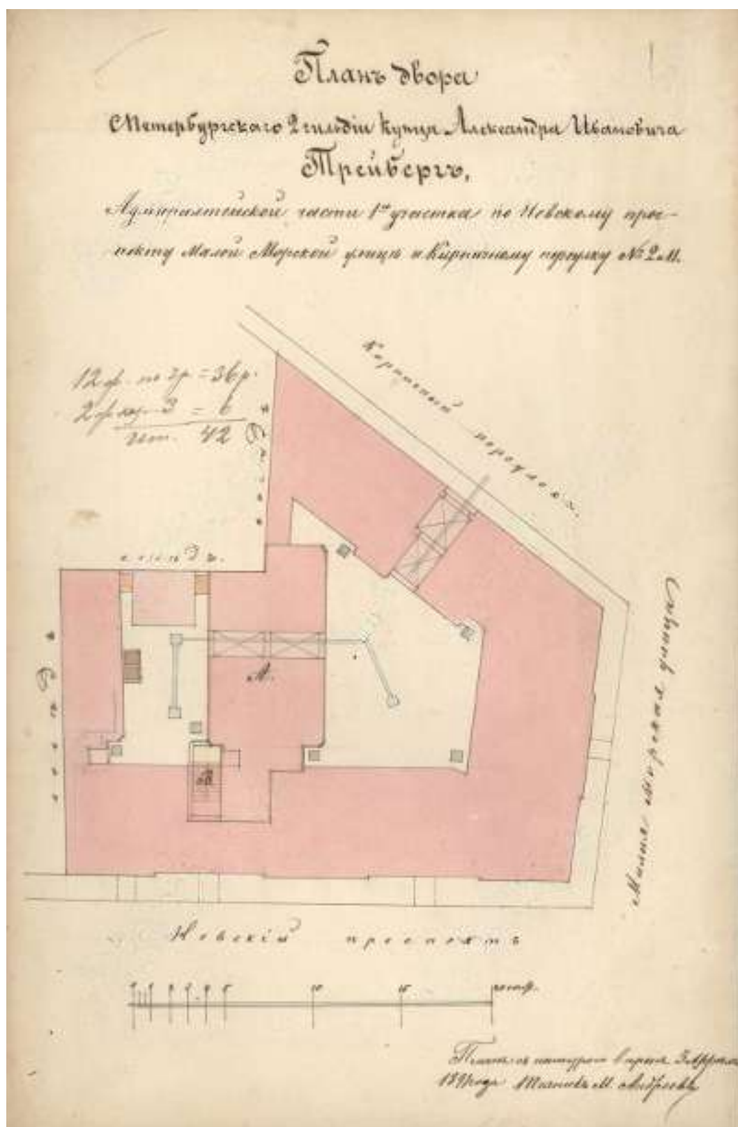
38. План двора С.Петербургского 2 гильдии купца Александра Ивановича Трейберга Адмиралтейской части 1-го участка по Невскому проспекту, Малой Морской улице и Кирпичному переулку №2/11. Подпись техника М.Андреева. 1891 г. // Источник: ЦГИА СПб фонд 513, опись 102, дело 213, лист 61об. Чертежи дома на участке, принадлежавшем В.И.Струбинскому, А.И.Трейбергу по Невскому пр., 11.
