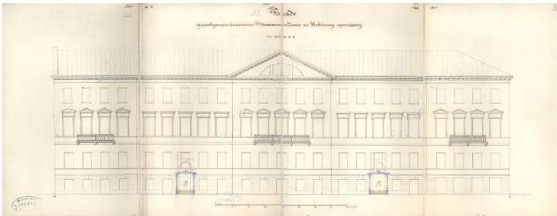
25. Фасад существующего каменного 4-хэтажного дома по Невскому проспекту. 1870 г. // Источник: ЦГИА СПб фонд 513, опись 102, дело 213, листы 32-35. Чертежи дома на участке, принадлежавшем В.И.Струбинскому, А.И.Трейбергу по Невскому пр., 11.
