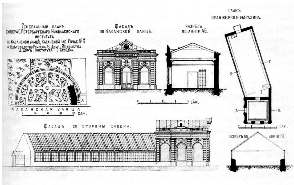
14. Генеральный план сквера С.Петербургского Николаевского института. Сер. XIX в. РГИА Ф. 759. Оп. 95. Д.6. Л. 2. Источник: Архив КГИОП. Фототека. Позитив № 36577/1
