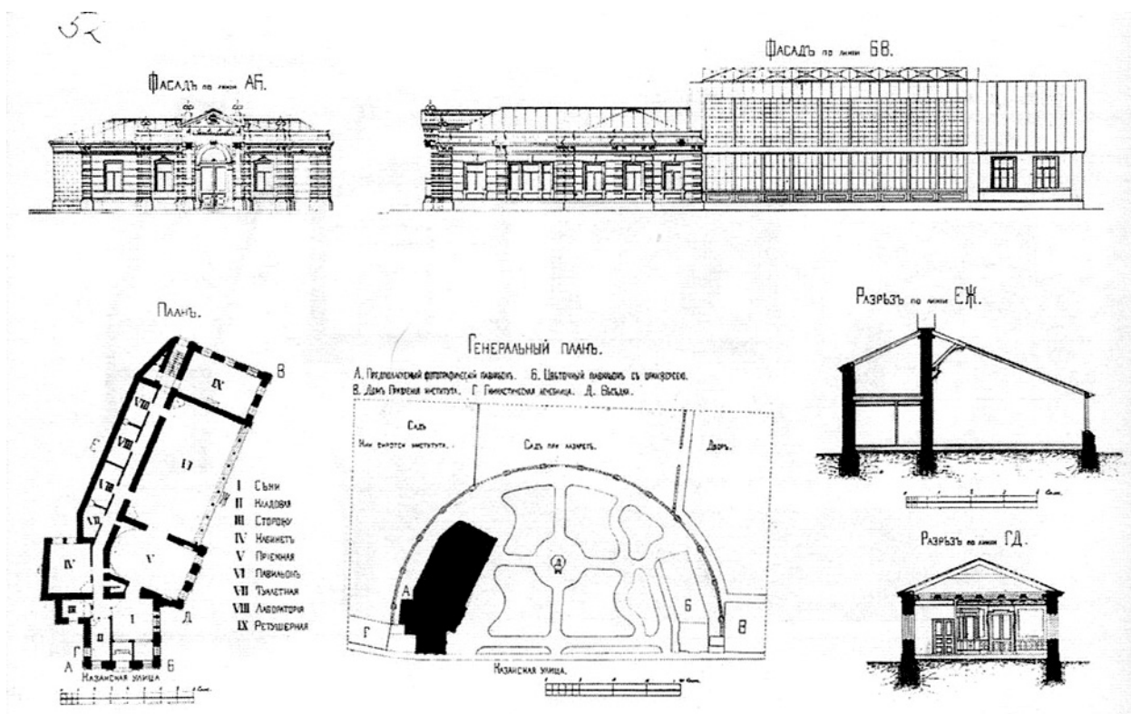
15. Генеральный план сквера С.Петербургского Николаевского института. 16. Сер. XIX в. РГИА Ф. 759. Оп. 95. Д.6. Л. 3. Источник: Архив КГИОП. Фототека. Позитив № 36577/1
