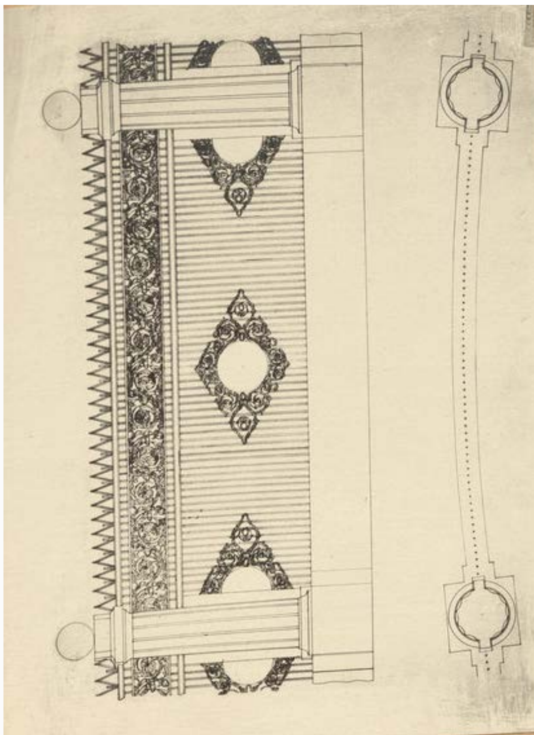
18. Решетка у Казанского собора. Архитектурный обмер. 1920-е гг. Санкт-Петербургское государственное бюджетное учреждение культуры "Государственный музей истории Санкт-Петербурга". Номер по КП (ГИК): ГМИ СПб 46/615. Инвентарный номер: ГМИ СПб Инв.№-I-A-1185/41 фп. Номер в Госкаталоге: 58199606
