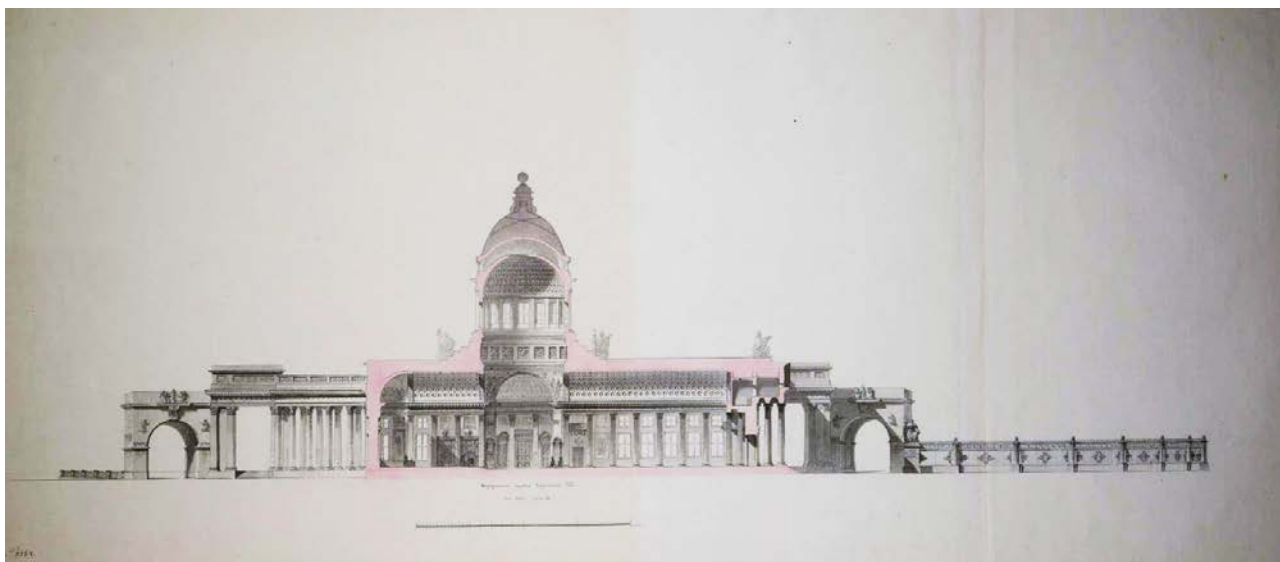
11. Воронихин А.Н. Разрез купола и центральной части Казанского собора. 1810 г. Государственный Эрмитаж. Инвентарный номер: ОР-9254. Источник:
