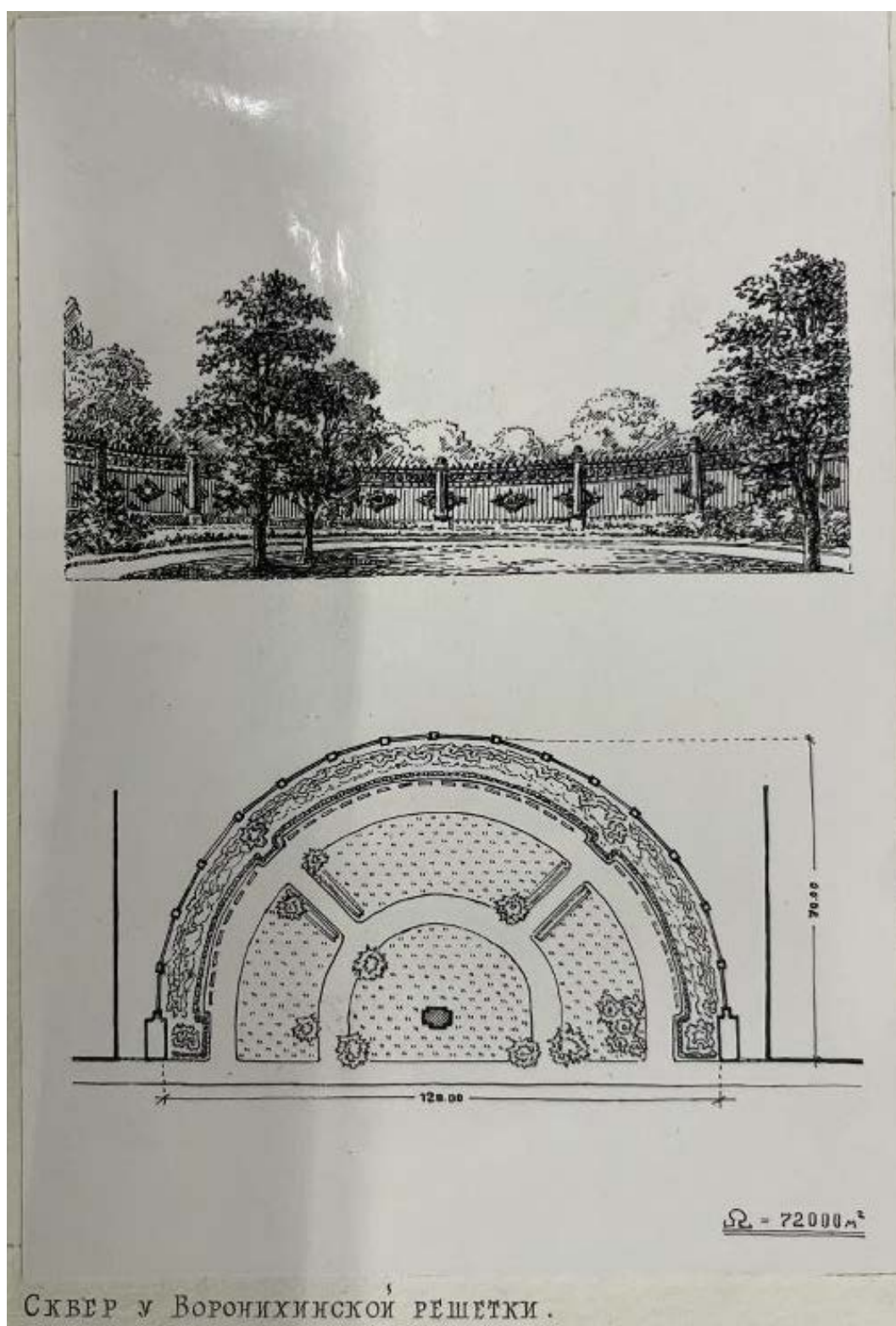
20. Сквер у Воронихинской решетки. Санкт-Петербург. План и развертка. Из комплекта планшетов «Озеленение города Москвы. Архитектура скверов и бульваров» к кандидатской диссертации М.И. Прохоровой «Скверы и бульвары г. Москвы — планировка и композиция» 1955 г. 1940 - середина 1950-х гг.
