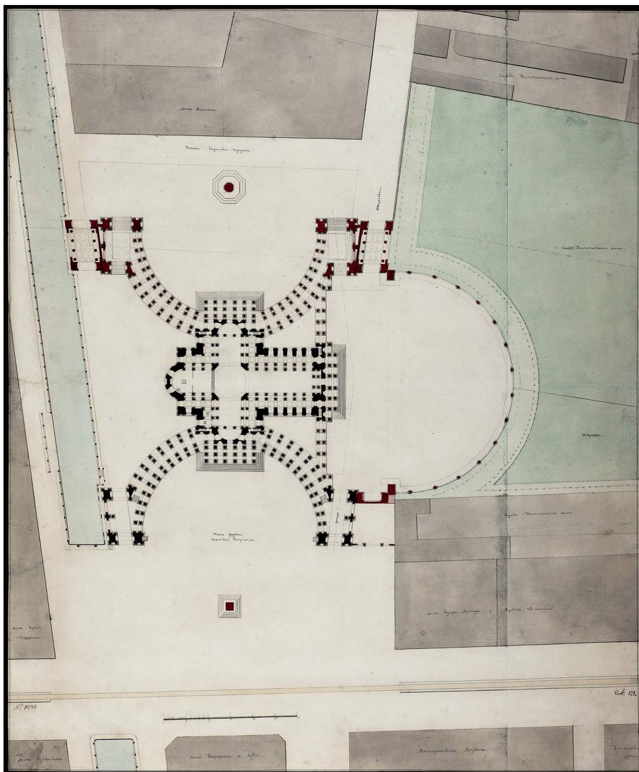
10. А. Н. Воронихин. Проект Казанского собора. План. 1810 г. Государственный Эрмитаж . Инвентарный номер: ОР-9249. Коллекция онлайн: сайт.
