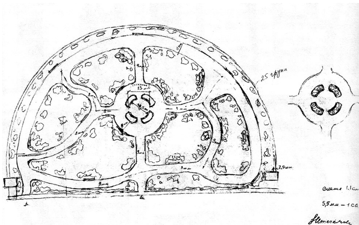
13. Проектный план сквера в ограде Воронихинской решётки перед западным фасадом собора. 1865. Г.Х.Штегеман, И.Альвардт. Веснина Н.Н. Сады Невского проспекта. 2008.- С. 86
