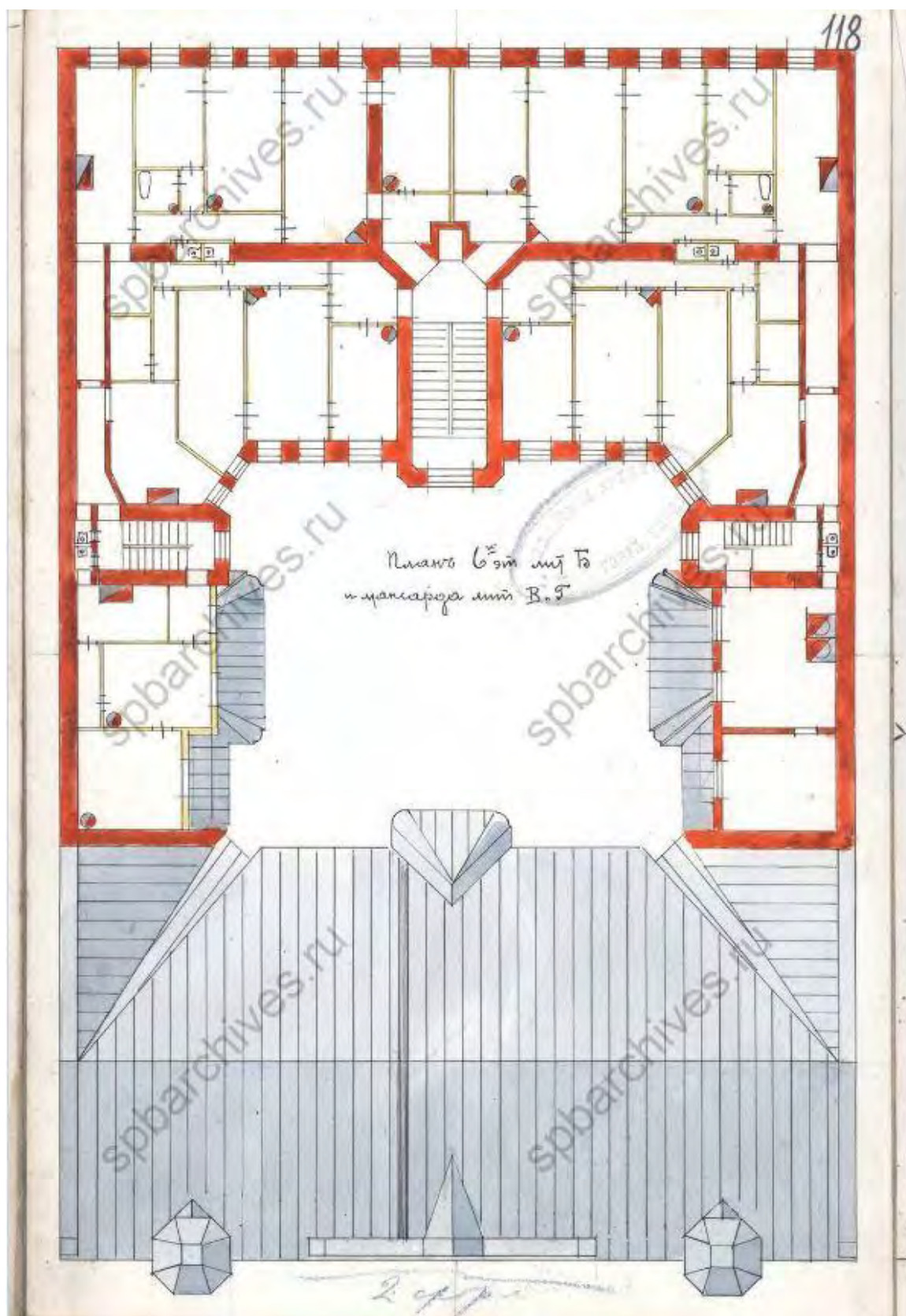
Илл. 30. План 6-го этажа лит. Б и мансарда лит. В, Г. 1905 г. Гражданский инженер М. Капелинский.
