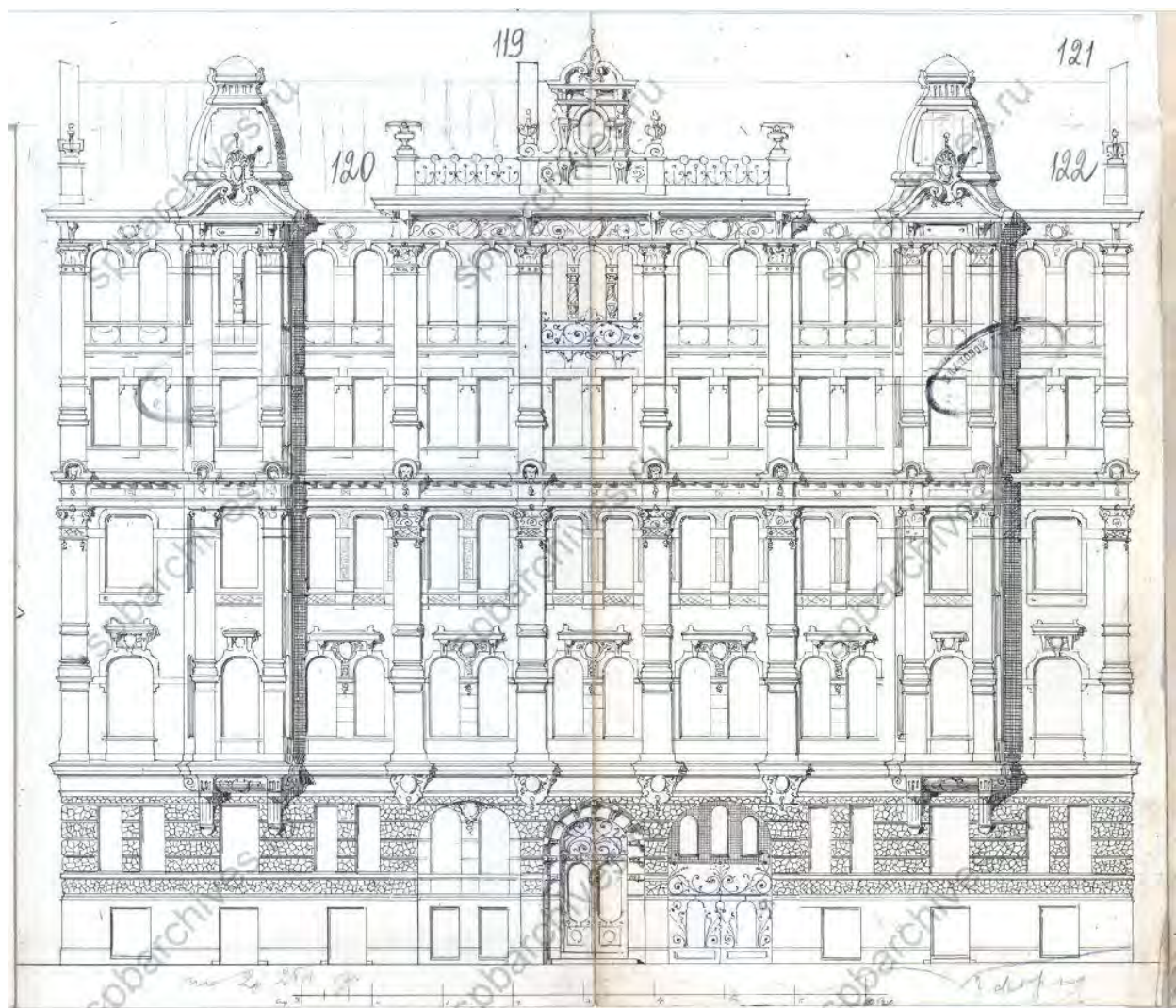
Илл. 31. Лицевой фасад. 1905 г. Гражданский инженер М. Капелинский. ЦГИА СПб. Ф. 513. Оп. 102. Д. 4306. Л. 119 – 122.
