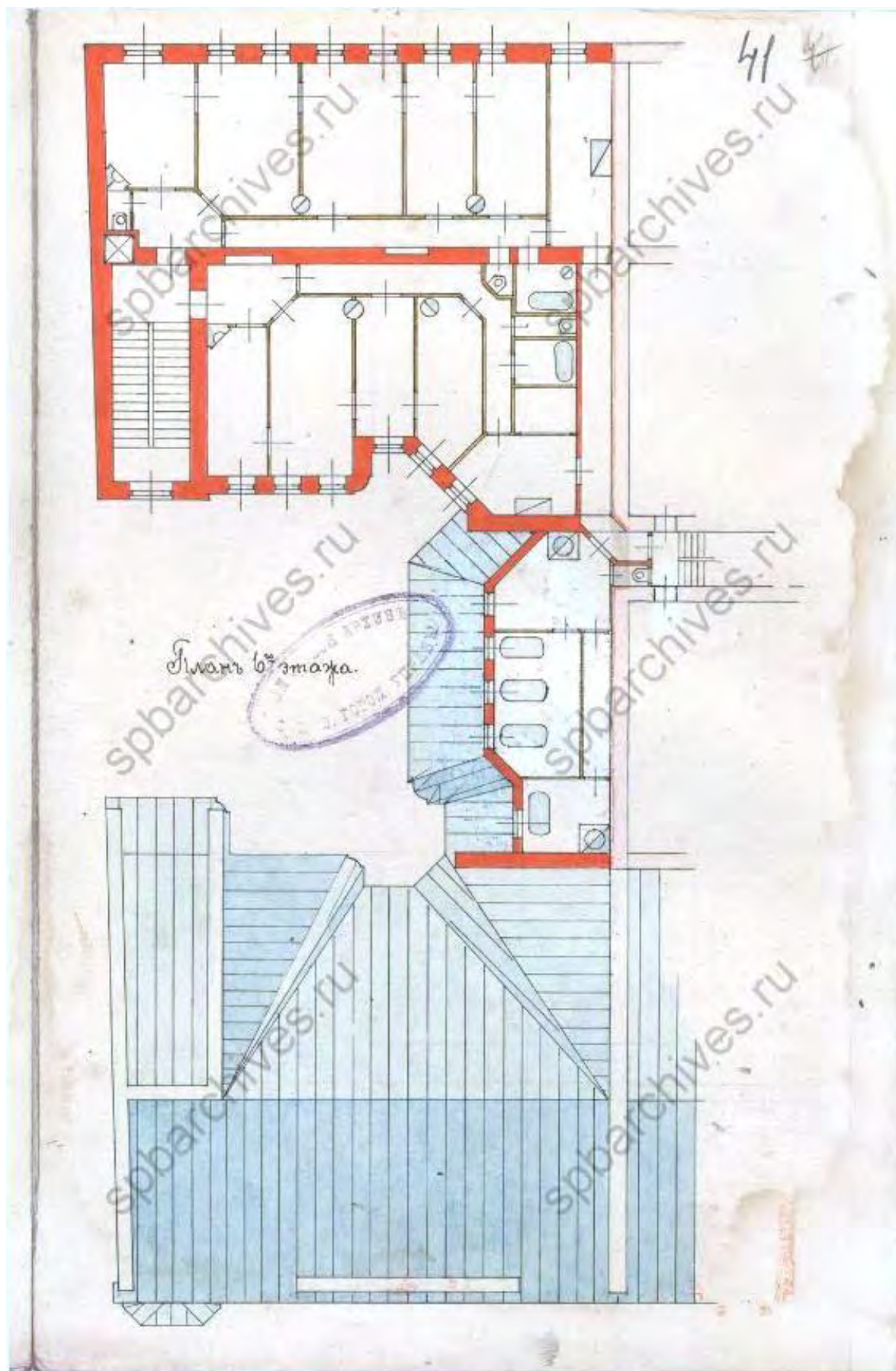
Илл. 35. План 6-го этажа. 1908 г. ЦГИА СПб. Ф. 513. Оп. 102. Д. 4306. Л. 41.
