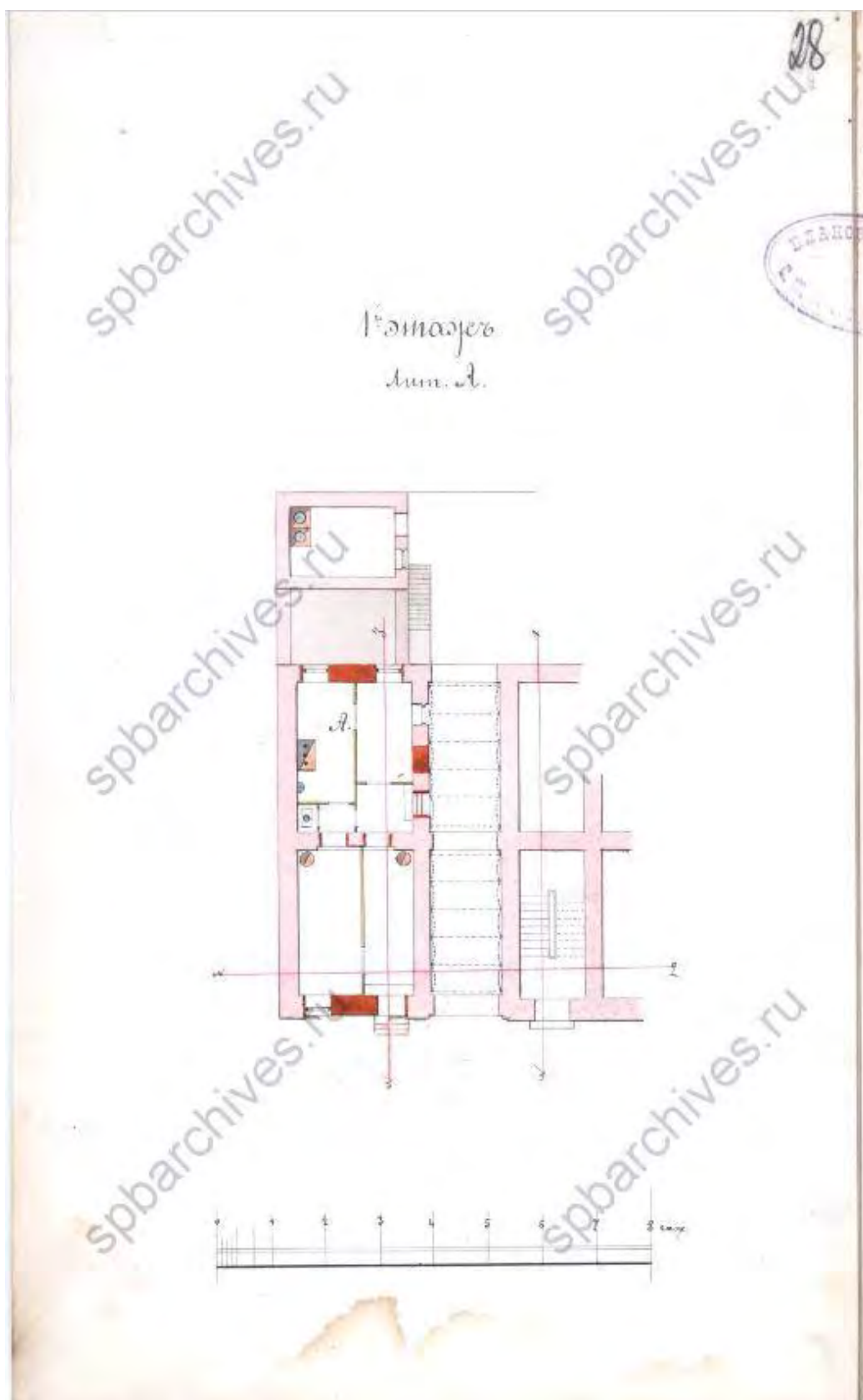
Илл. 23. 1-й этаж. 1898 г. ЦГИА СПб. Ф. 513. Оп. 102. Д. 4306. Л. 28.
