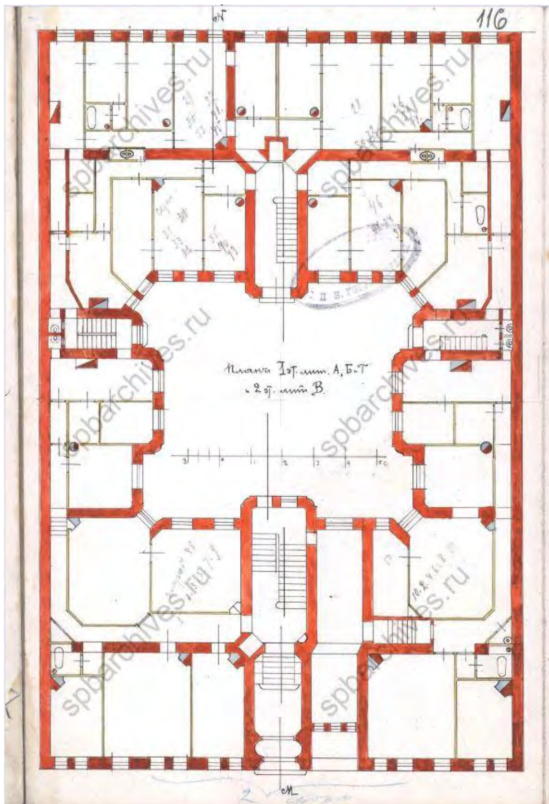
Илл. 28. План 1-го этажа лит. А, Б, Г и 2-й этаж лит. В. 1905 г. Гражданский инженер М. Капелинский.
