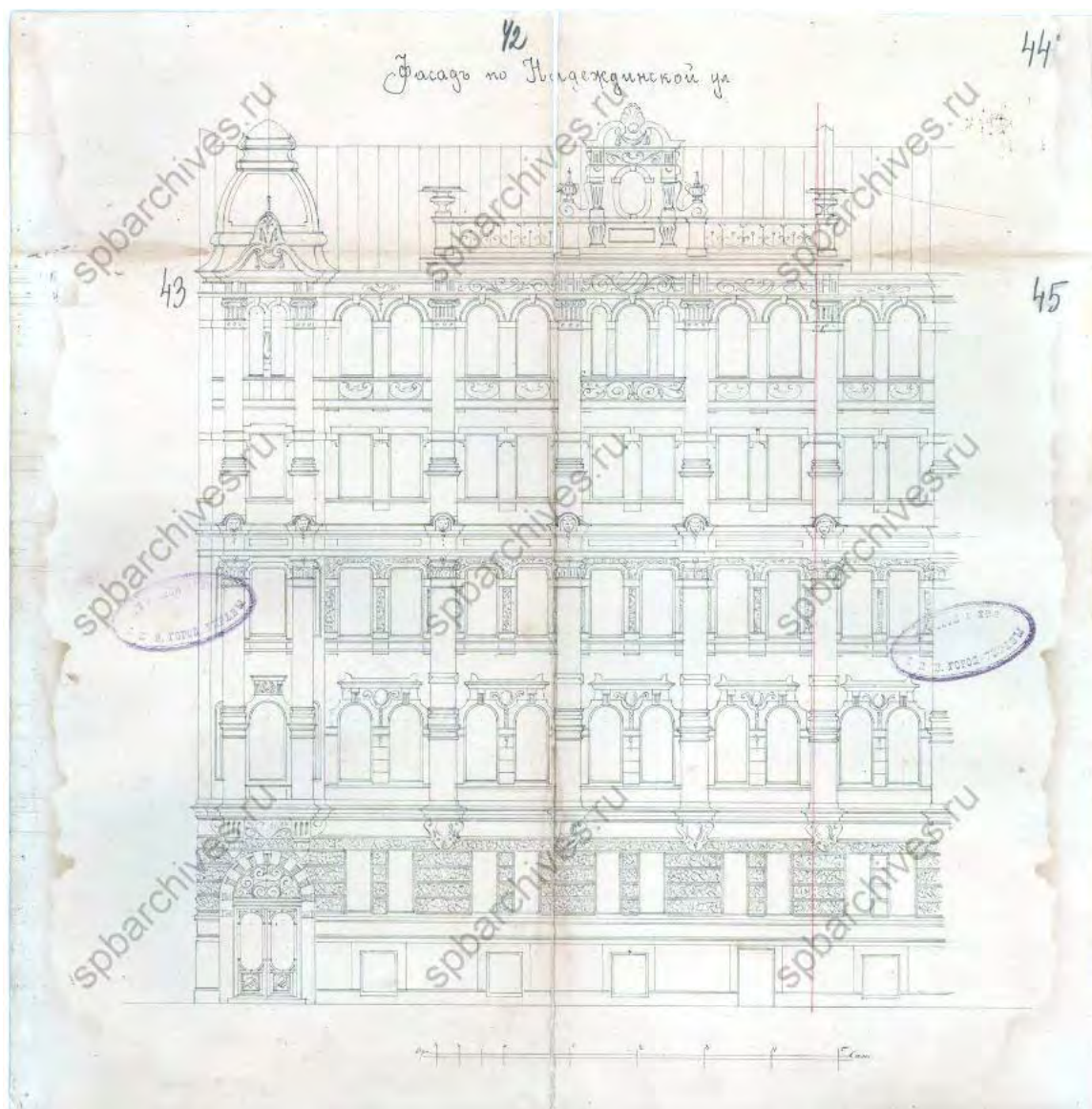
Илл. 36. Фасад по Надеждинской улице. 1908 г. ЦГИА СПб. Ф. 513. Оп. 102. Д. 4306. Л. 42 – 45.
