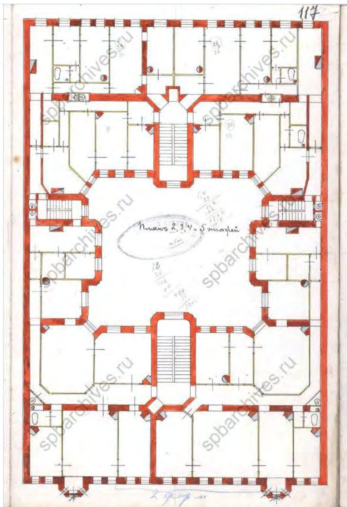
Илл. 29. План 2, 3, 4 и 5-го этажей. 1905 г. Гражданский инженер М. Капелинский. ЦГИА СПб. Ф. 513. Оп. 102. Д. 4306. Л. 117.
