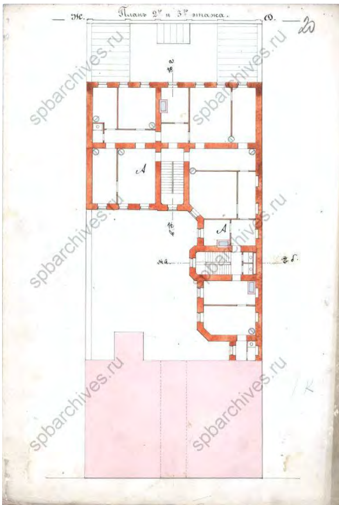
Илл. 19. План 2-го и 3-го этажа. 1873 г. Арх. Ф.И. Шустер. ЦГИА СПб. Ф. 513. Оп. 102. Д. 4306. Л. 20.
