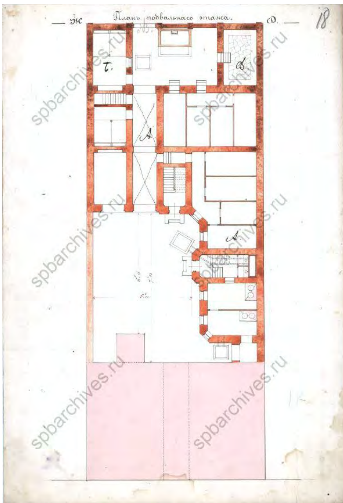
Илл. 17. План подвального этажа. 1873 г. Арх. Ф.И. Шустер. ЦГИА СПб. Ф. 513. Оп. 102. Д. 4306. Л. 18.
