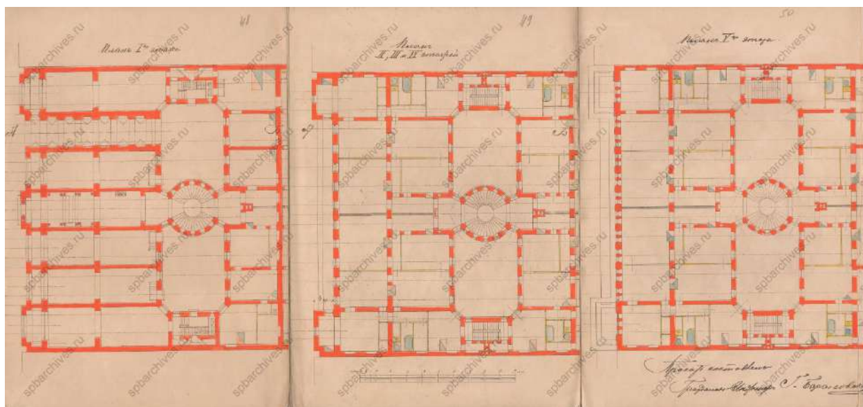
Илл. 8. Проектный план 1-го, 2-го, 3-го и 4-го, 5-го этажей. 1891 г. (источник: ЦГИА СПб. Ф. 513. Оп. 102. Д. 5358)
