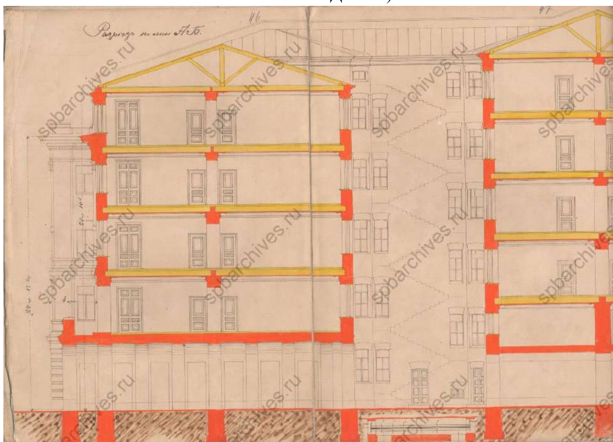
Илл. 11. Проектный разрез по А-Б. 1891 г. (источник: ЦГИА СПб. Ф. 513. Оп. 102. Д. 5358).
