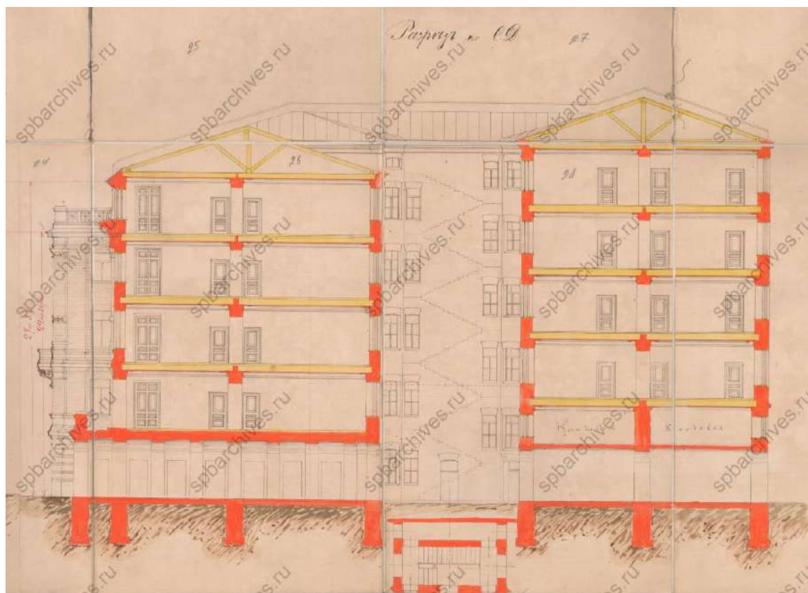
Илл. 12. Проектный разрез по С-Д. 1891 г. (источник: ЦГИА СПб. Ф. 513. Оп. 102. Д. 5358).
