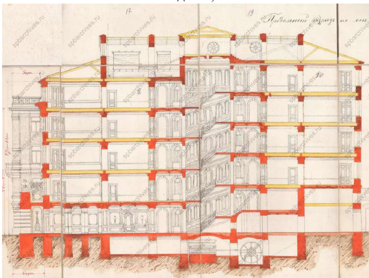
Илл. 13. Продольный разрез по оси. 1891 г. (источник: ЦГИА СПб. Ф. 513. Оп. 102. Д. 5358).
