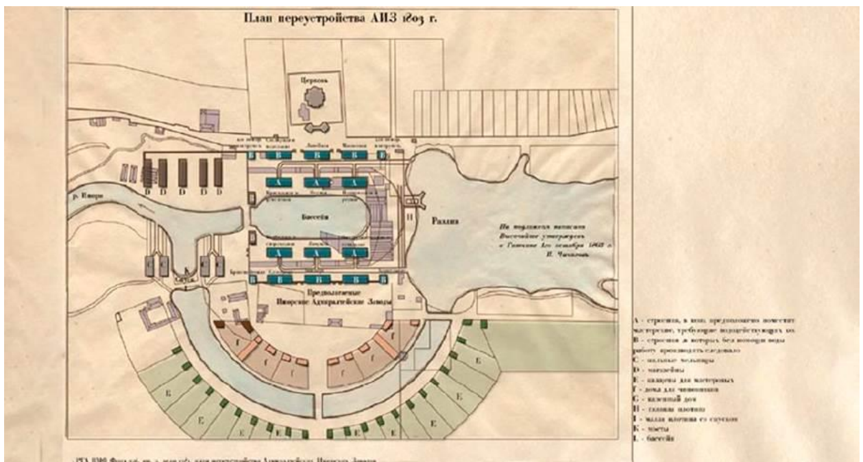
Илл. 4. План переустройства Ижорских заводов, утвержденный 1 октября 1803 г.
