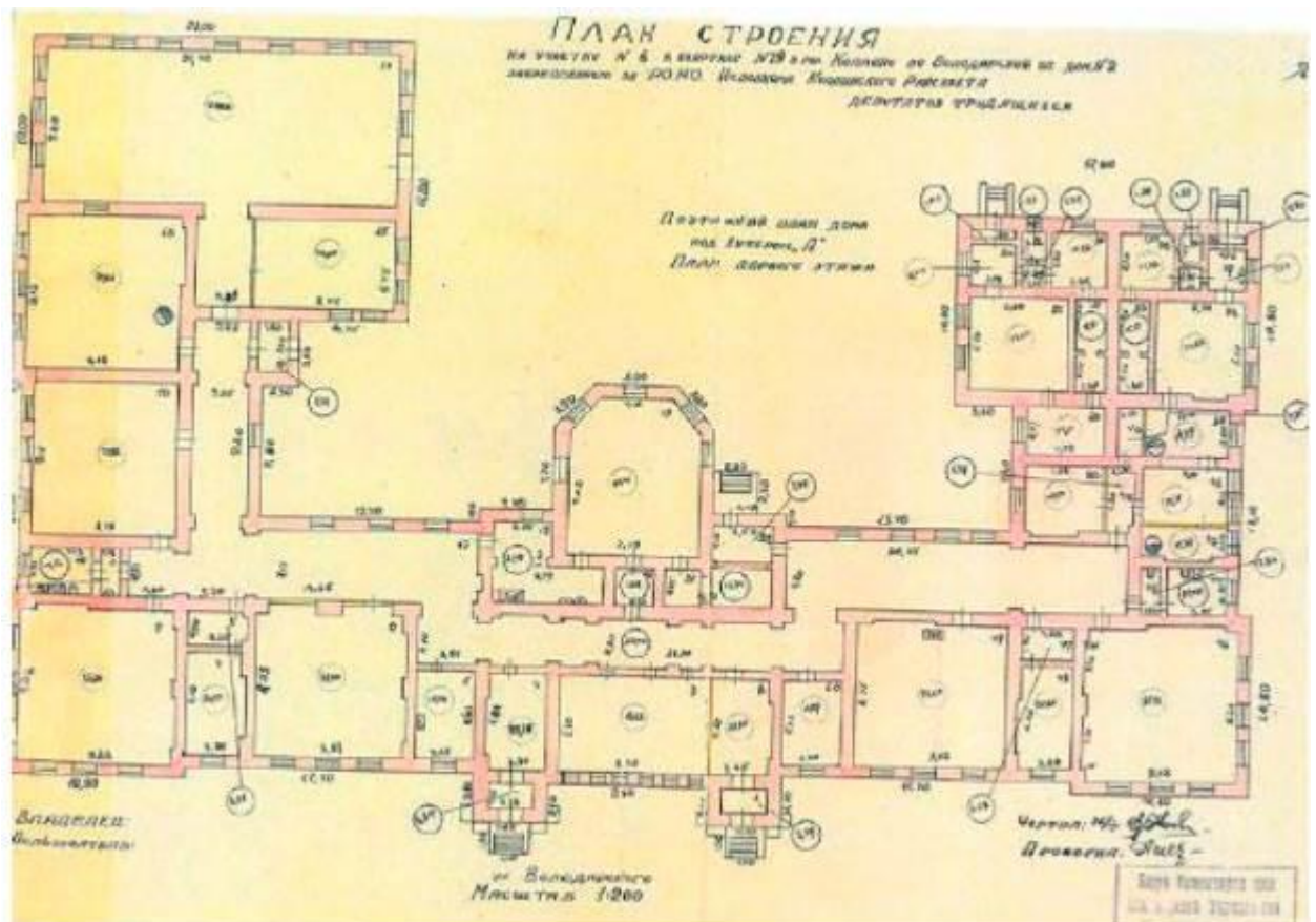
Илл.22. Колпино. Быв. школа Адмиралтейских Ижорских заводов. План здания. 1948 год. Архив ПИБ. № 14, 01КЛ-198.
