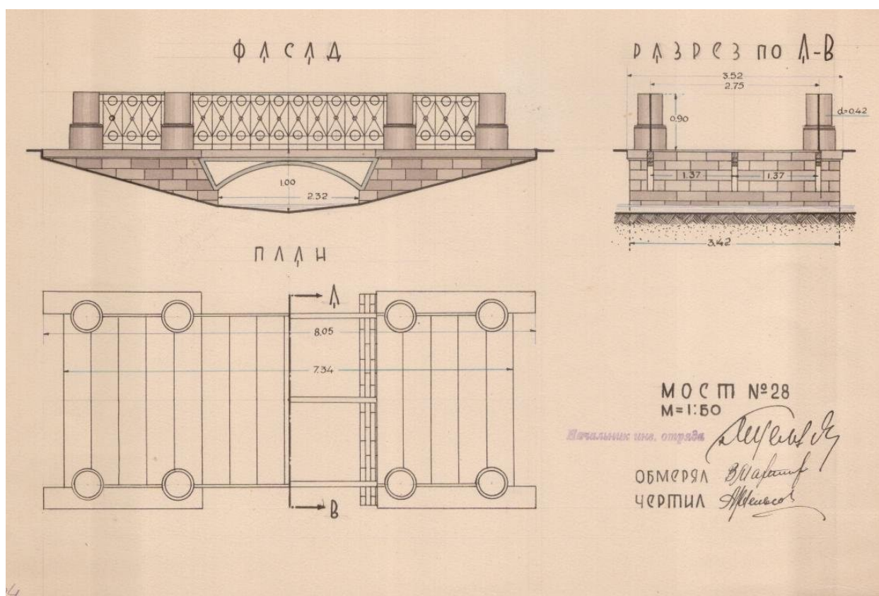
9. Мост № 28. Фасад, план, разрез. 1935. Госкаталог. Инв. № ЕД-3875-ХIII.
