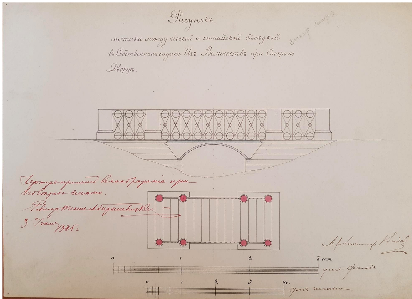
7. Рисунок мостика между киоском и китайской беседкой. Архитектор Видов А.Ф. 1895. Госкаталог. Инв. № ЕД-956-ХІІІ.
