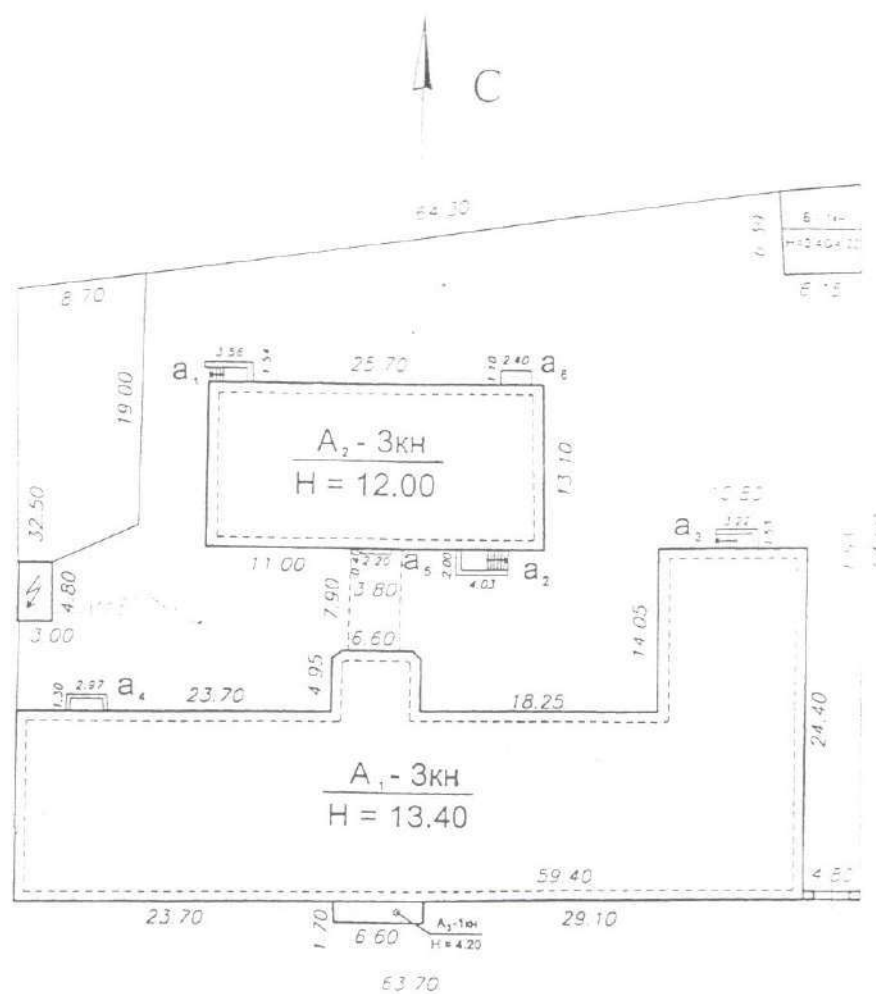
План земельного участка
