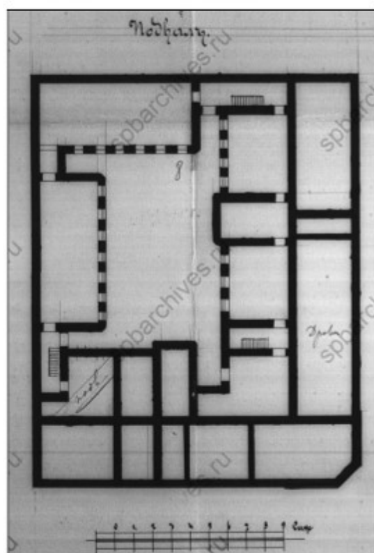
31. План подвала. 1910 г. ЛЛ. 7-10.
