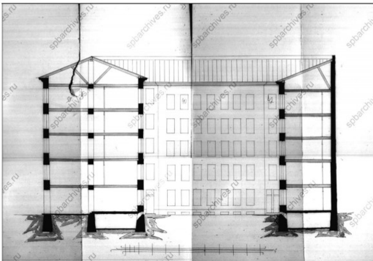
38. Разрез. 1910 г. Ф. 515. Оп. 4. Д. 2122. ЛЛ. 37-44.
