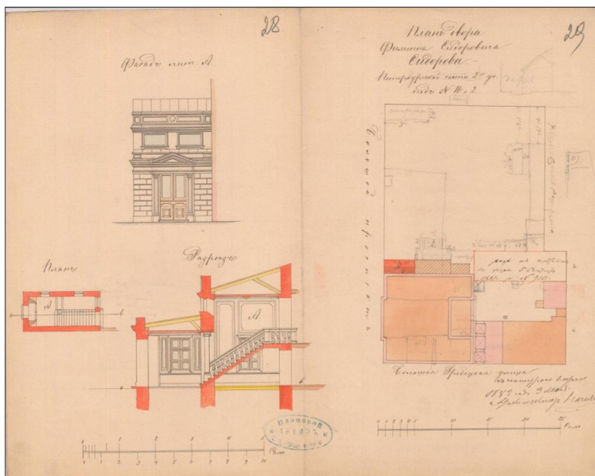
13. План двора Филиппа Сидоровича Сидорова Петербургской части 2го участка по Большому проспекту и Большой Гребенцкой улице под №№16 и 2 с показом существующих и строящихся корпусов 1882 г. Ф. 513. Оп. 102. Д. 7292. ЛЛ. 28, 29.
