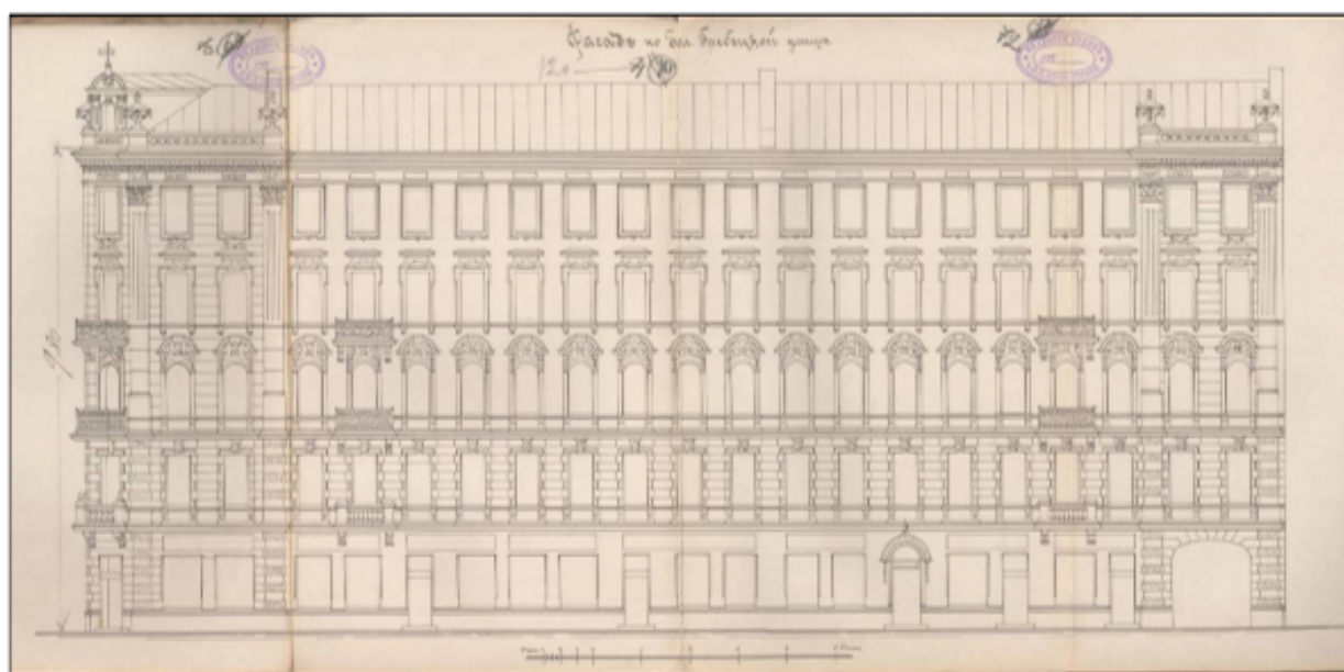
21. Лицевой фасад по Большой Гребенцовой улице [совр. Пионерская ул.]. 1913 г. Ф. 513. Оп. 102. Д. 7292. ЛЛ. 70-73.
