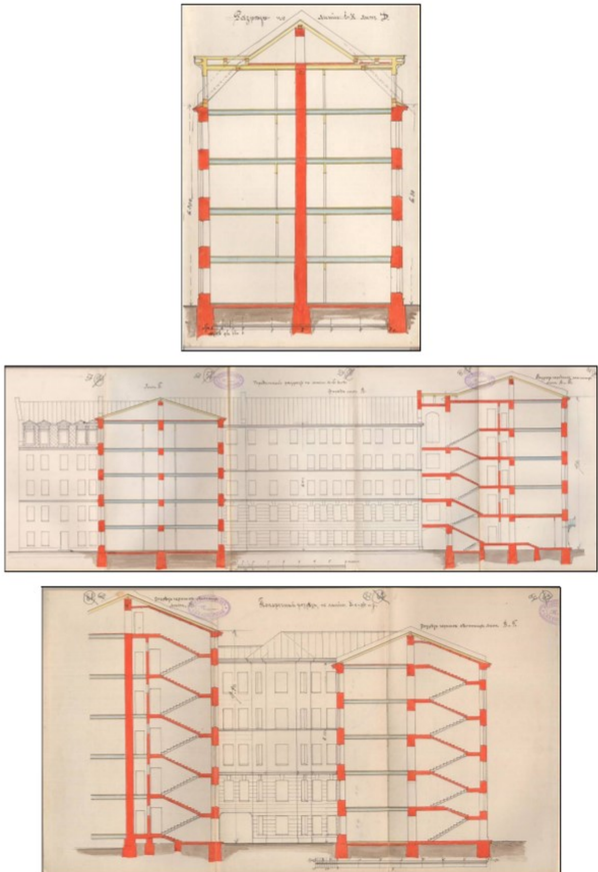
19. Разрезы поперечные и продольные, разрезы лестниц, фасад. 1913 г. Ф. 513. Оп. 102. Д. 7292. ЛЛ. 56-64.
