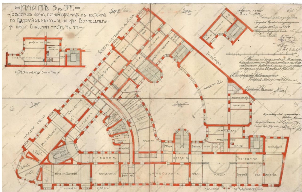
9. План 3-го этажа Городского дома. 22.02.1905. Проект арх. Лишневского. ЦГИА СПб. Ф.503. Оп.101. Д.587. Л.66-67
