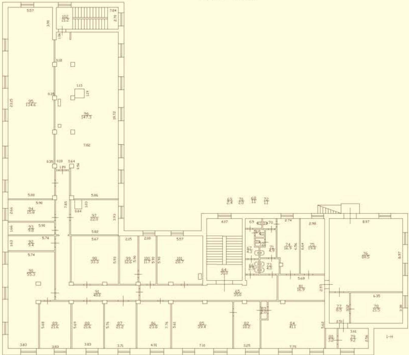
План 2 этажа
