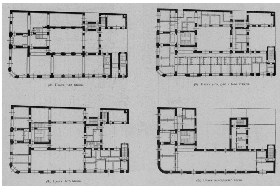
14. Планы 1-го, 2-го, 4-го, 5-го, 6-го и мансардного этажей. 1904 г. Опубликовано в: Строитель. Вестник архитектуры, домовладения и санитарного зодчества. / Редактор-издатель гражданский инженер Г.В. Барановский. – Десятый год издания. – № 17-20. СПб.: Фонтанка, 66. 1904. С. 661 – 662.
