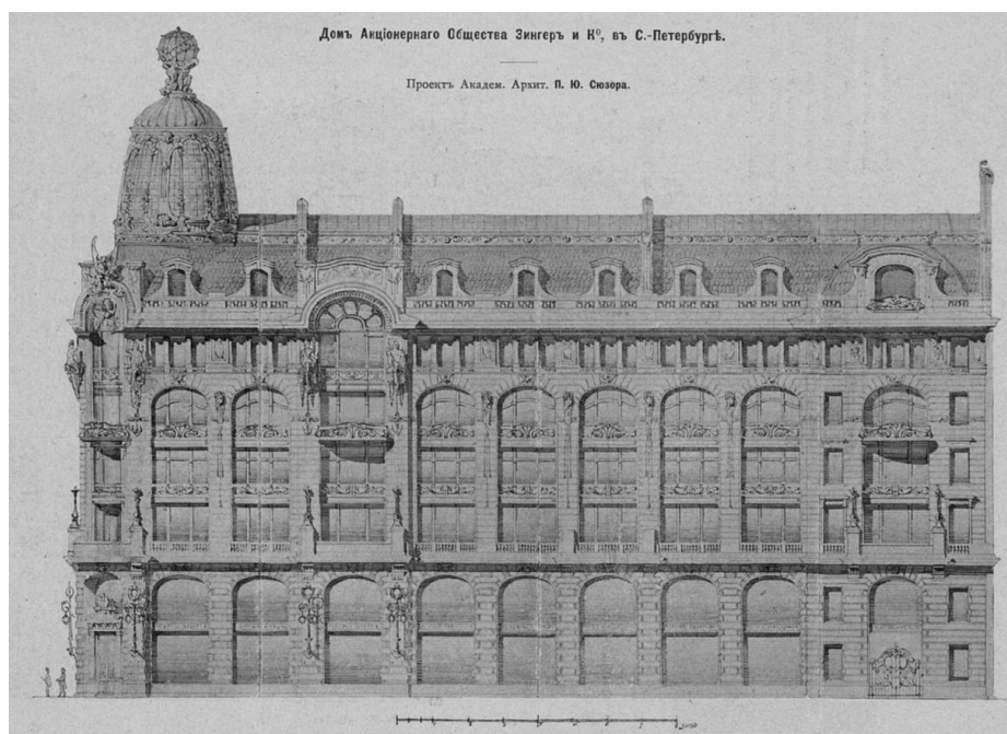
13. Фасад по наб. Екатерининского канала (утвержденный проект). 1904 г. Опубликовано в: Строитель. Вестник архитектуры, домовладения и санитарного зодчества. / Редактор-издатель гражданский инженер Г.В. Барановский. – Десятый год издания. – № 17- 20. СПб.: Фонтанка, 66. 1904. С. 659 – 660.
