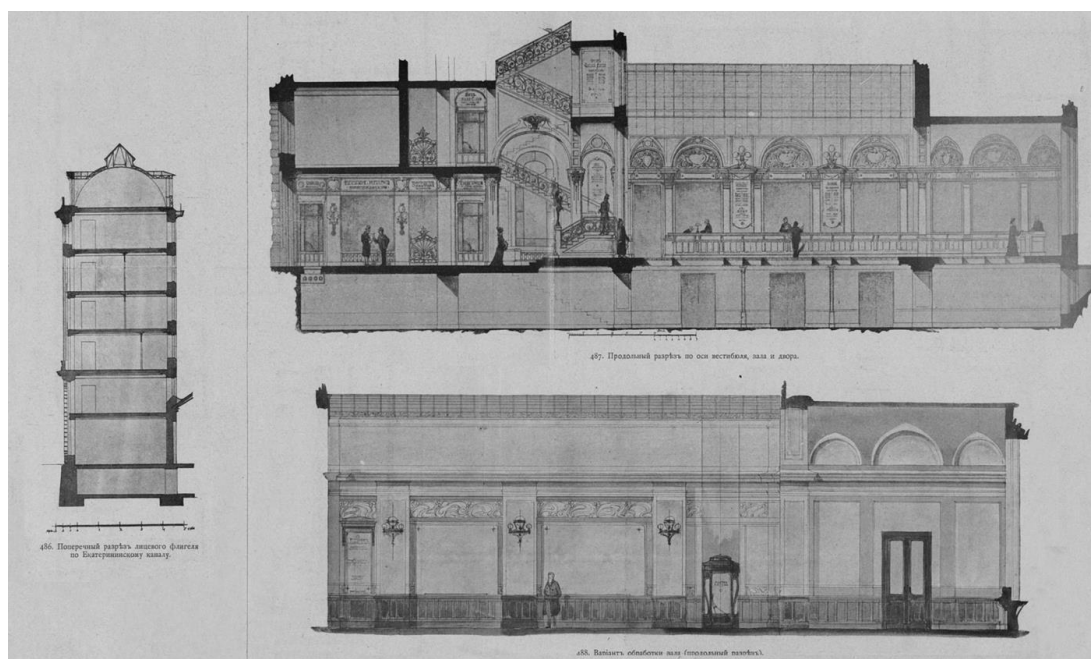
15. Поперечный разрез лицевого флигеля по Екатерининскому каналу, продольный разрез по оси вестибюля, зала и двора и вариант обработки зала (продольный разрез). 1904 г. Опубликовано в: Строитель. Вестник архитектуры, домовладения и санитарного зодчества. / Редактор-издатель гражданский инженер Г.В. Барановский. – Десятый год издания. – № 17-20. СПб.: Фонтанка, 66. 1904. С. 663 – 666.
