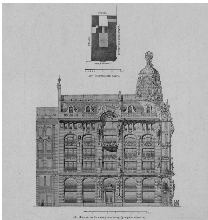
12. Генеральный план и фасад по Невскому проспекту (утвержденный проект). 1904 г. Опубликовано в: Строитель. Вестник архитектуры, домовладения и санитарного зодчества. / Редактор-издатель гражданский инженер Г.В. Барановский. – Десятый год издания. – № 17-20. СПб.: Фонтанка, 66. 1904. С. 657 – 658.
