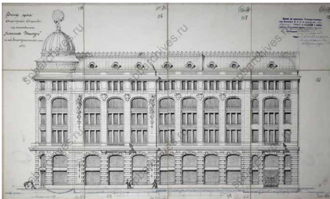
9. Фасад дома Акционерного общества под наименованием «Компания Зингер» по набережной Екатерининского канала, № 21. 1902 г. ЦГИА СПб. Ф. 513. Оп. 102 Д. 3423. Лл. 114 – 121.
