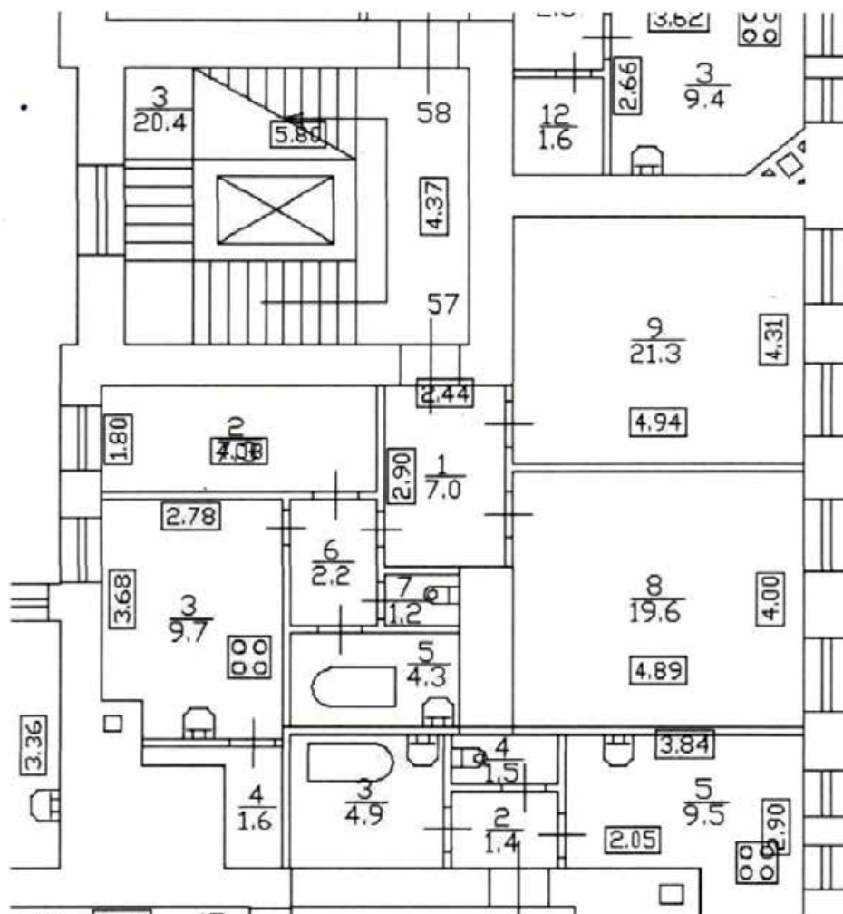
План части 2 этажа. М.1:200 h = 3.15
