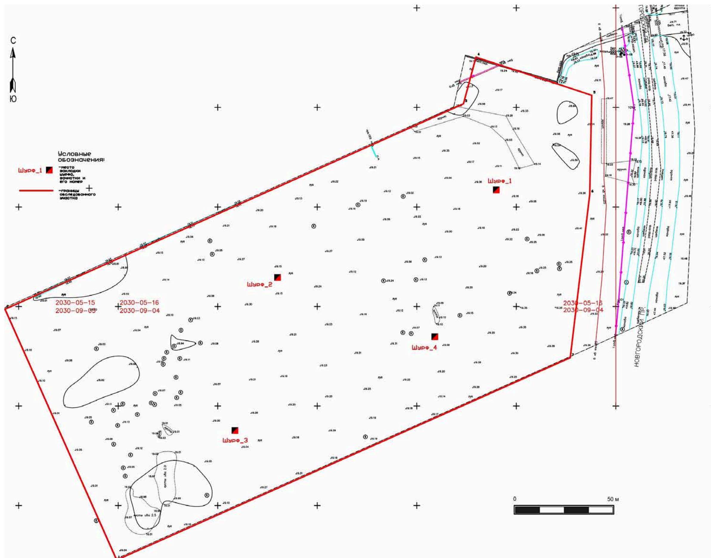
Рис. 17. Санкт-Петербург, пос. Шушары, ул. Школьная, ЗУ 30 (дом 181, литера А по Школьной улице), земельный участок с кадастровым номером: 78:42:0015104:4812. Местоположение шурфа и зачистки на топографической основе, предоставленной заказчиком.
