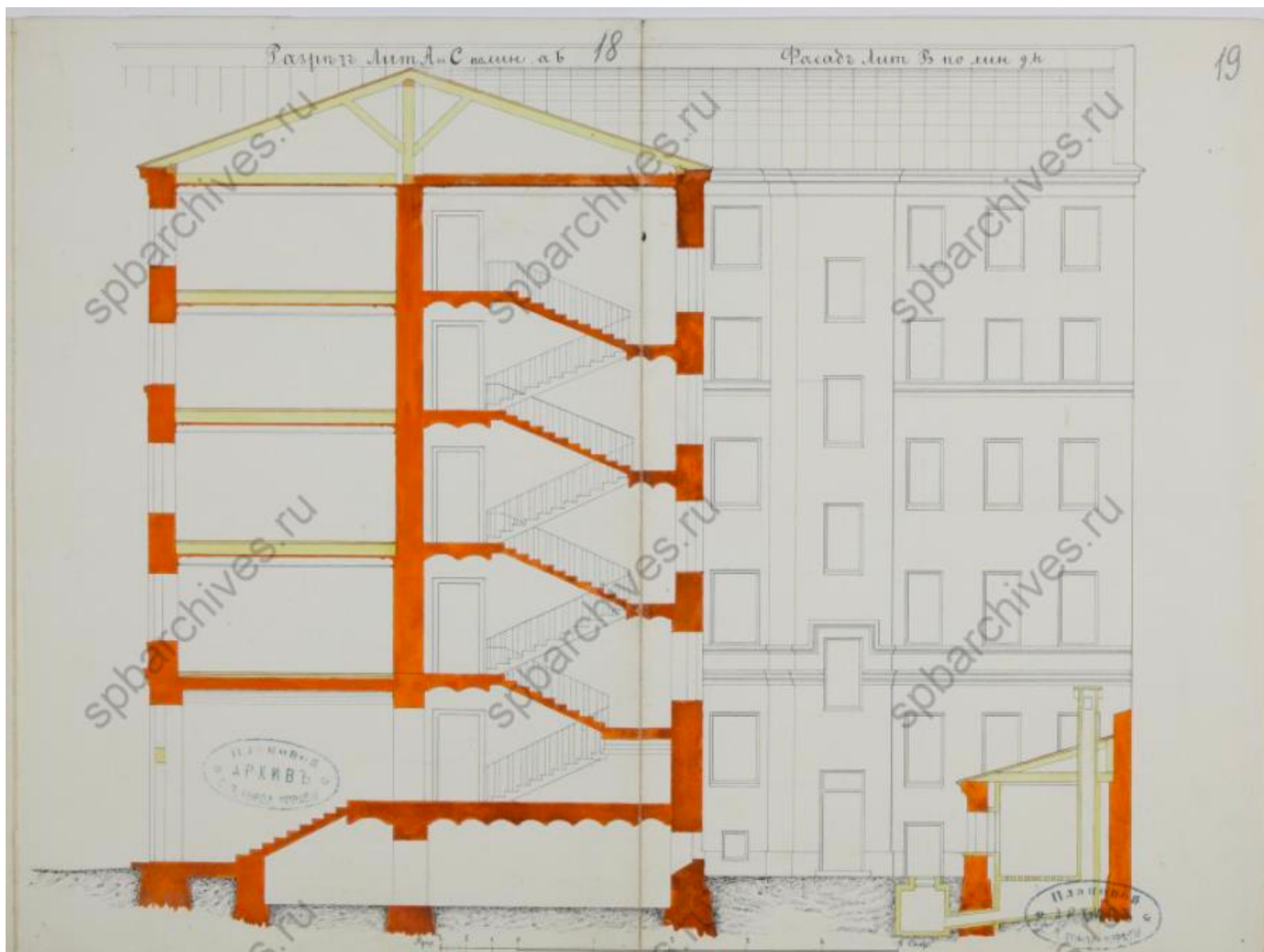
14. Разрез Лит. А и С по лин. а в. Фасад Лит. В по лин. г в. ЦГИА СПб. Ф. 513. Оп. 102. Д. 4580. Лл. 18-19.
