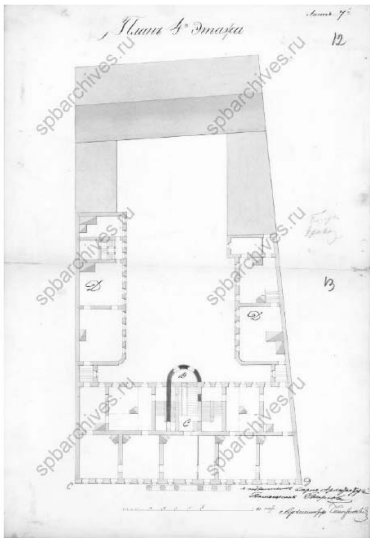
Илл. 10. Проектный план 4-го этажа. 1855 г. (источник: ЦГИА СПб. Ф. 513. Оп. 102. Д. 4558).
