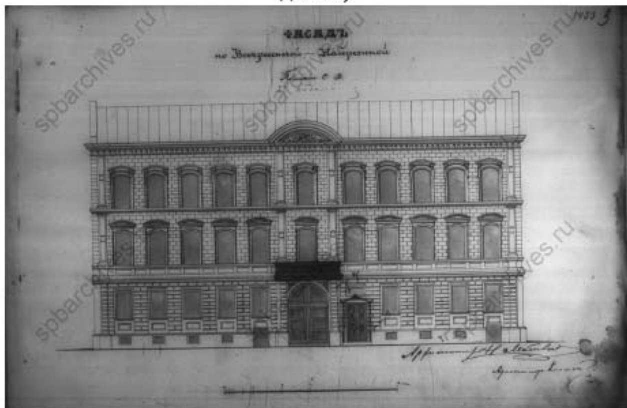
Илл. 19. Фасад по Воскресенской набережной. 1866 г. (источник: ЦГИА СПб. Ф. 515 Оп. 4. Д. 394-1).
