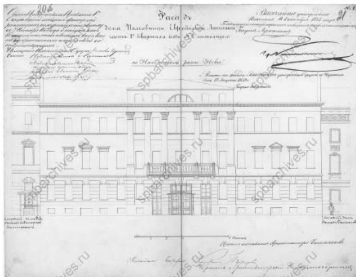
Илл. 15. Фасад дома Полковницы Еврейновой Литейной части 1-го квартала под № 15/7 по набережной реки Невы. 1855 г. (источник: ЦГИА СПб. Ф. 513. Оп. 102. Д. 4558).
