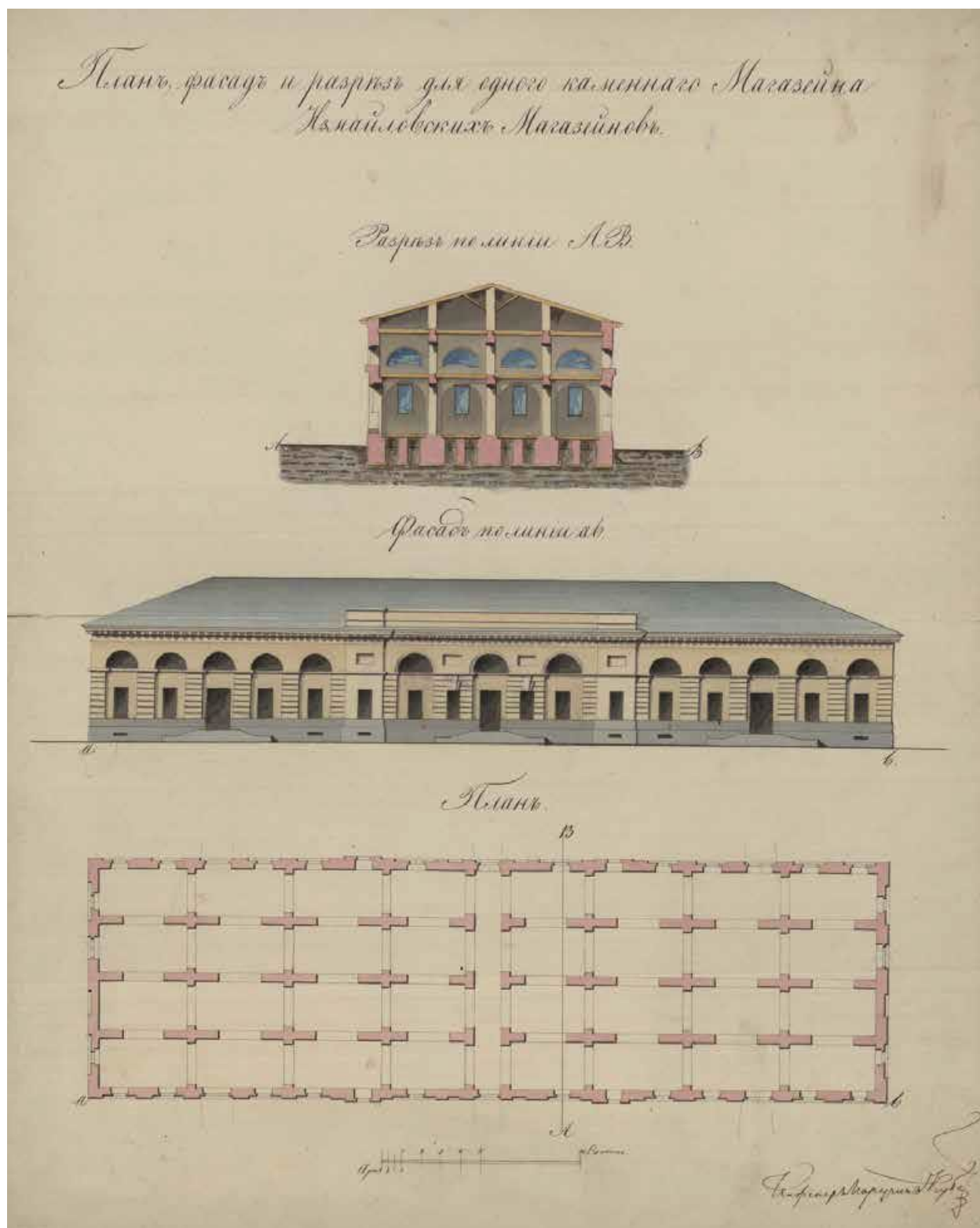
17. План, фасад и разрез одного каменного магазина Измайловских магазинов. 1836 г. // РГА ВМФ. Ф. 3Л. Оп. 36. Д. 8894. Л. 1.
