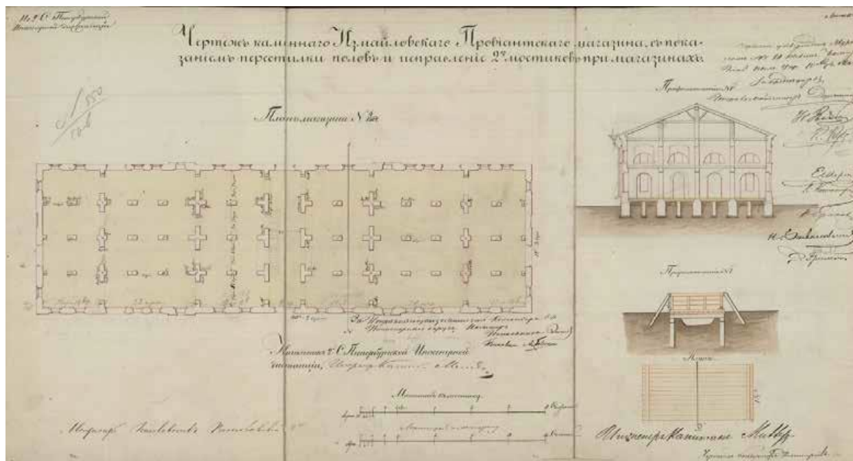
19. Чертеж каменного Измайловского провиантского магазина с показанием перестилки полов и исправления двух мостиков при магазинах. 1864 г. // РГА ВМФ. Ф. 3Л. Оп. 36. Д. 8945. Л. 1.
