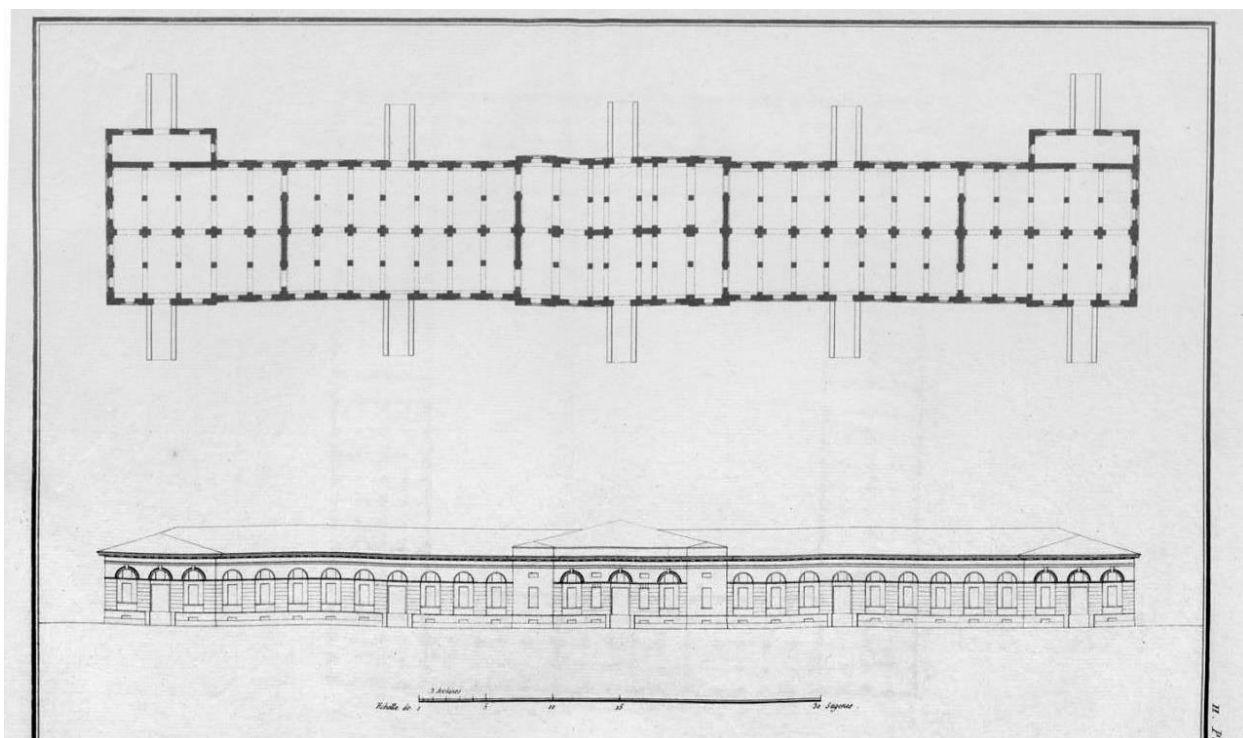
15. Фасад и план Троицкого провиантского магазина. Арх. Л. Руска. 1800-е гг. // https://p1.citywalls.ru/photo_355-364329.jpg?mt=1538673769
