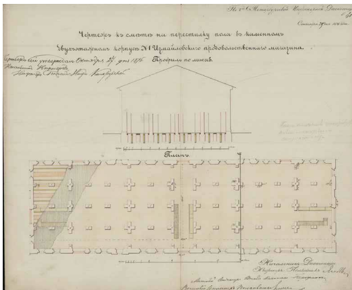
20. Чертеж к смете на перестилку пола в каменном двухэтажном корпусе № 1 Измайловского продовольственного магазина. 1876 г. // РГА ВМФ. Ф. 3Л. Оп. 36. Д. 8972. Л. 1.
