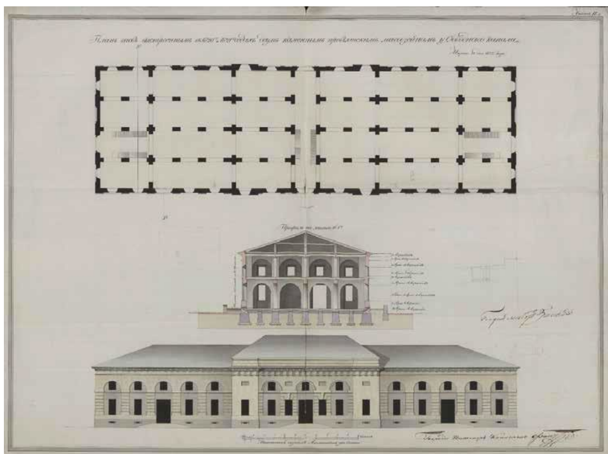
16. План, фасад и профиль вновь выстроенным двум каменным провиантским магазинам у Обводного канала. 1822 г. // РГА ВМФ. Ф. 3Л. Оп. 36. Д. 8868. Л. 1.
