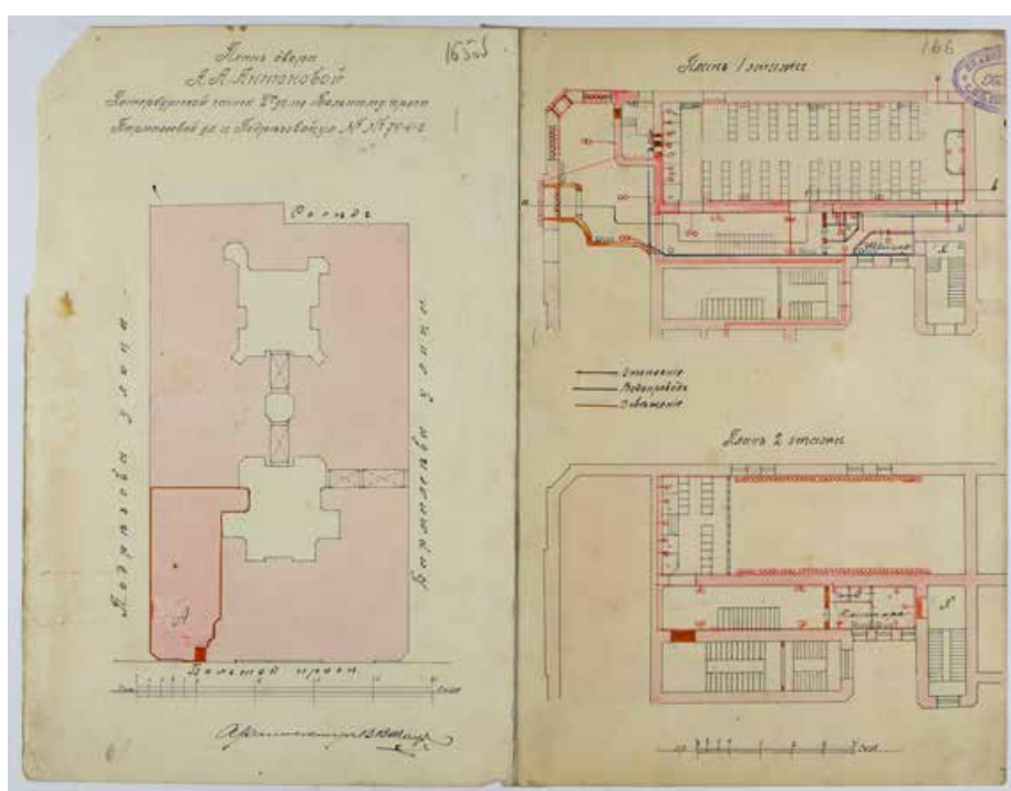
18. Постановление. План двора Антоновой Анастасии Александровны. Фрагменты поэтических планов. Проект устройства кинематографа (арх. В. Шауб). Утверждено 1 февраля 1913 г (не осуществлено, в дальнейшем осуществлено по проекту, утверждённому 12 января, 10 ноября 1915 г.). ЦГИА СПб. Ф. 513. Оп. 102. Д. 7348. ЛЛ. 165-166.
