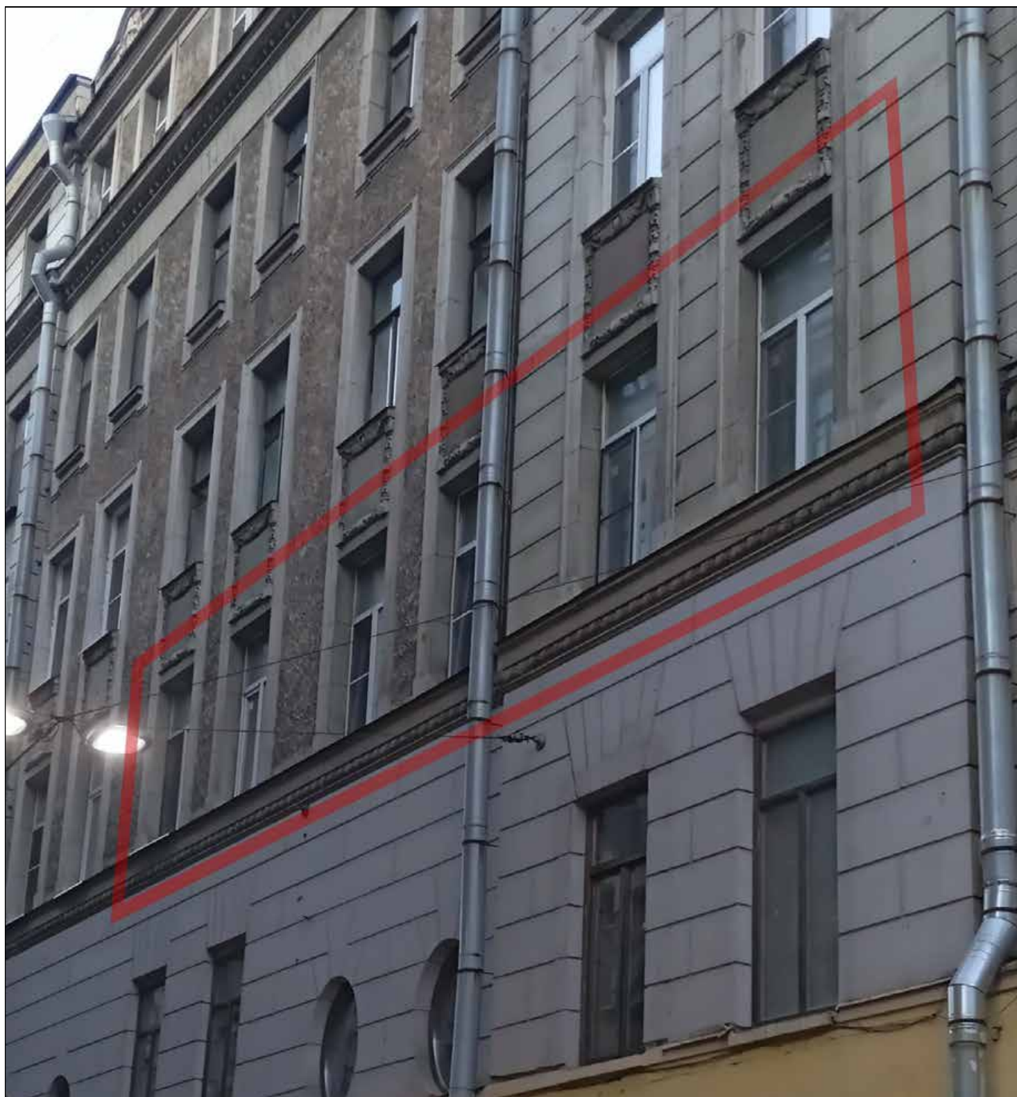
4. Лицевой фасад лицевого корпуса по Подрезова улице. Фрагмент. Окна кв. № 3.
