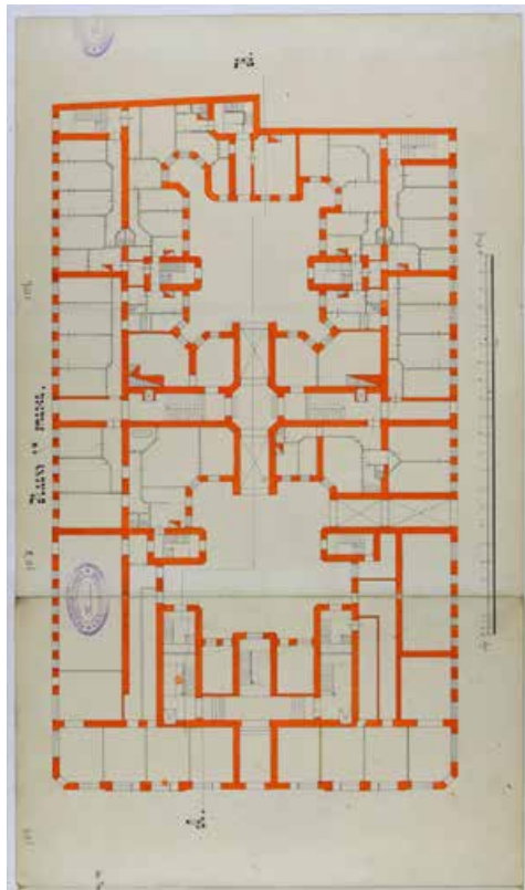
16. Постановление. План двора Антоновой Анастасии Александровны. Фасад. Поэтажные планы. Проект постройки шестизэтажных с мансардой лицевых домов по Большому пр., Бармалеевой и Подрезова ул. и флигелей. Утверждено 15 июня 1912 г., осуществлено по проекту, подписанному архитектором В.Шаубом 5 декабря 1913 г. ЦГИА СПб. Ф. 513. Оп. 102. Д. 7348. ЛЛ. 105-133.
