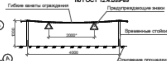
Конструкция сигнального ограждения по ГОСТ 12.4.059-89
